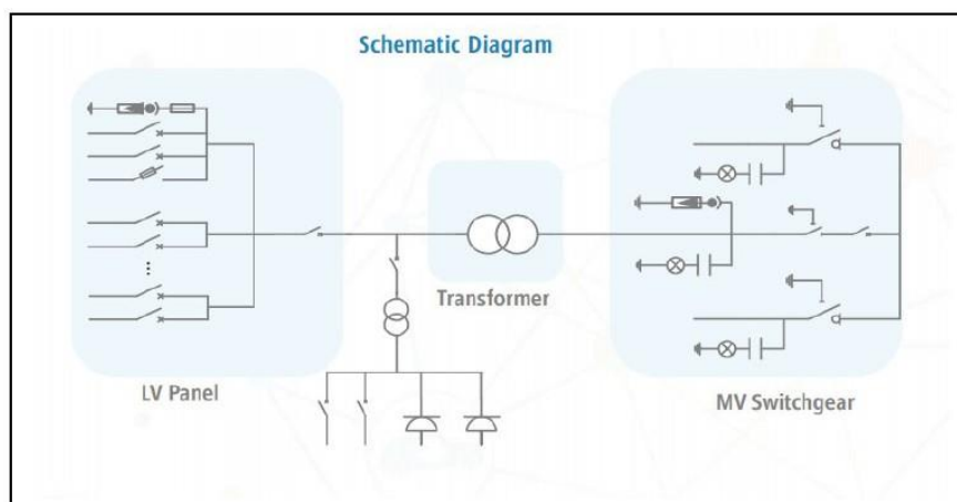
FIGURA 6: SCHEMA DI POSSIBILE COLLEGAMENTO E PROTEZIONE
