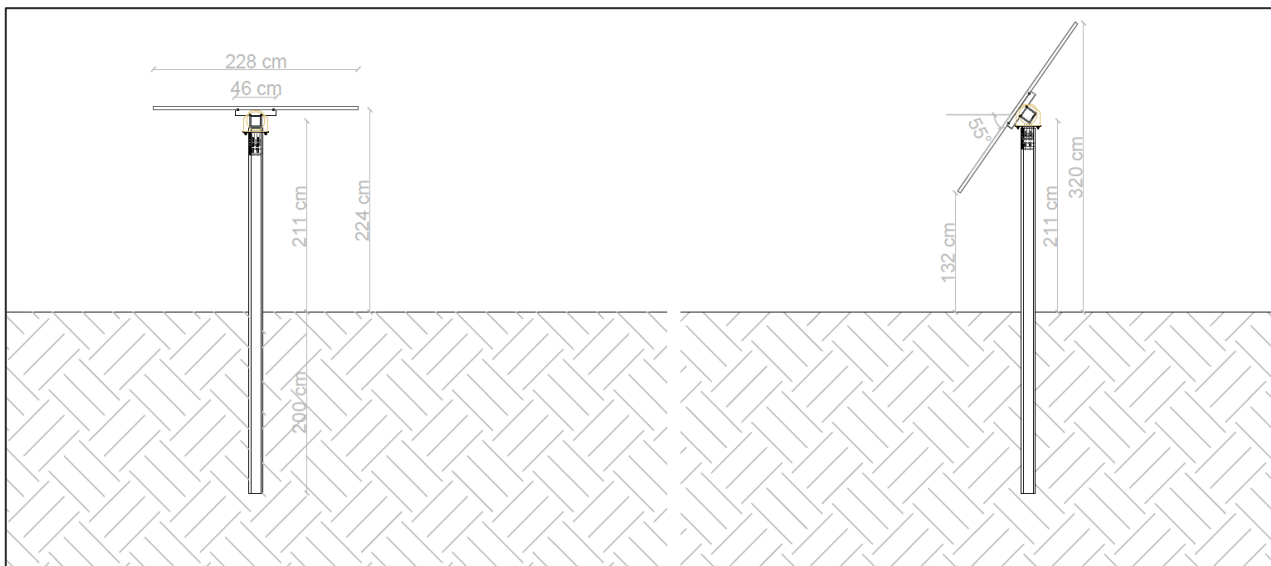
FIGURA 2: TRACKER TIPO AD ASSE VARIABILE
