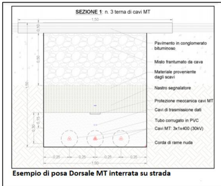
FIGURA 7: ESEMPI DI POSA DORSALI
