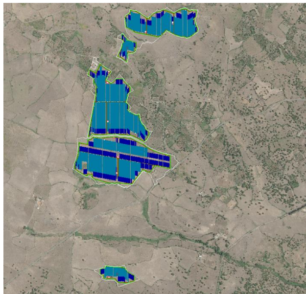
FIGURA 4: LAYOUT DI PROGETTO
