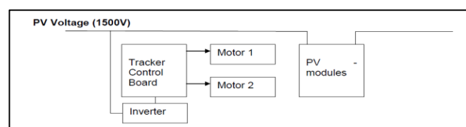
FIGURA 5: ALIMENTAZIONE DEL MOTORE DEI TRACKER DIRETTAMENTE DAL CAMPO FV
