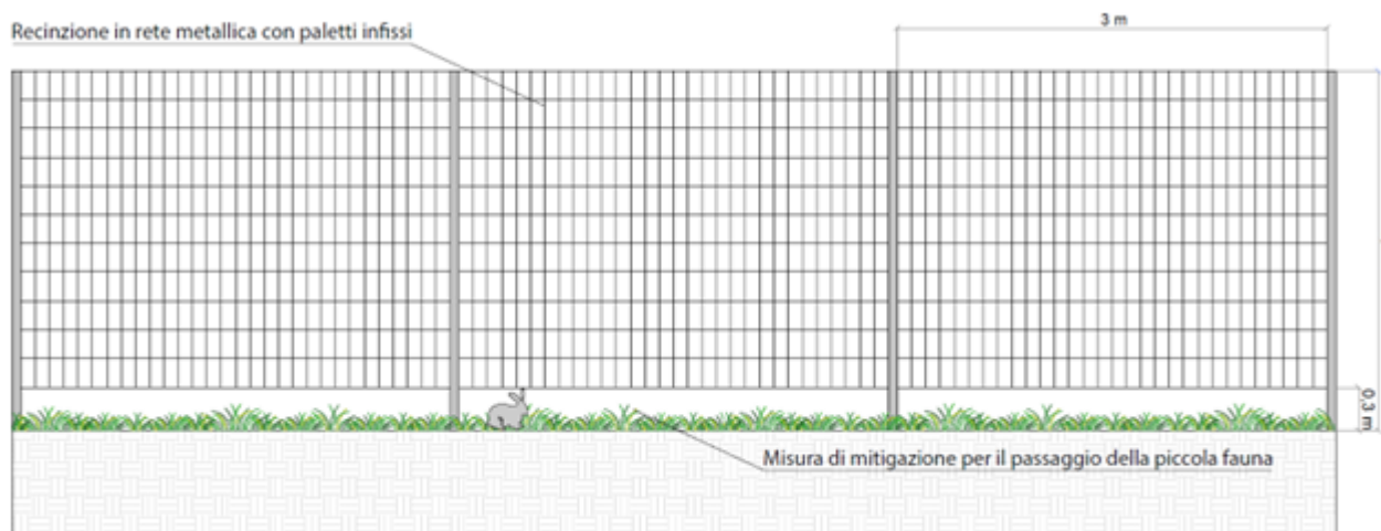
FIGURA 9: RECINZIONE TIPO
