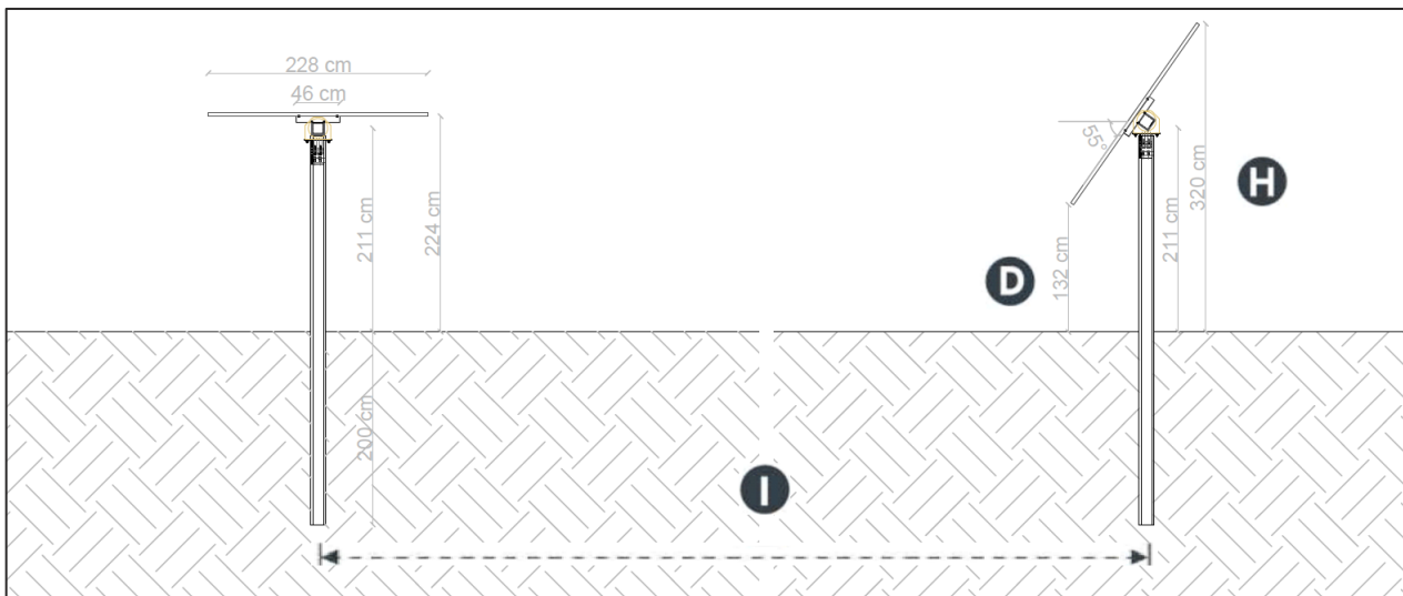
FIGURA 3: DEFINIZIONE DELLE DIMENSIONI DEI TRACKER
