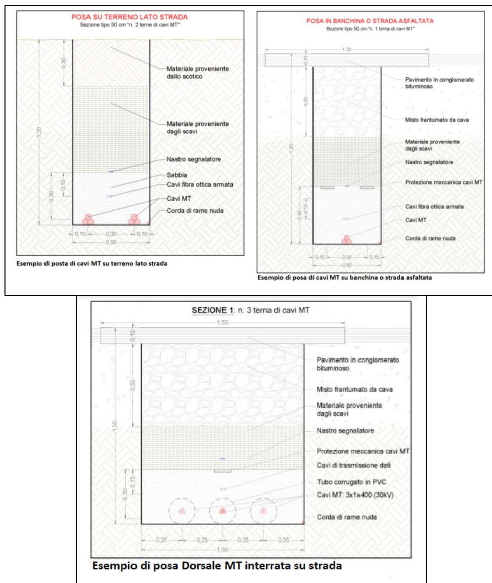
FIGURA 11: ESEMPI POSA CAVI
