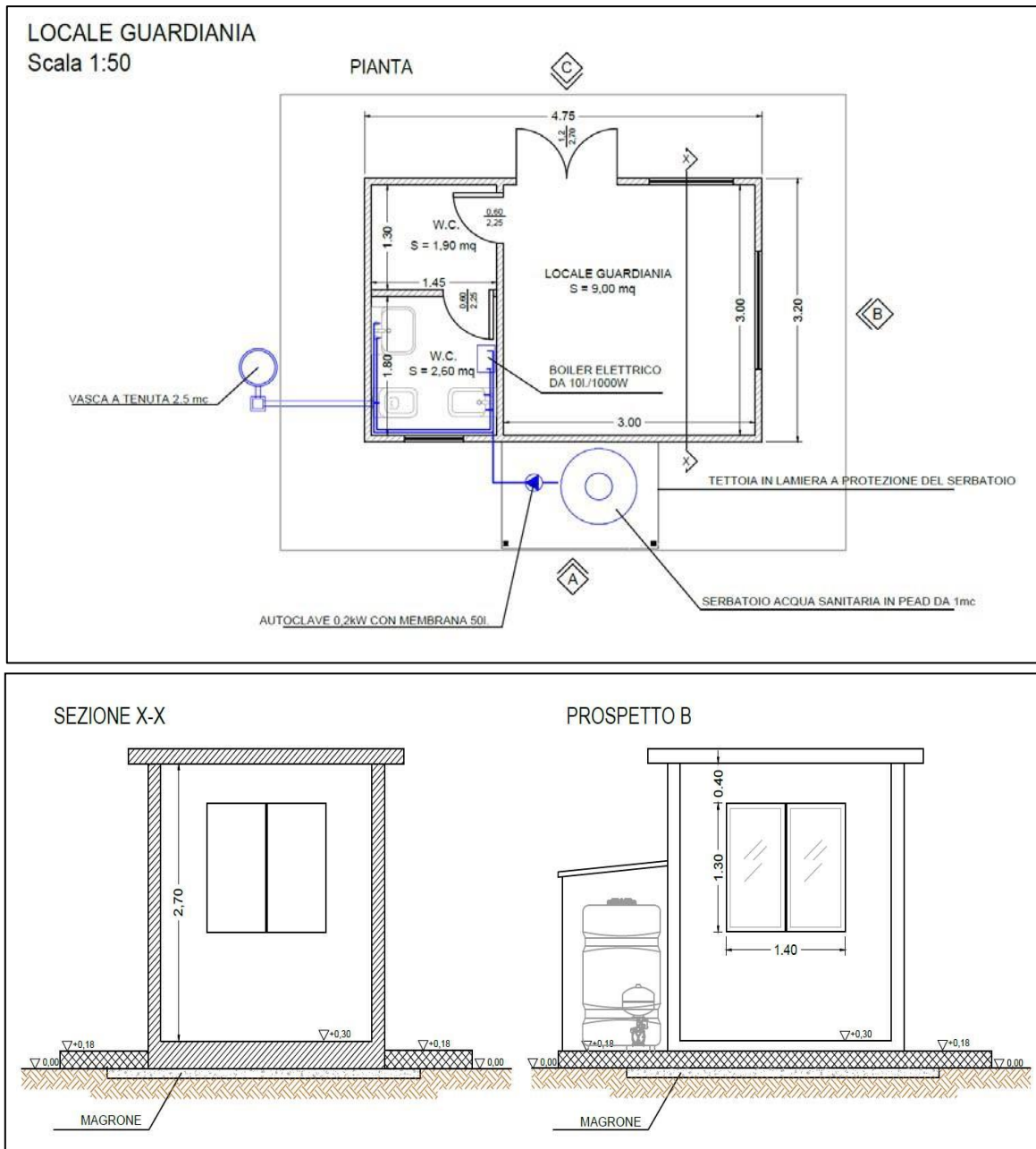
FIGURA 8: LOCALE DI GUARDIANIA
