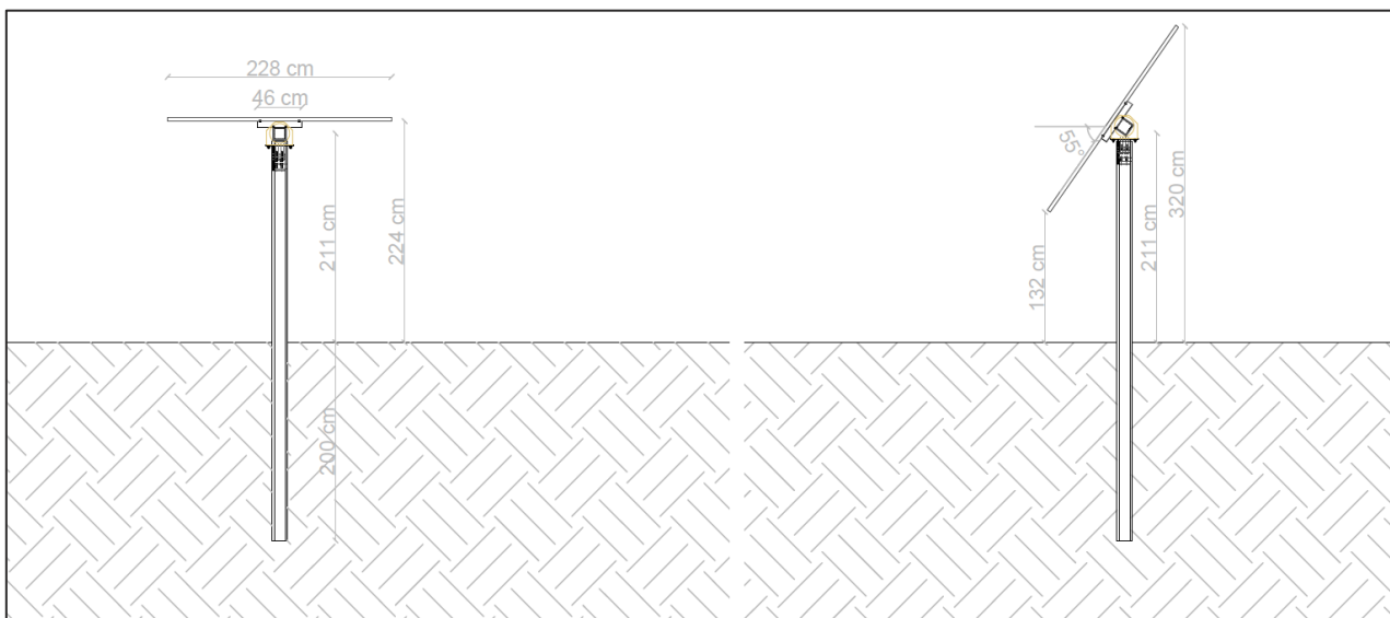
FIGURA 2: SCHEMA TIPO TRACKER AD ASSE VARIABILE
