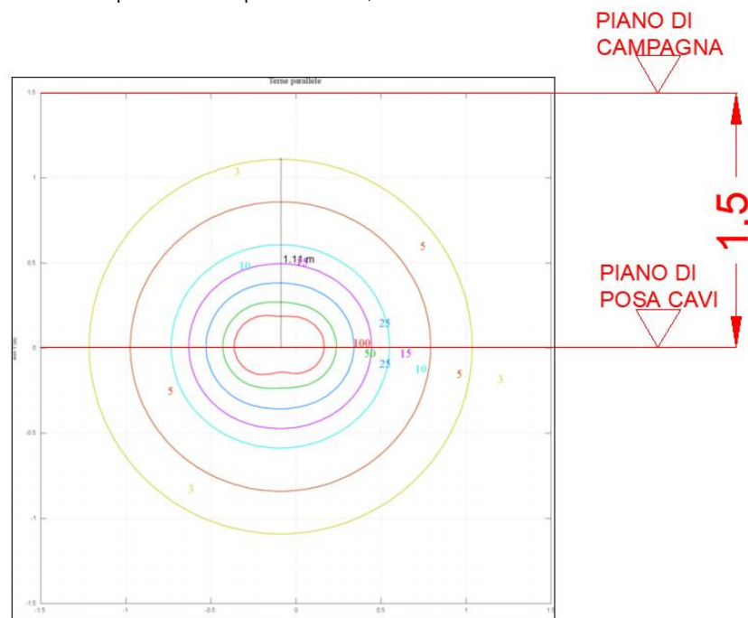
FIGURA 2: CURVE ISOINDUZIONE – 2 LINEE AT INTERRATE
