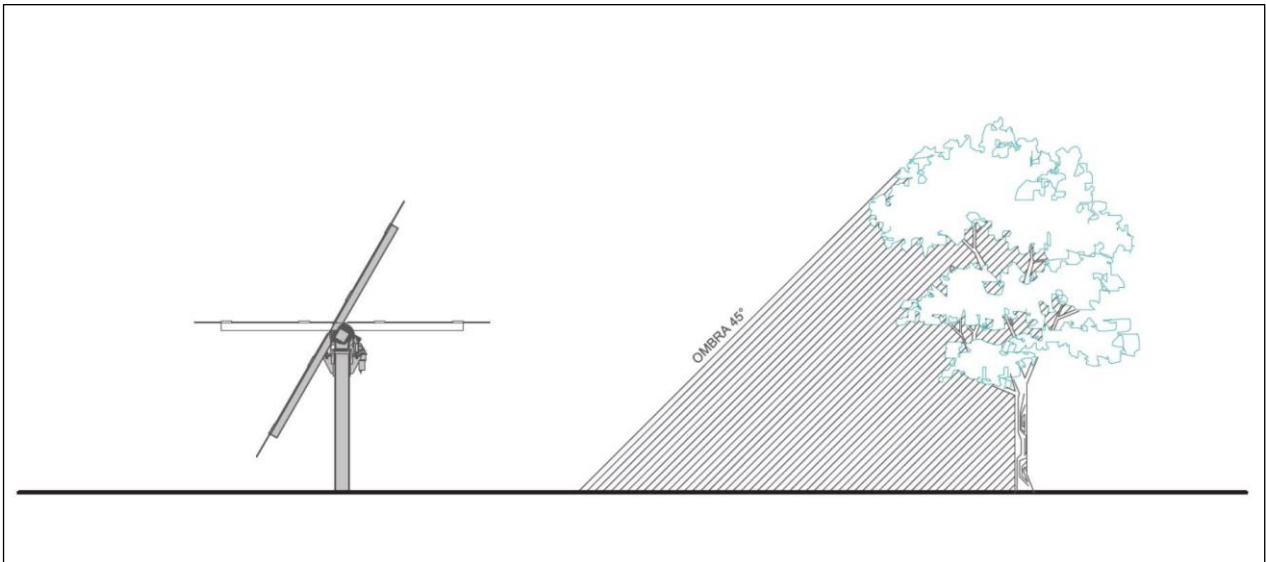
Fig. 4: Posizionamento Tracker, adeguata distanza dai fattori di ombreggiamento.
