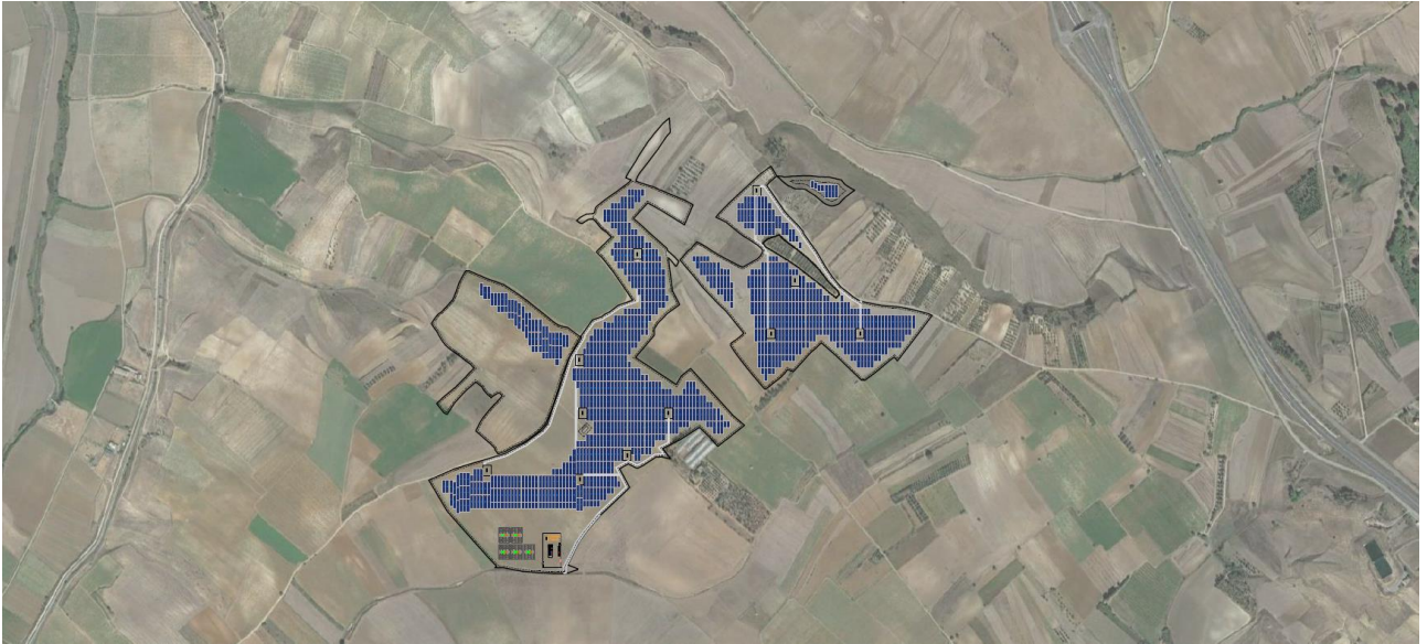
Fig. 1: Layout dell'impianto
