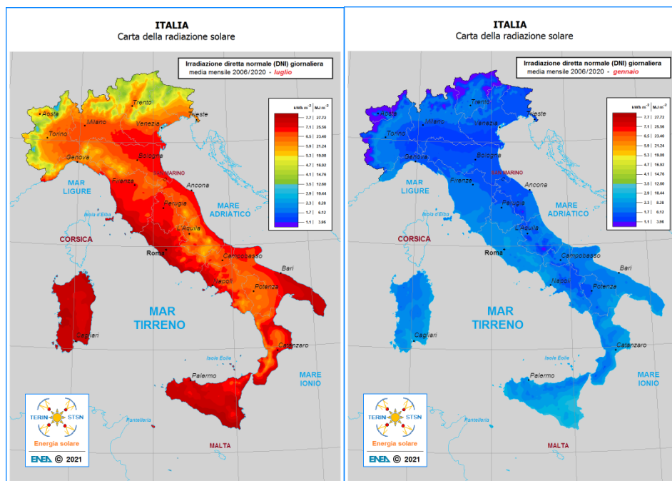
Fig. 11-12: carta della radiazione solare (DNI giornaliera) mese luglio/gennaio
