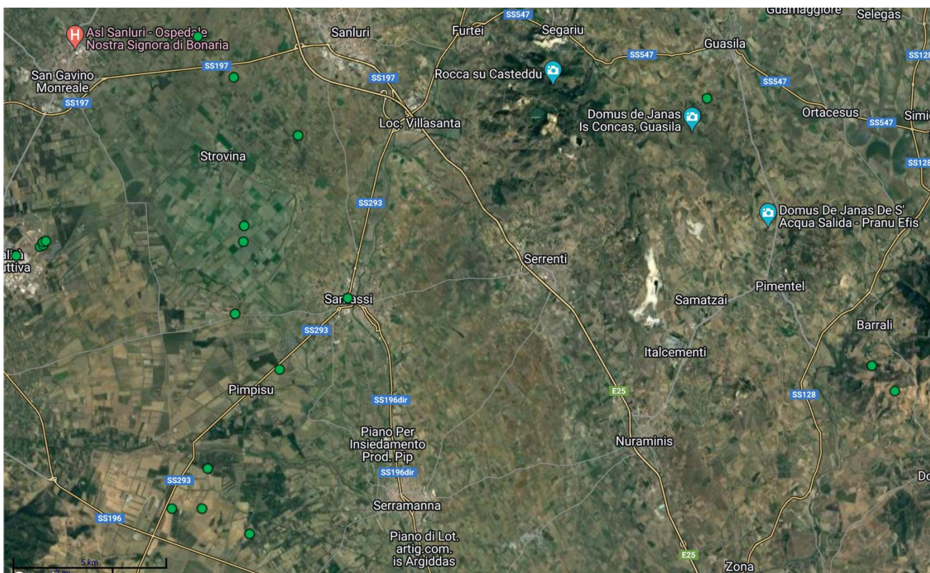
Fig. 4: WebGis di atla.gse, in verde la produzione di elettricità da fonte eolica
