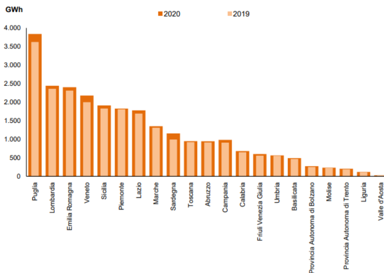
Fig.13: Produzione degli impianti fotovoltaici nelle regioni italiane nel 2019 e 2020
