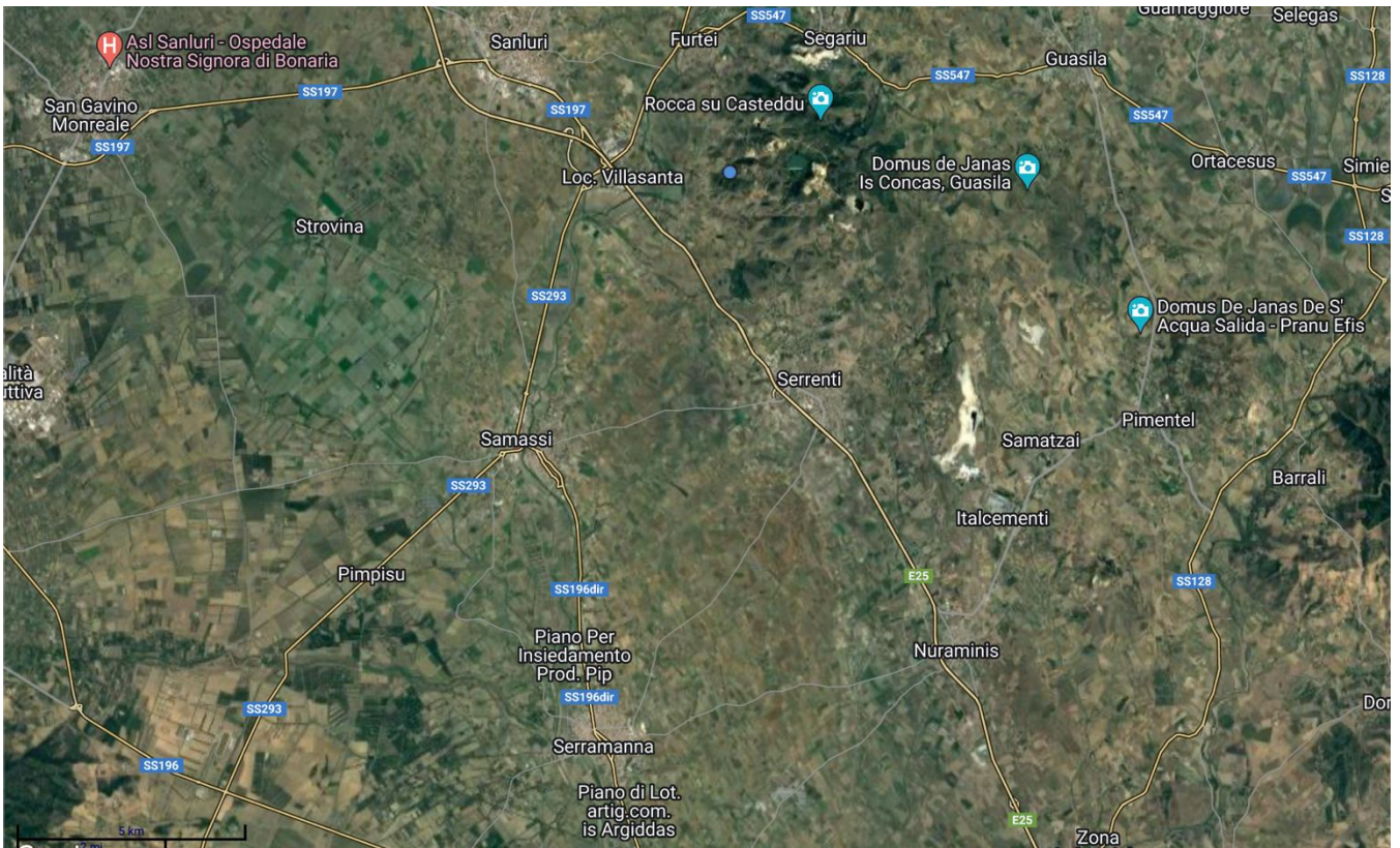
Fig. 6: WebGis di atla.gse, in celeste la produzione di energia da fonte idraulica
