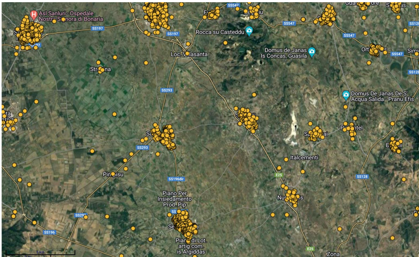
Fig. 3: WebGis di atla.gse, in giallo la produzione di elettricità da fonte solare
