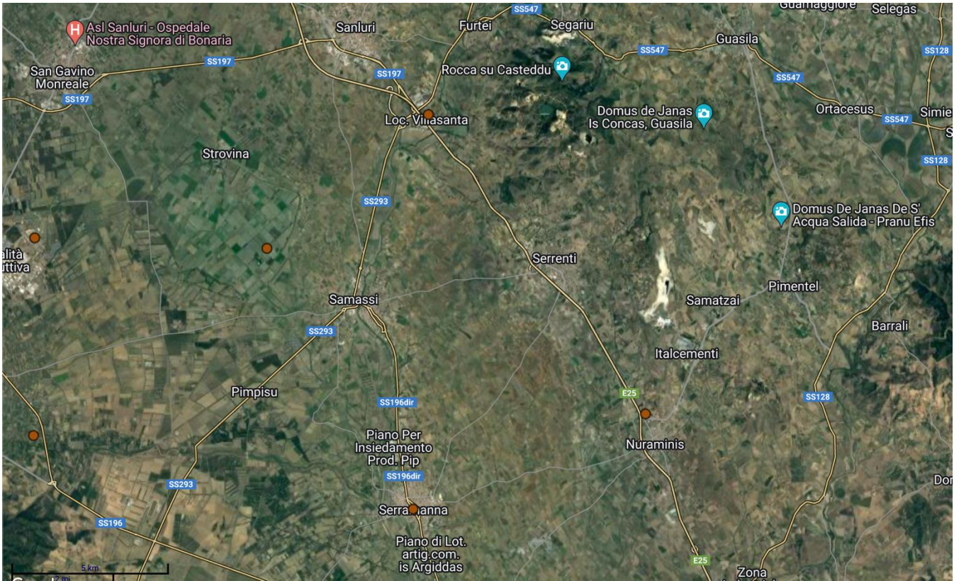
Fig. 5: WebGis di atla.gse, in rosso la produzione di elettricità da bioenergie
