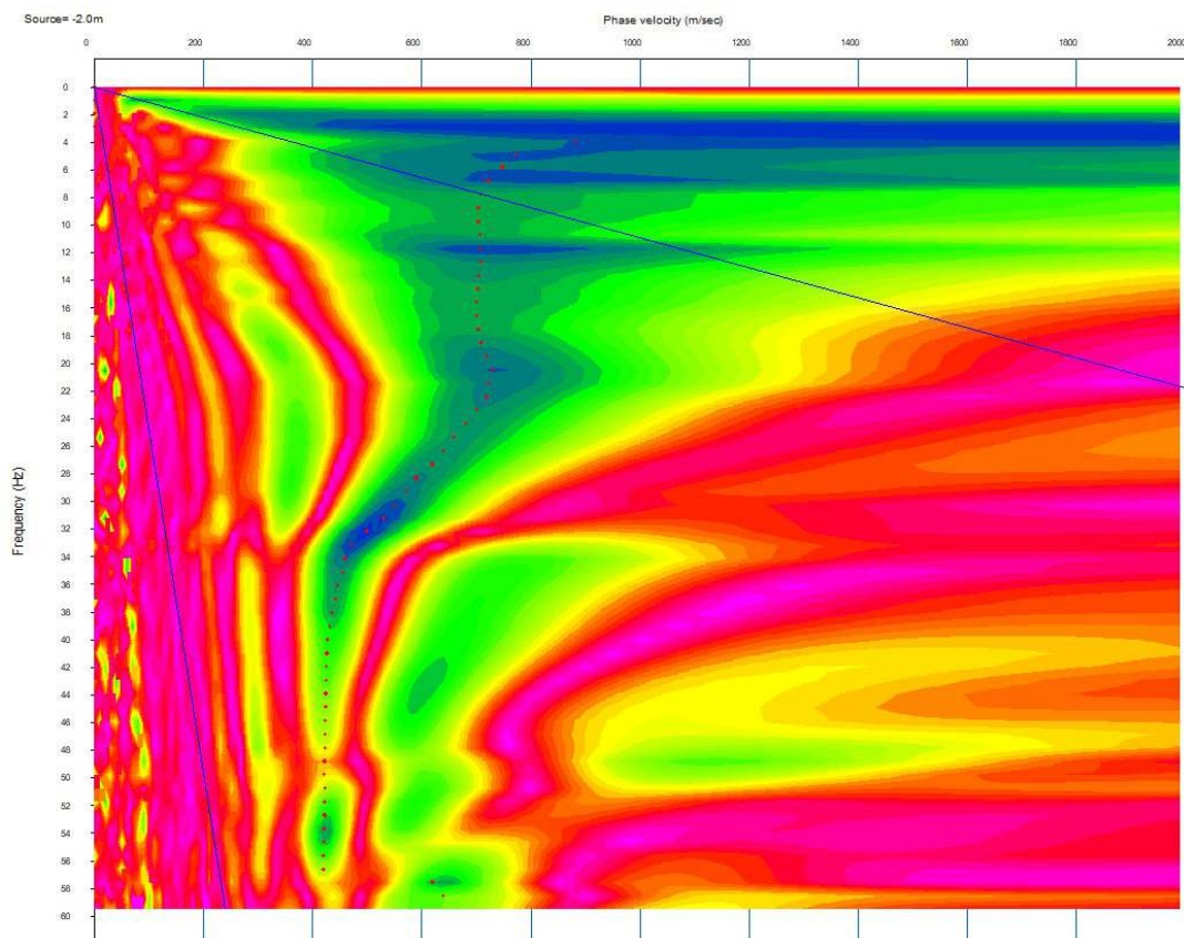
Figura 5.3– Curva di dispersione
