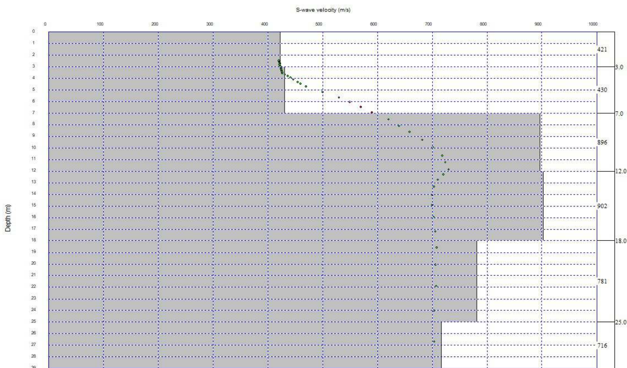
Figura 5.4 – modello stratigrafico delle Vs
