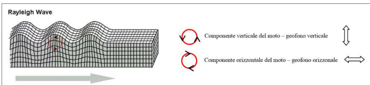
Figura 4.2– Rappresentazione onde superficiali
