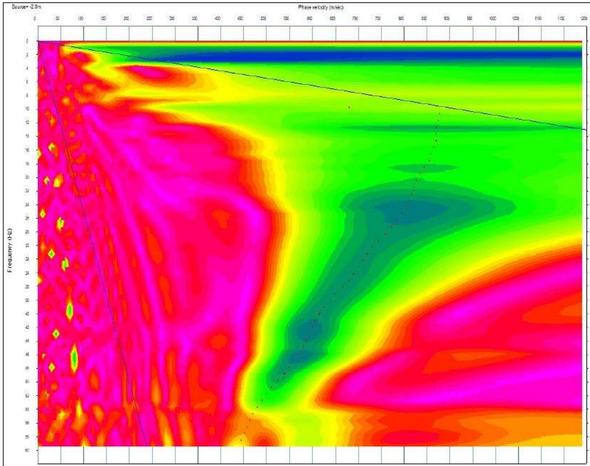
Figura 5.7 – Curva di dispersione
