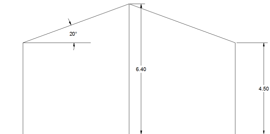
Figura 7.3: Sezione edificio ricovero mezzi agricoli
