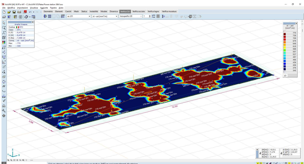
Figura 6.17: Differenze di armatura [xt-axt] – verifiche oK
