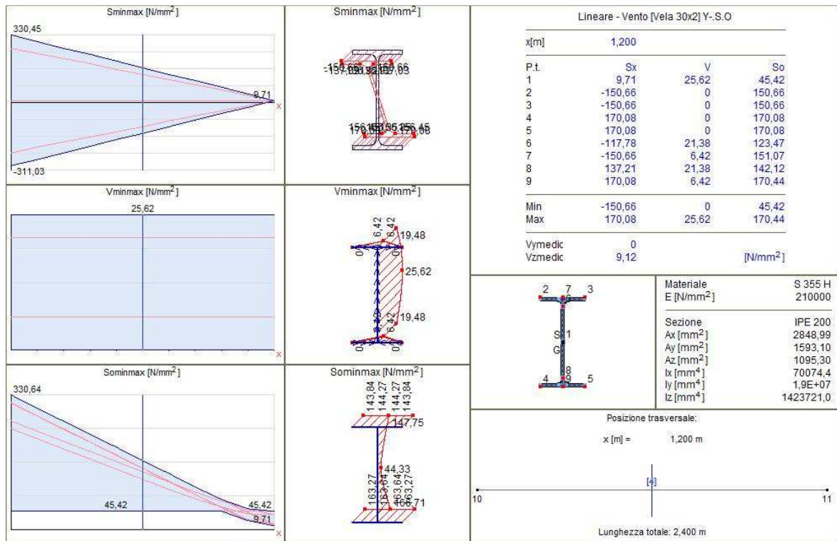
Figura 5.18: calcolo delle tensioni negli elementi strutturali – montanti
