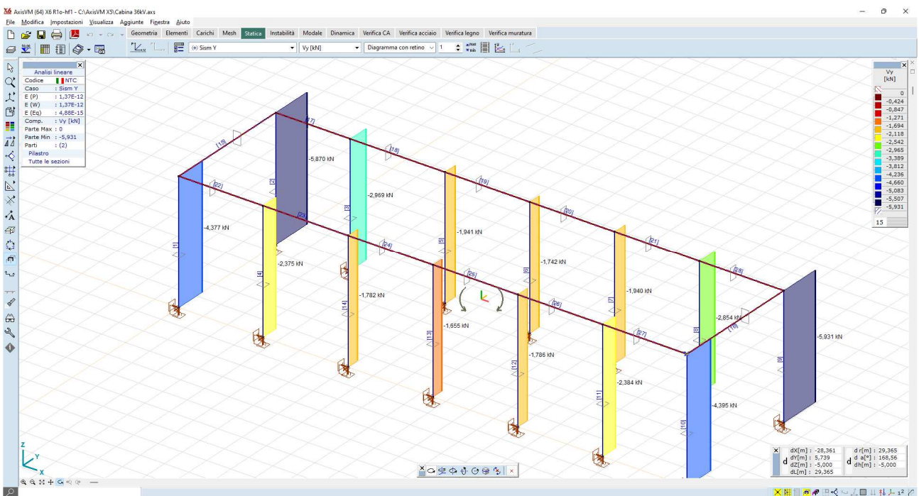
Figura 8.14: azioni taglianti Vy comb sism Y – valori max 5,8 kN
