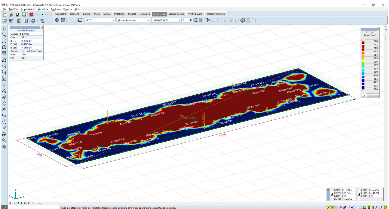
Figura 6.15: Differenze di armatura [yt-ayt] – verifiche ok
