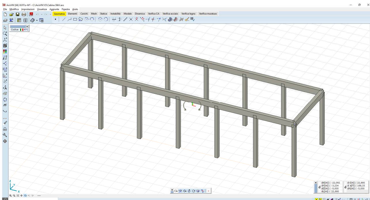
Figura 8.6: vista assometrica del modello ad aste_render
