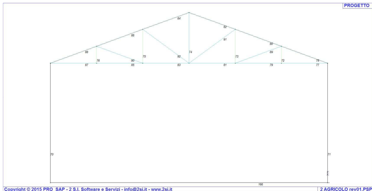
Figura 7.4: Modello 2D dell'edificio agricolo
