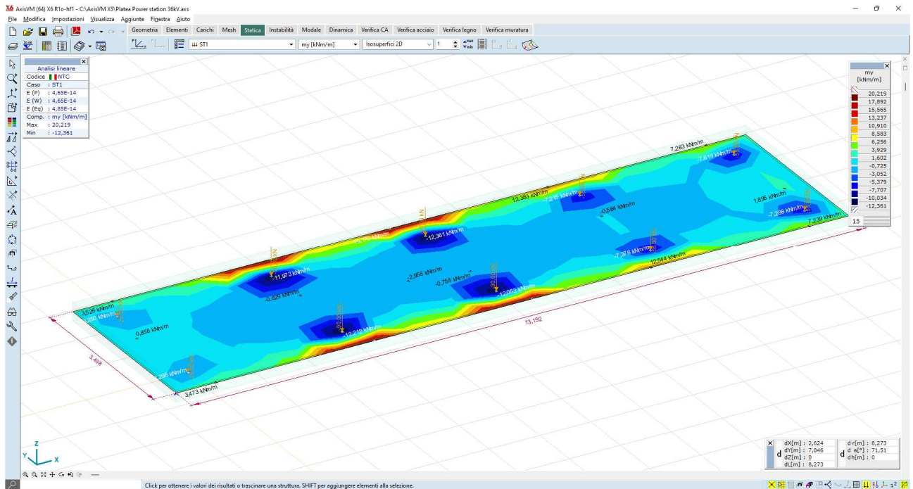
Figura 6.9: Sollecitazioni elemento plate – my – valori max 17,8 kNm/m
