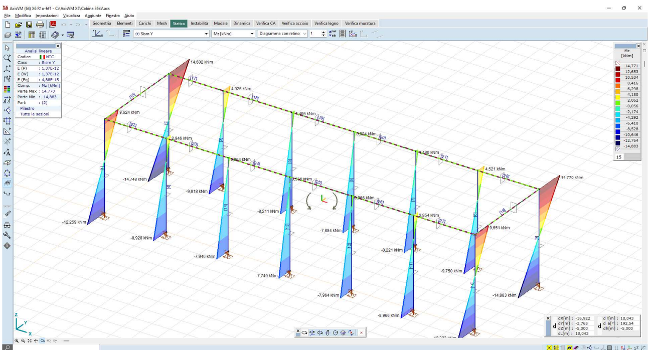
Figura 8.12: momenti flettenti Mz comb sism Y – valori max pilastri 14,7 kNm
