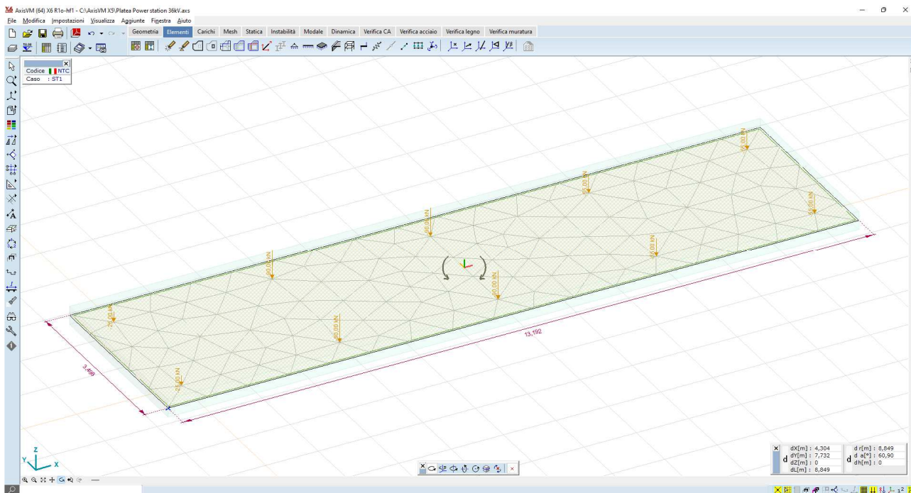
Figura 6.6: carichi concentrati nodali - scarichi al piede
