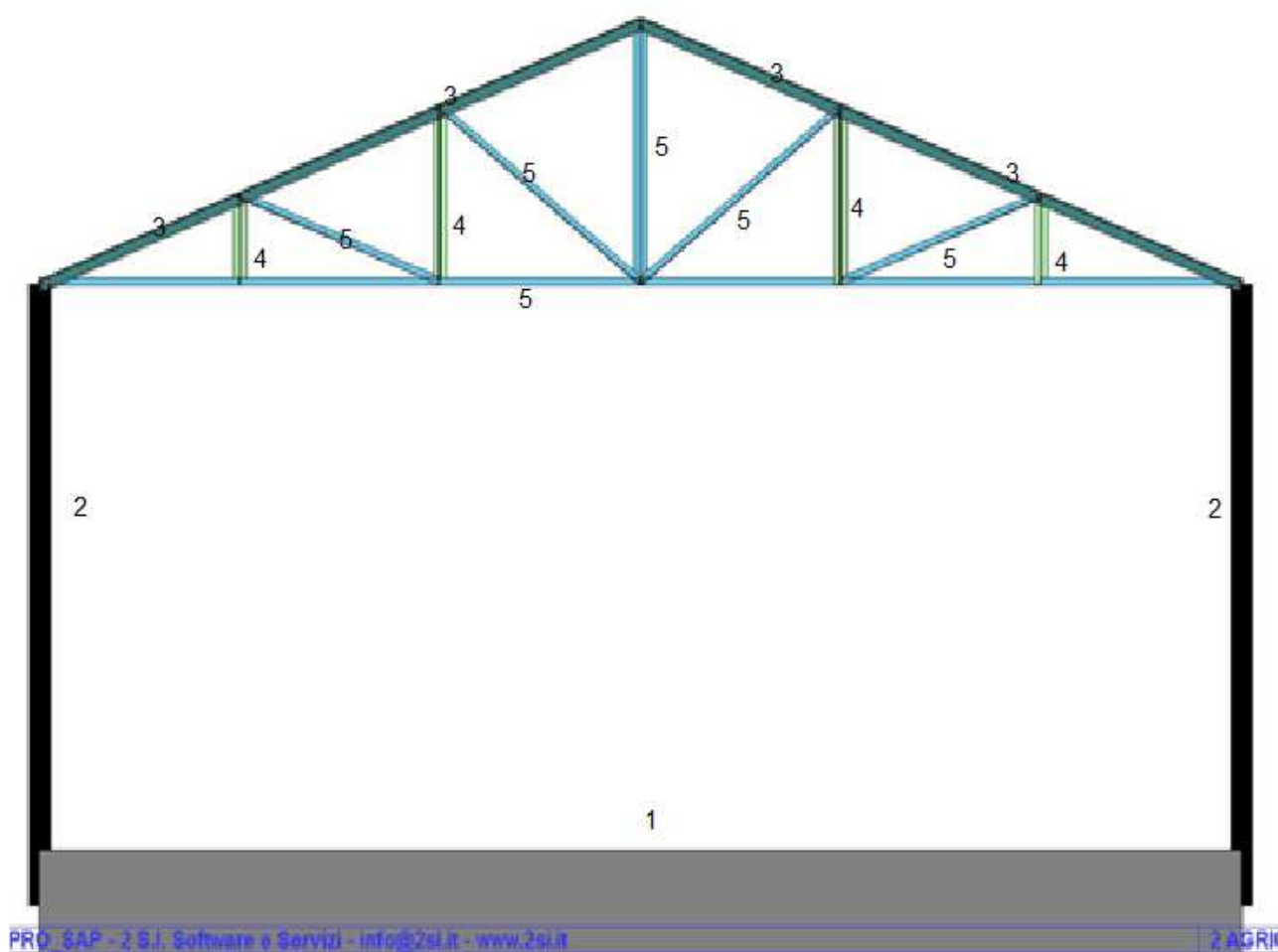
Figura 7.5: Tipologie di sezioni
