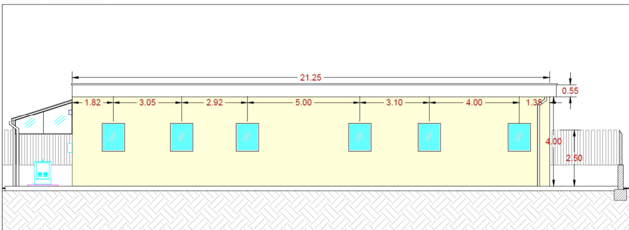
Vista B - Scala 1:100
