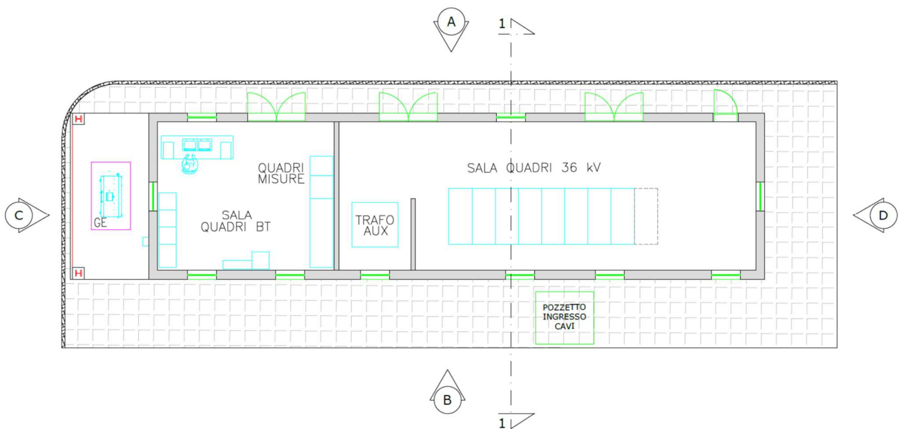
Figura 8.1: Pianta architettonica edificio
