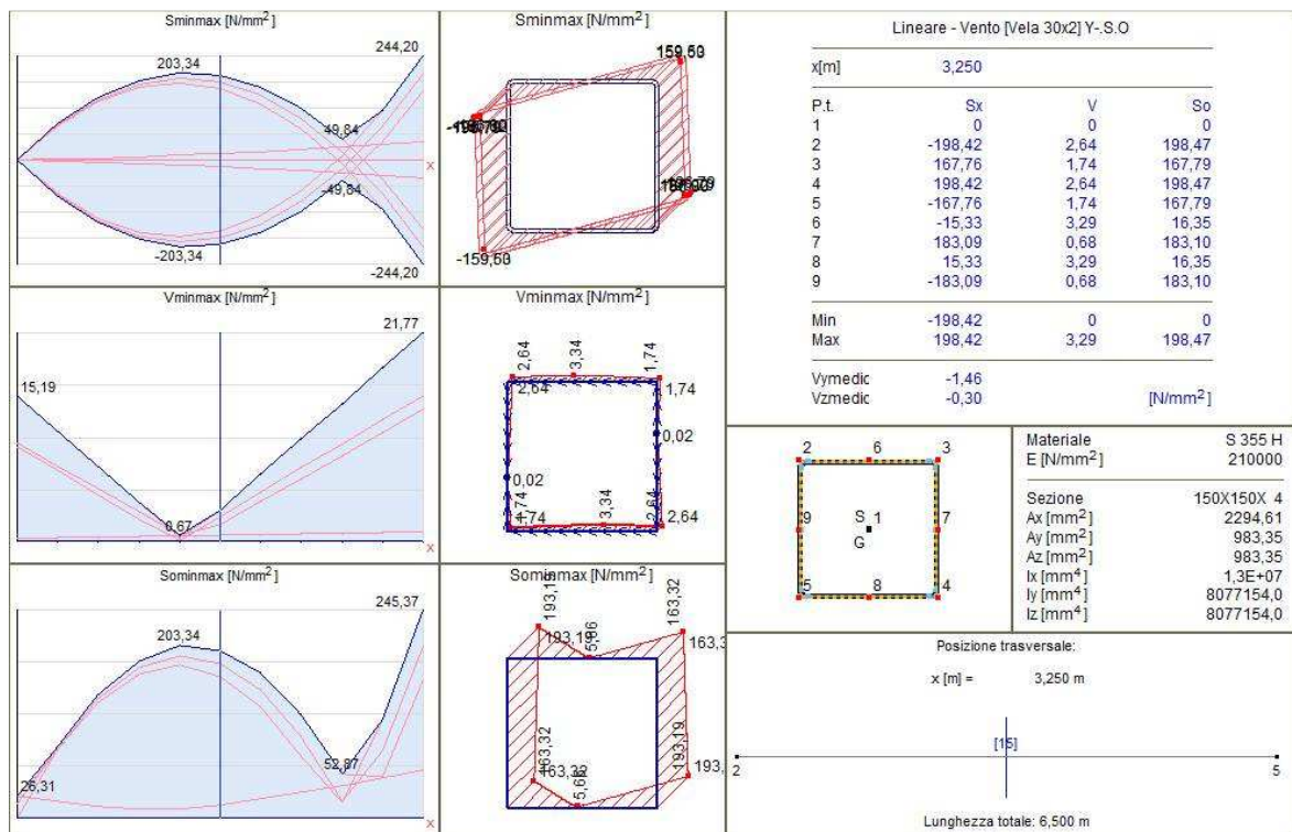
Figura 5.19: calcolo delle tensioni negli elementi strutturali – trave
