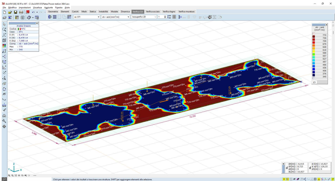
Figura 6.16: Differenze di armatura [xb-axb] – verifiche oK
