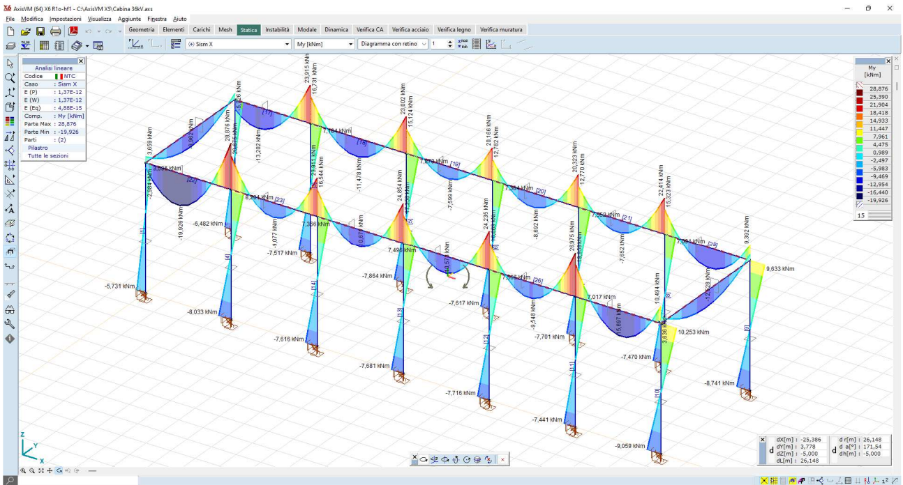
Figura 8.11: momenti flettenti My comb sism X – valori max travi 23kNm valori max pilastri 9,6 kNm
