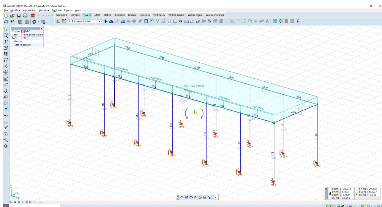
Figura 8.7: Carichi permanenti portati
