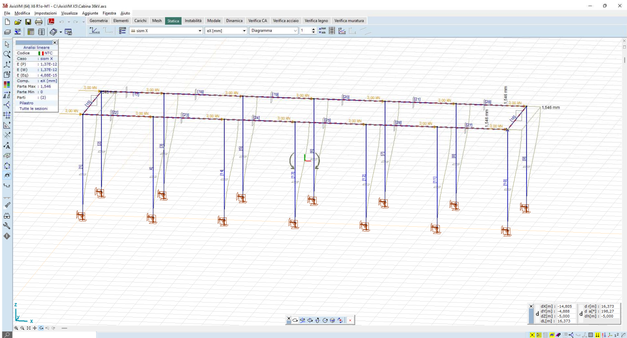
Figura 8.17: configurazione deformata sism X – valori max 1,6 mm
