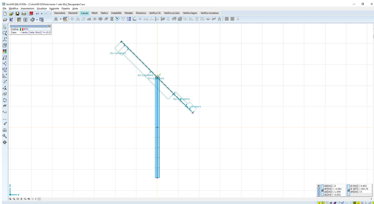
Figura 5.9: carico vento Y+S.O.
