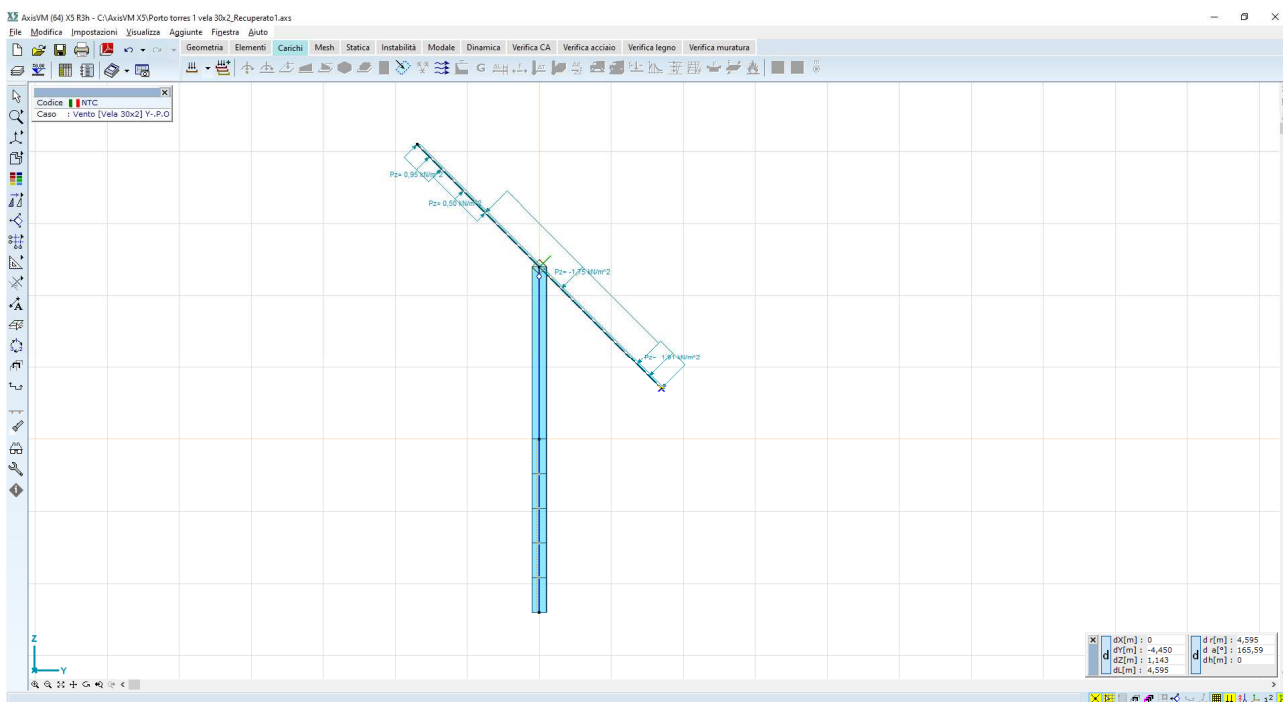
Figura 5.10: carico vento Y-P.O.
