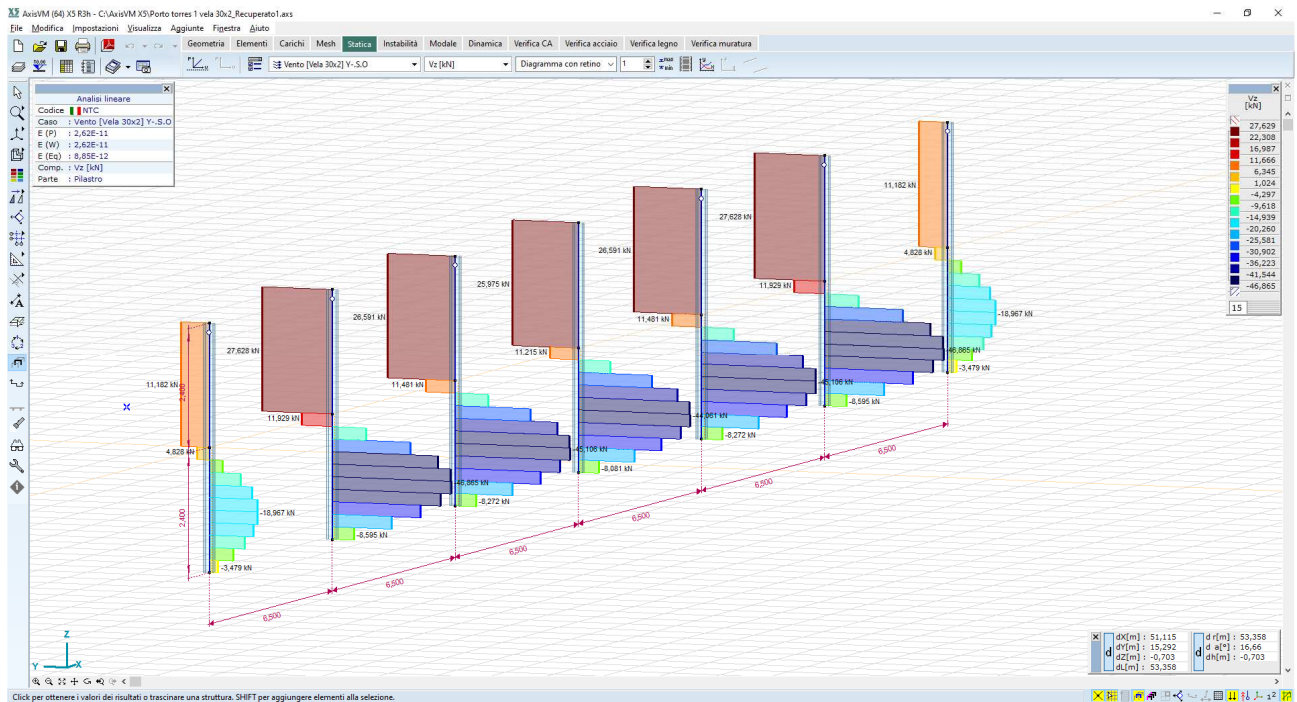
Figura 5.14: diagrammi del taglio V_z – montanti - valori massimi dell'ordine dei 36kN – combinazione Y-S.O.
