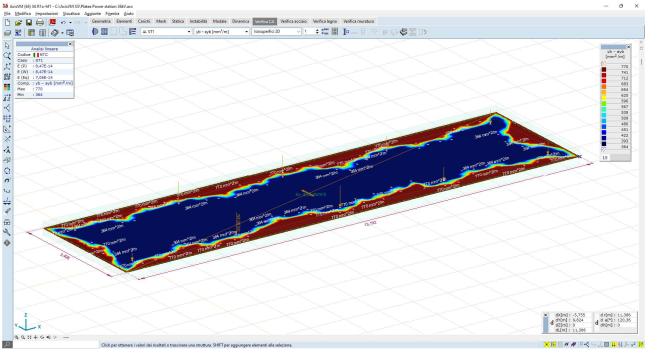
Figura 6.14: Differenze di armatura [yb-ayb] – verifiche ok
