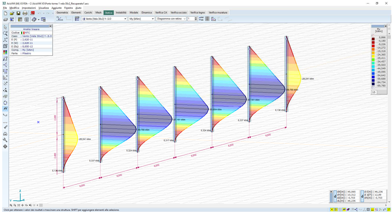
Figura 5.13: diagrammi del momento flettente M_y – montanti - valori massimi dell'ordine dei 67kN*m – combinazione Y-S.O.
