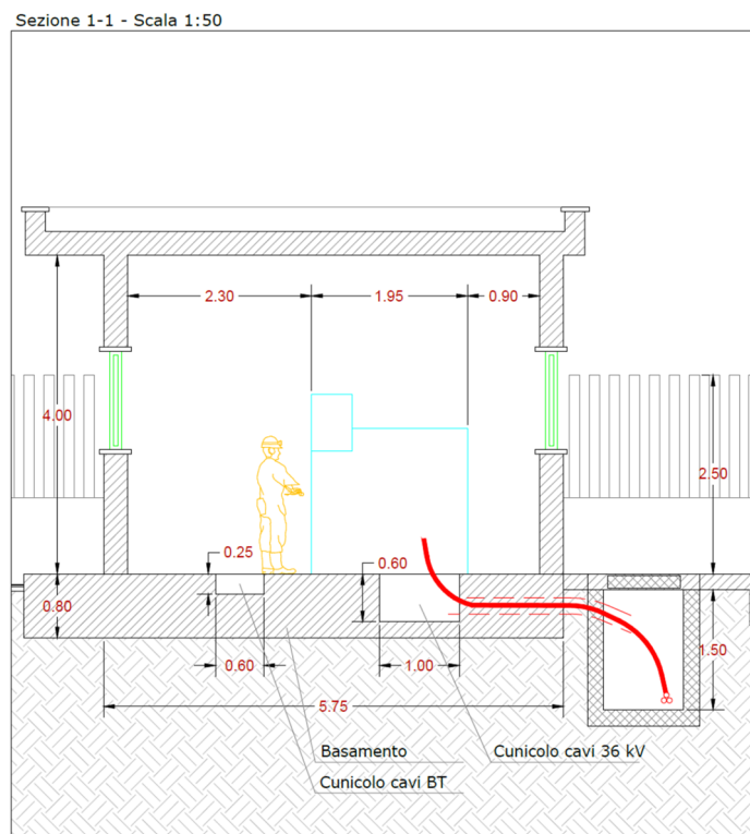
Figura 8.4: Sezione architettonica trasversale
