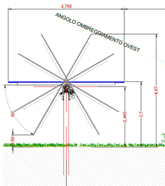
Figura 5.3 - Sezione trasversale della struttura tipo
