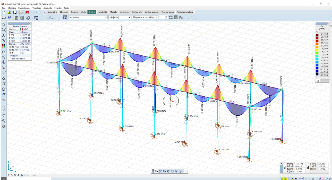
Figura 8.10: momenti flettenti My comb statico – valori max travi 20 kNm
