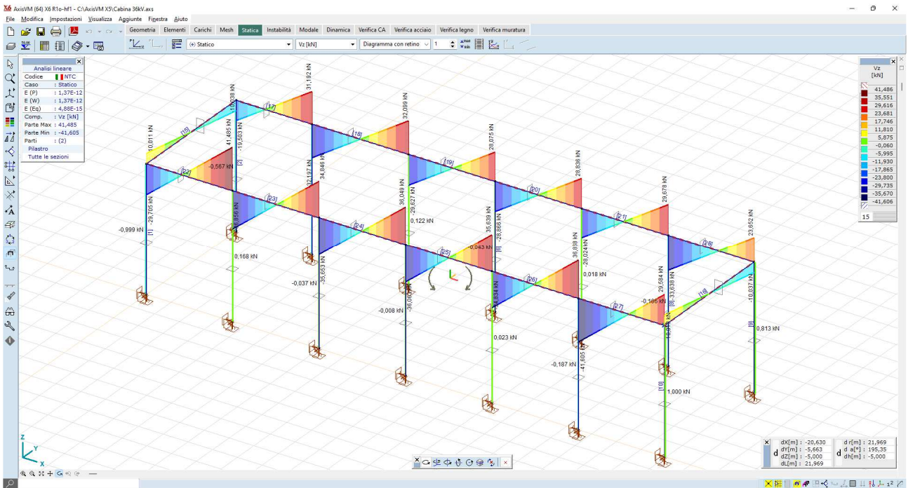
Figura 8.13: azioni taglianti Vz comb statico – valori max travi 35 kNm
