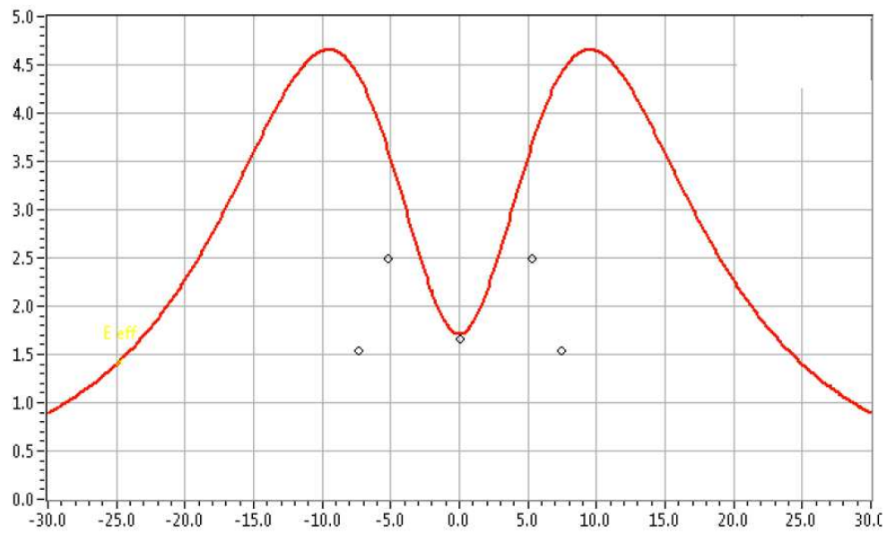
Figura 10.3 – Andamento del campo elettrico a 1,50 m dal suolo del raccordo linea 380 kV (sezione con conduttori in piano a 11.5 m dal suolo)
