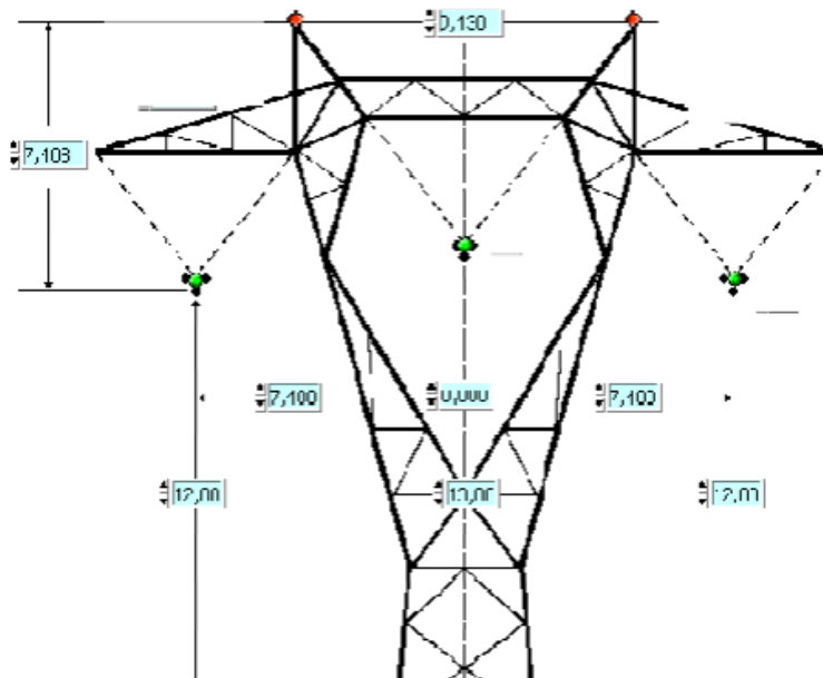
Figura 10.1 – disposizione geometrica dei conduttori sul sostegno tipico
