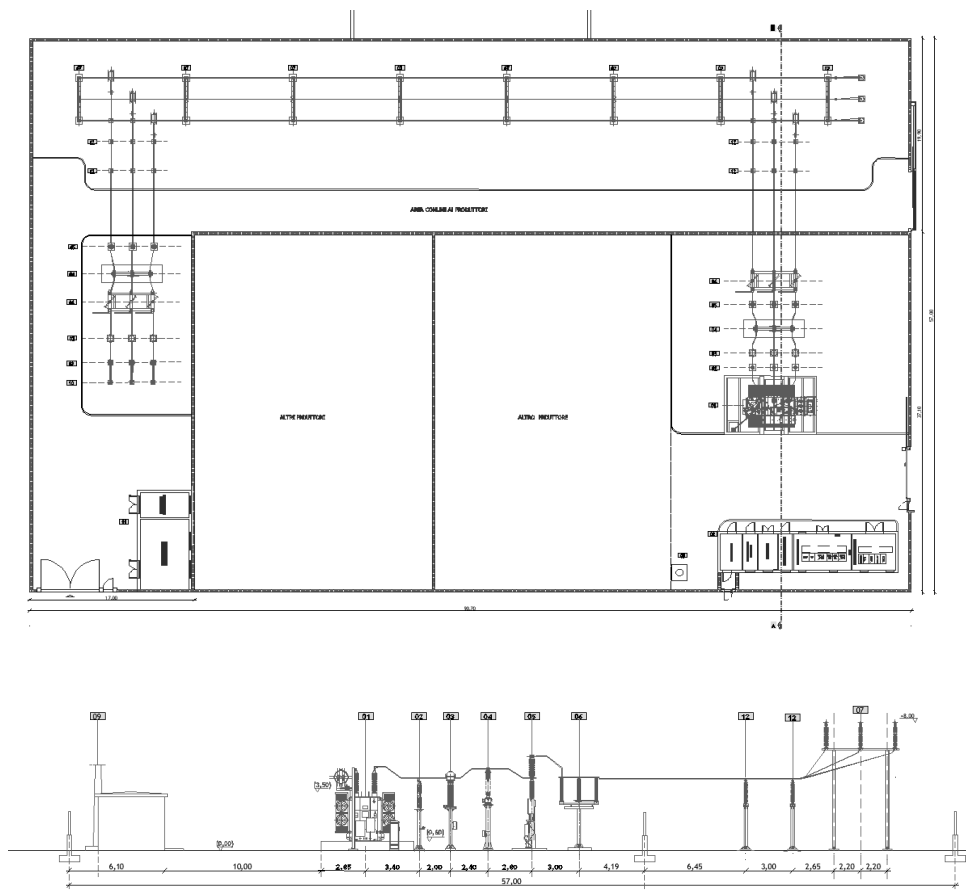
Figura 6 - Planimetria elettromeccanica della Stazione Elettrica di Utanza
