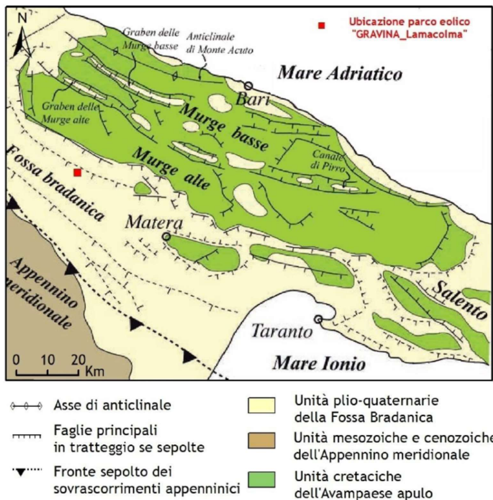
Figura 6.1: Carta geologica schematica (Inquadramento Geologico Locale).
