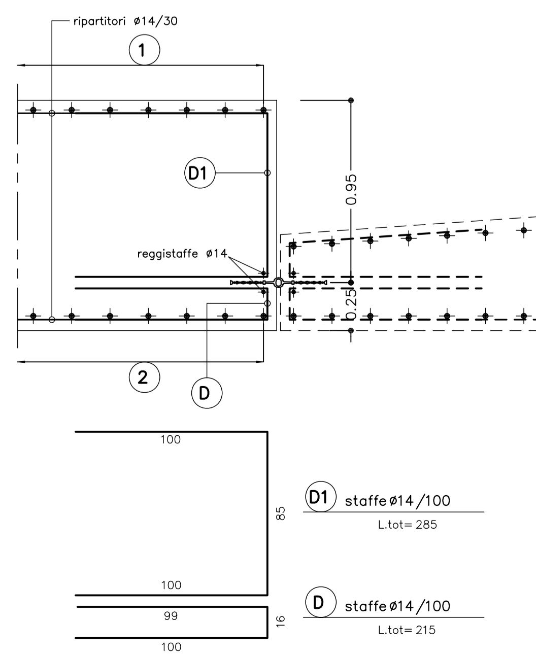
PARTICOLARE "D" SCALA 1:20 PARTICOLARE WATER-STOP PROFILO LONGITUDINALE C-C
