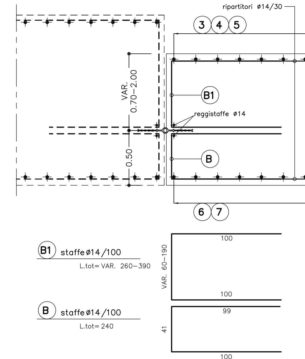
PARTICOLARE "B" SCALA 1:20 PARTICOLARE WATER-STOP PIANTA D-D
