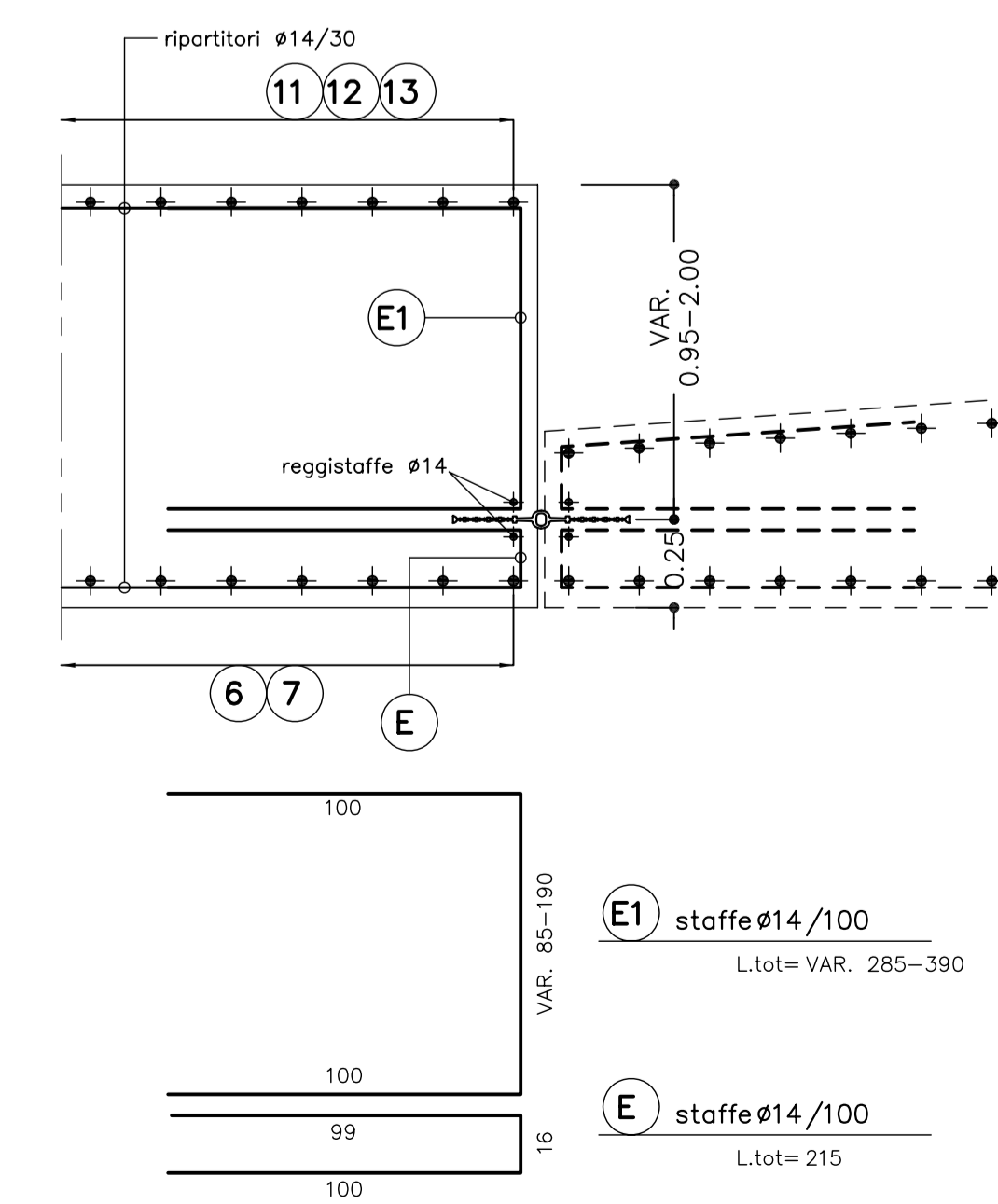
PARTICOLARE "E" SCALA 1:20 PARTICOLARE WATER-STOP PIANTA D-D
