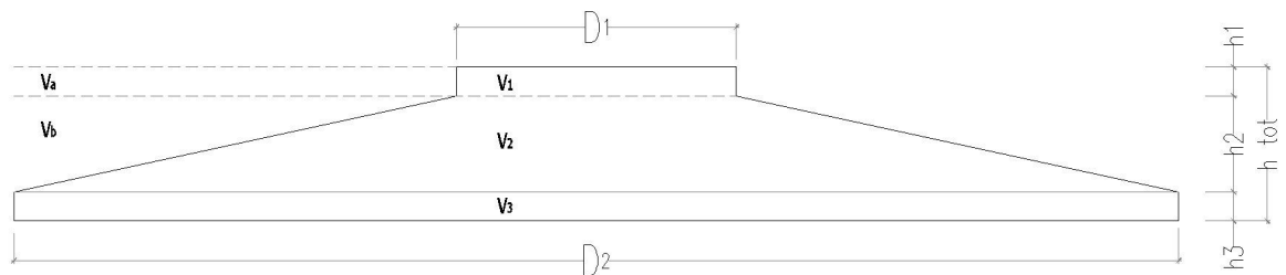
Schema in sezione basamento di fondazione
