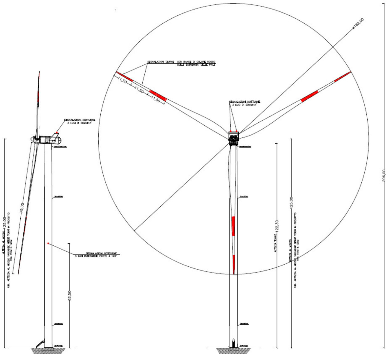
Figura 5 Prospetto e sezione dell'aerogeneratore tipo VESTAS – V162-6 MW
