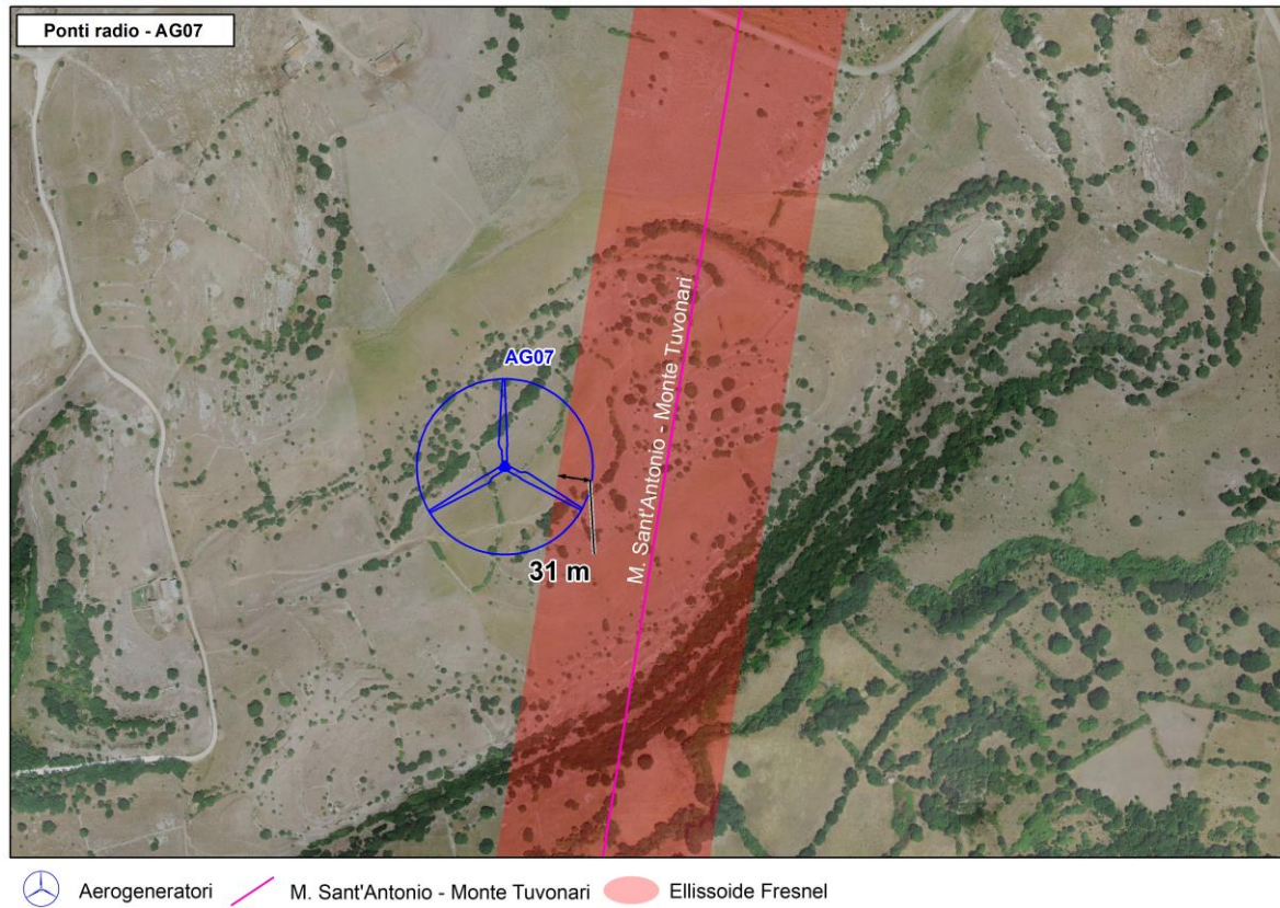
Figura 10: ellissoide di Fresnel del ponte radio Monte Sant'Antonio – Monte Tuvonari sul piano orizzontale.
