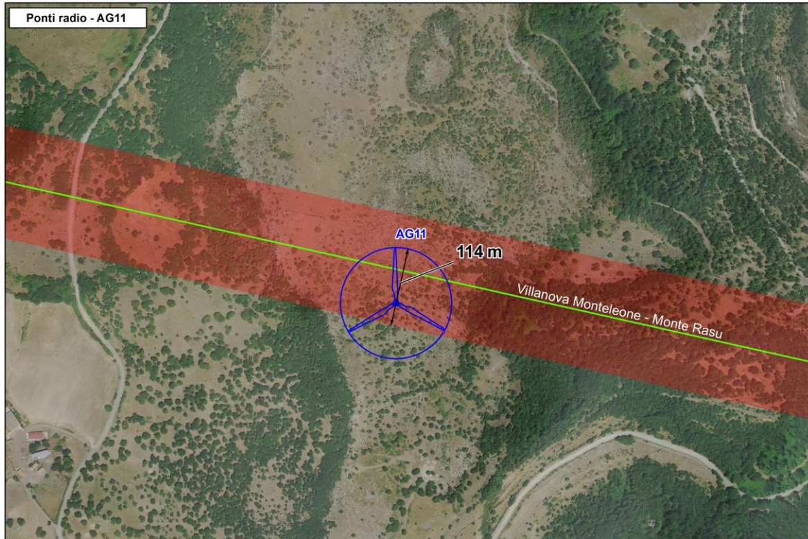
Figura 12: ellissoide di Fresnel del ponte radio Villanova Monteleone – Monte Rasu sul piano orizzontale.
