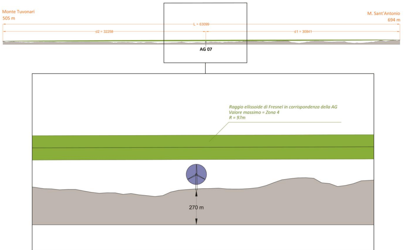
Figura 11: ellissoide di Fresnel del ponte radio Monte Sant'Antonio - Monte Tuvonari sul piano verticale.
