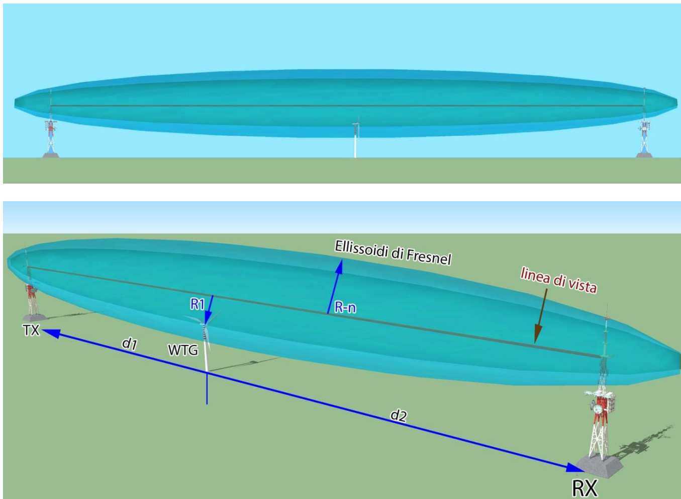
Figura 7 - Rappresentazione schematica interferenza AG con le zone di Fresnel tra due ponti radio.
