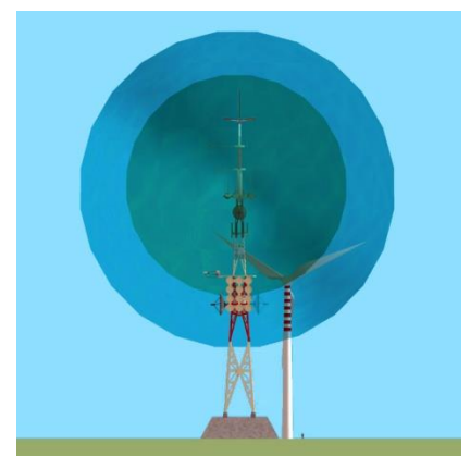
Figura 6 - Interferenza di un aerogeneratore con le zone di Fresnel
