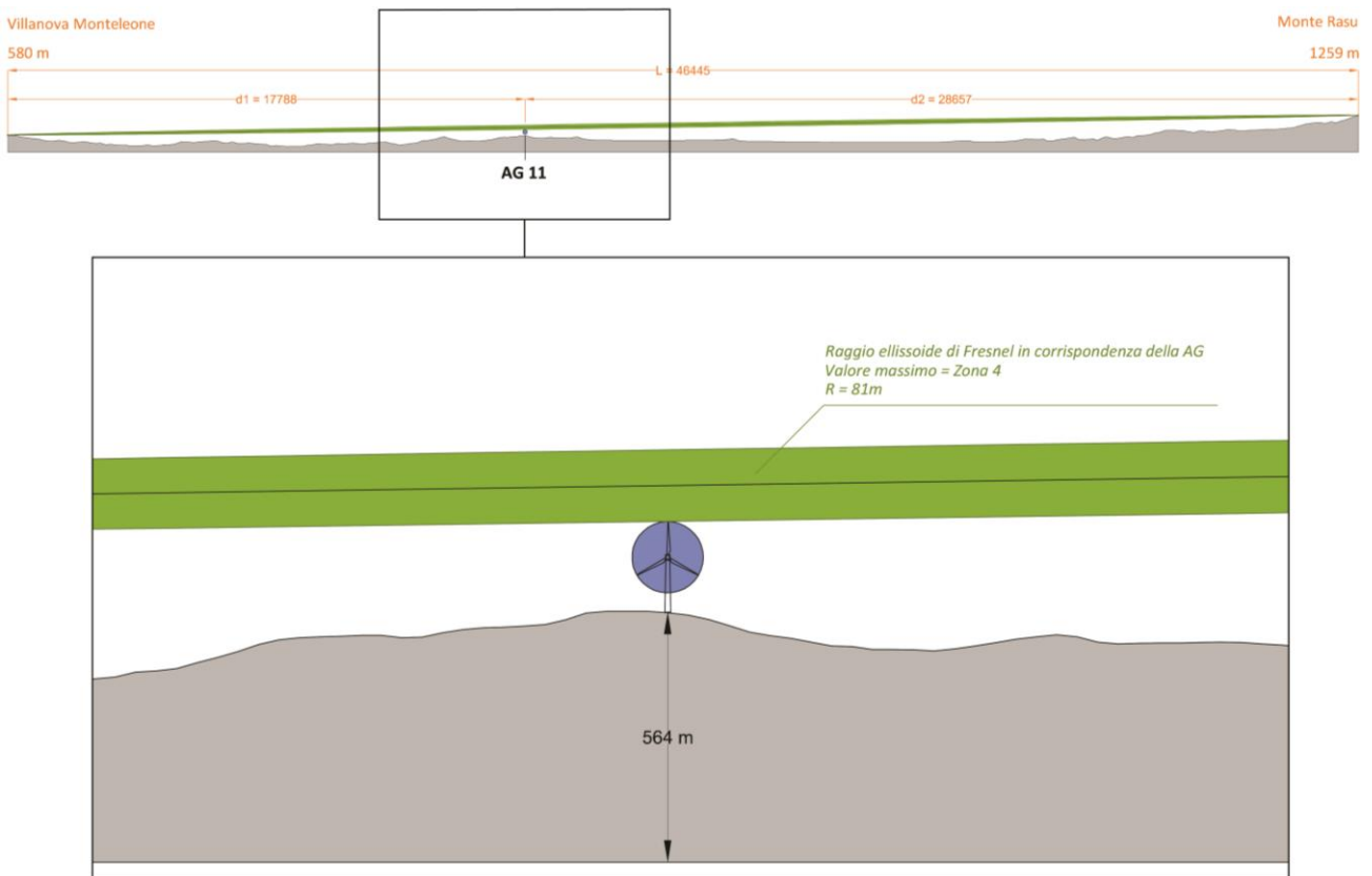
Figura 13: ellissoide di Fresnel del ponte radio Villanova Monteleone – Monte Rasu sul piano verticale.
