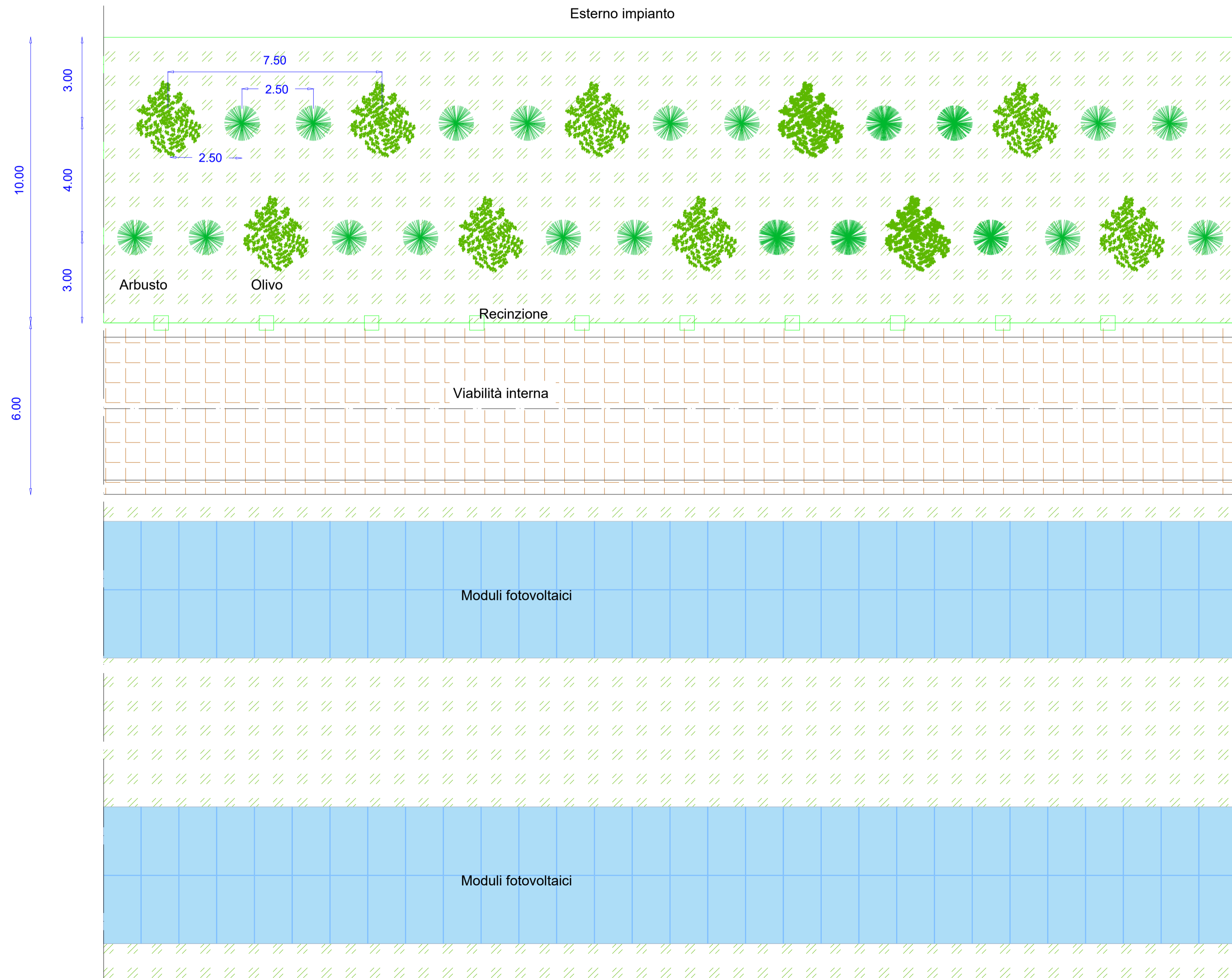
PIANTA
