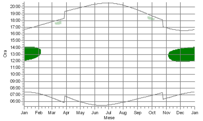
2: VESTAS V105-3.45 3450 105.0 !O! hub: 72,5 m (TOT: 125,0 m) (3)
