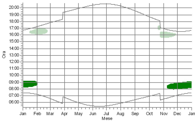
3: VESTAS V105-3.45 3450 105.0 !O! hub: 72,5 m (TOT: 125,0 m) (4)
