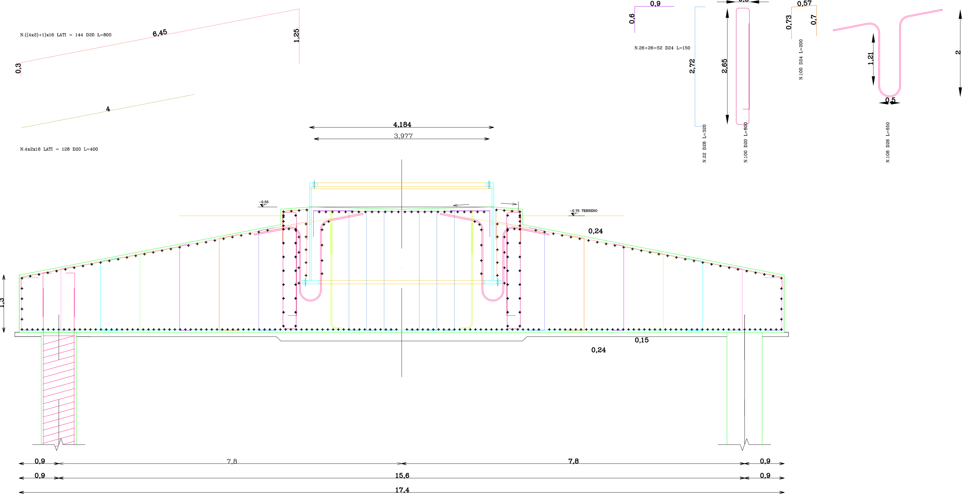
SEZIONE
