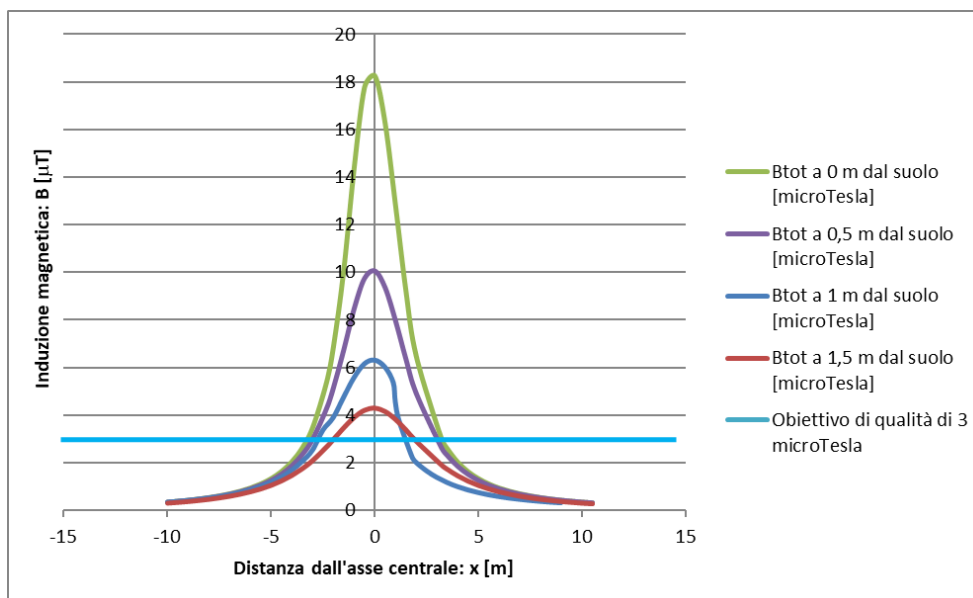
Figura 3: Andamento del campo magnetico generato dal cavidotto, composto da sei terne da 630 mm 2
