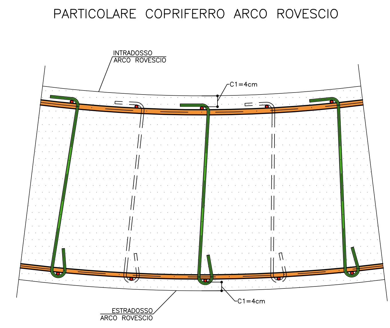
PARTICOLARE "2" SCALA 1:10
