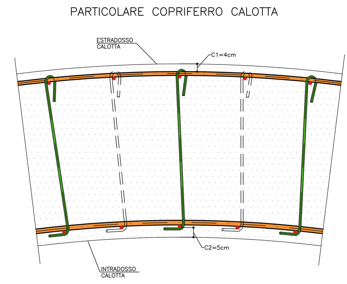
PARTICOLARE "1" SCALA 1:10
