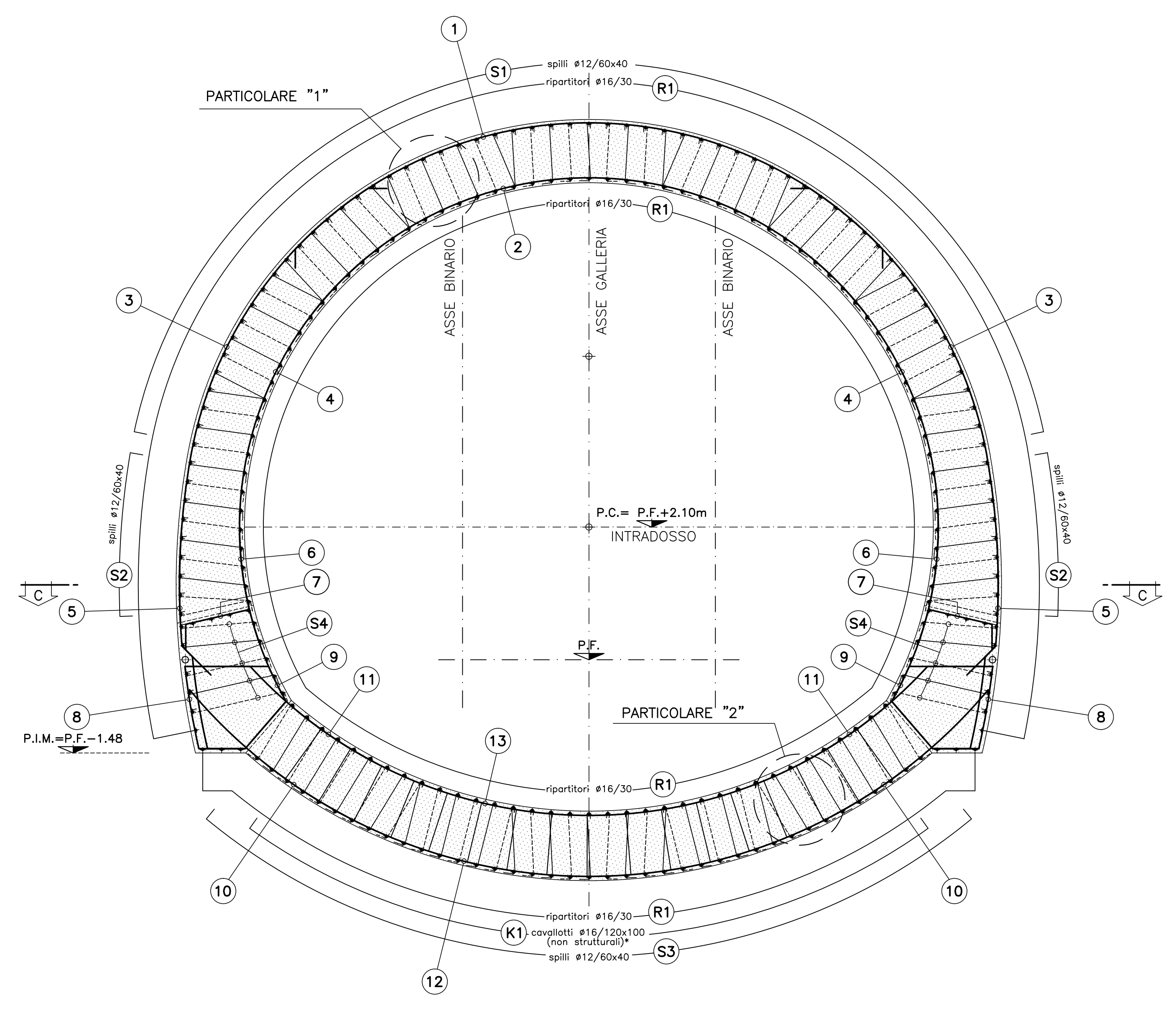
ESPLOSO
