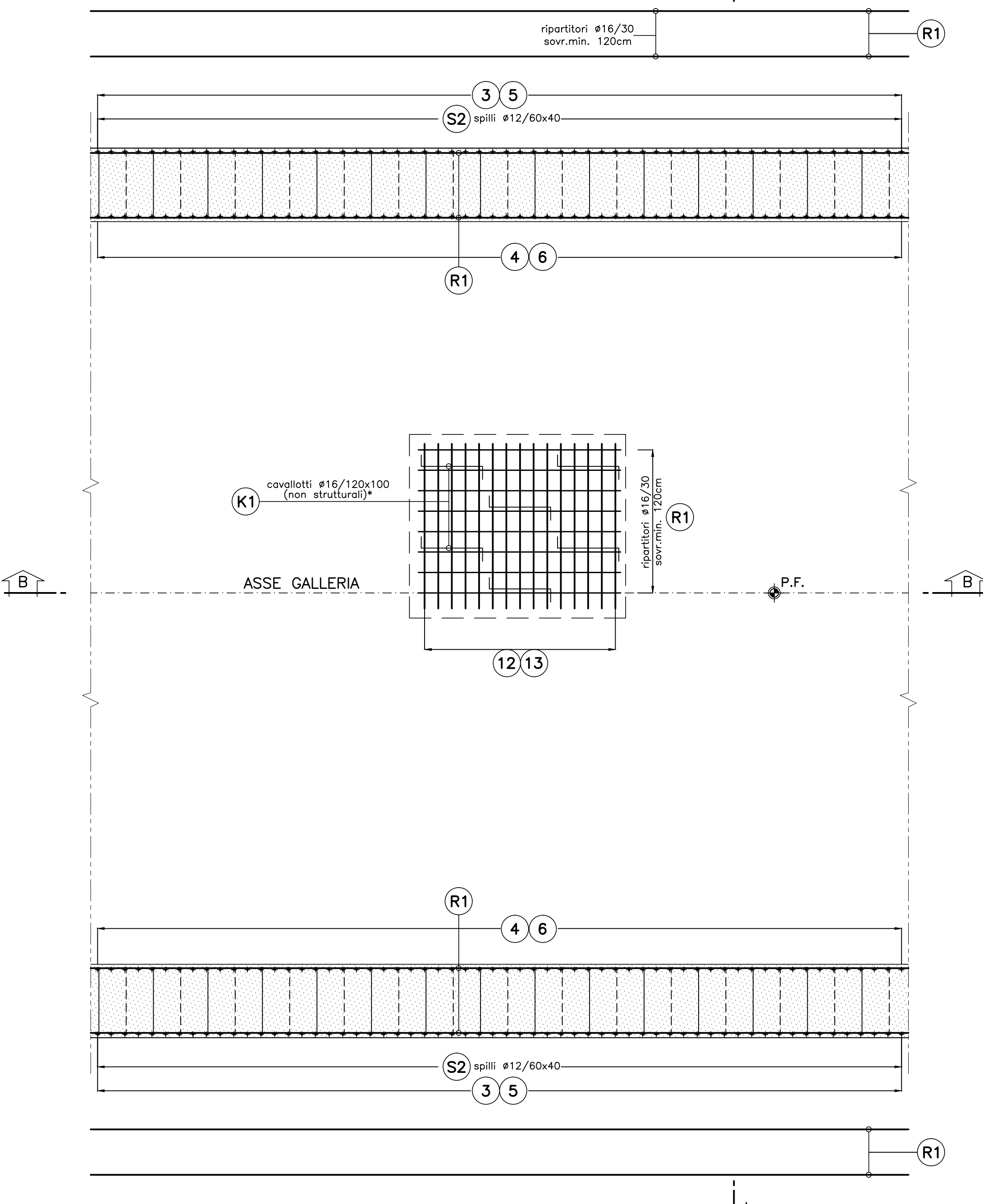
SEZIONE C-C SCALA 1:50 PIANTA
