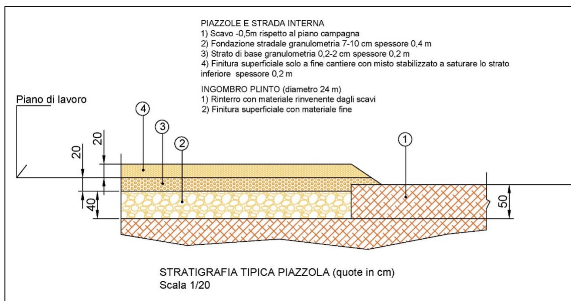
Fig.3 - Stratigrafia tipica di progetto area piazzole e strade
