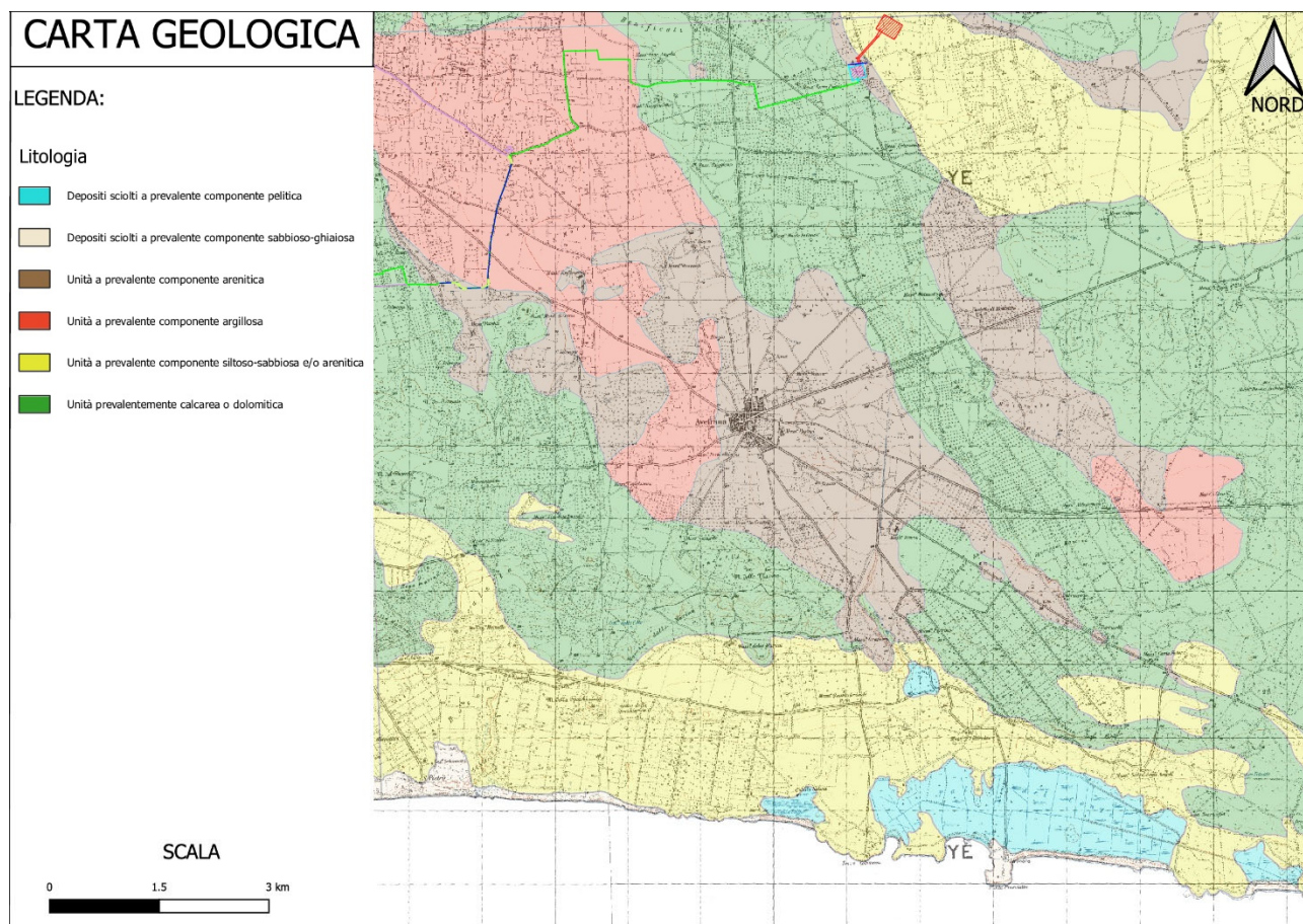
Fig.2 Inquadramento geologico dell'area d'intervento relativa all'impianto di connessione alla RTN.
