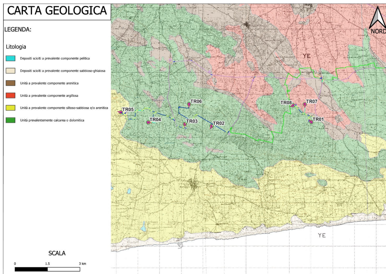
Fig.2 Inquadramento geologico dell'area d'intervento relativa all'impianto eolico.
