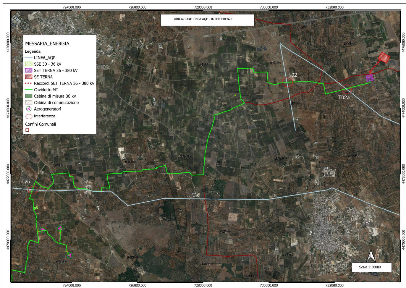
Fig. 1 Inquadramento linea MT 36 kV interferente le linee AQP – Cerchio rosso interferenza linea AQP
