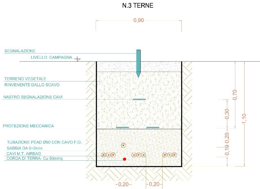
Tipo cavidotto interrato MT
