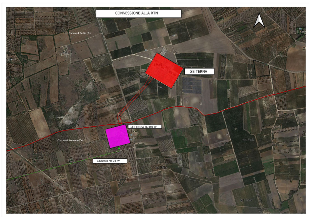
Ubicazione della SET TERNA 36/380 kV – In rosso la Stazione elettrica nel Comune di Erchie (Br)
