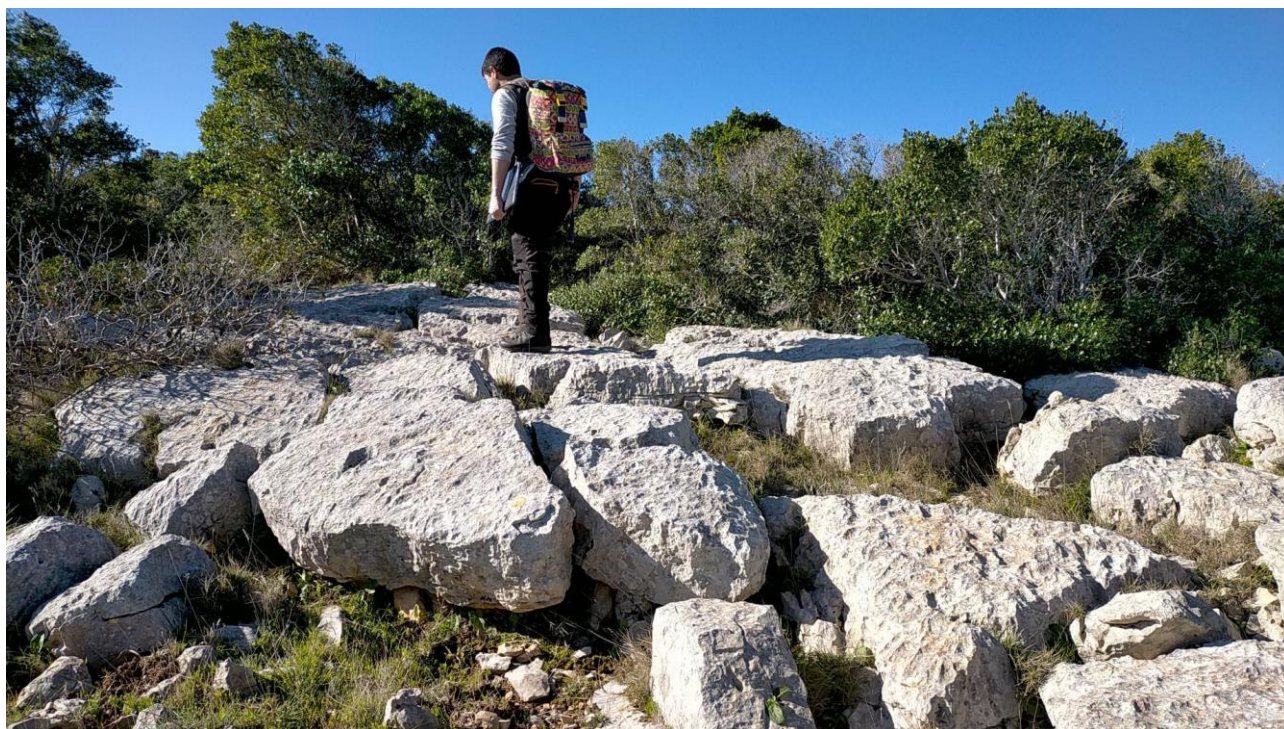
Figura 18 Fratturazione in blocchi alla scala dell'affioramento. (Formazione di Monte Nurra)
