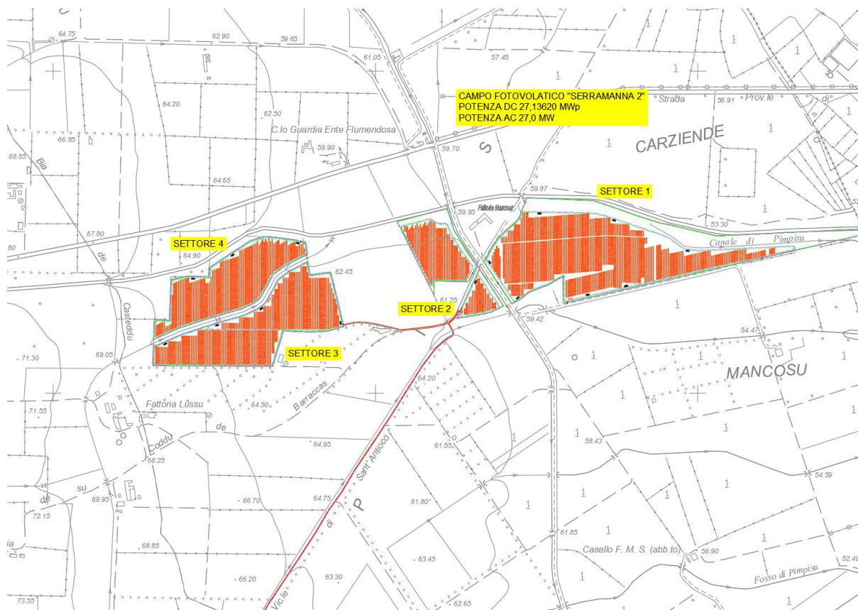
Fig. 2 Area d’impianto con individuazione settori
