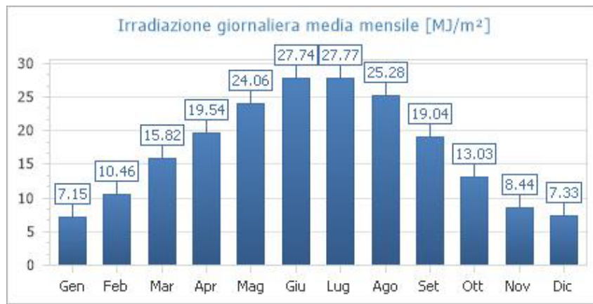
Fig. 1: Irradiazione giornaliera media mensile sul piano orizzontale [MJ/m²]- Fonte dati: UNI 10349:2016 - Stazione di rilevazione: Samassi
