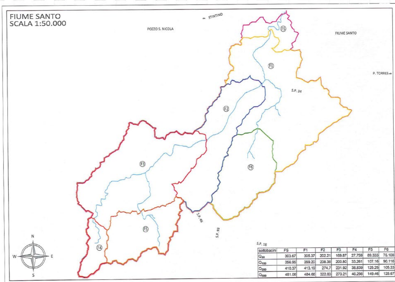
Figura 34 – Sottobacini del Bacino idrografico di Fiume Santo
