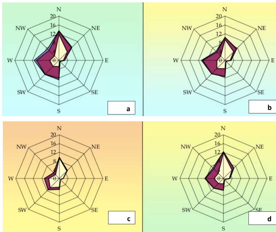
Figura 25 Ventosità media per inverno (a), primavera (b), estate (c), e autunno (d) durante il periodo 1971-2000 registrate nella stazione meteorologica di Fertilia.
