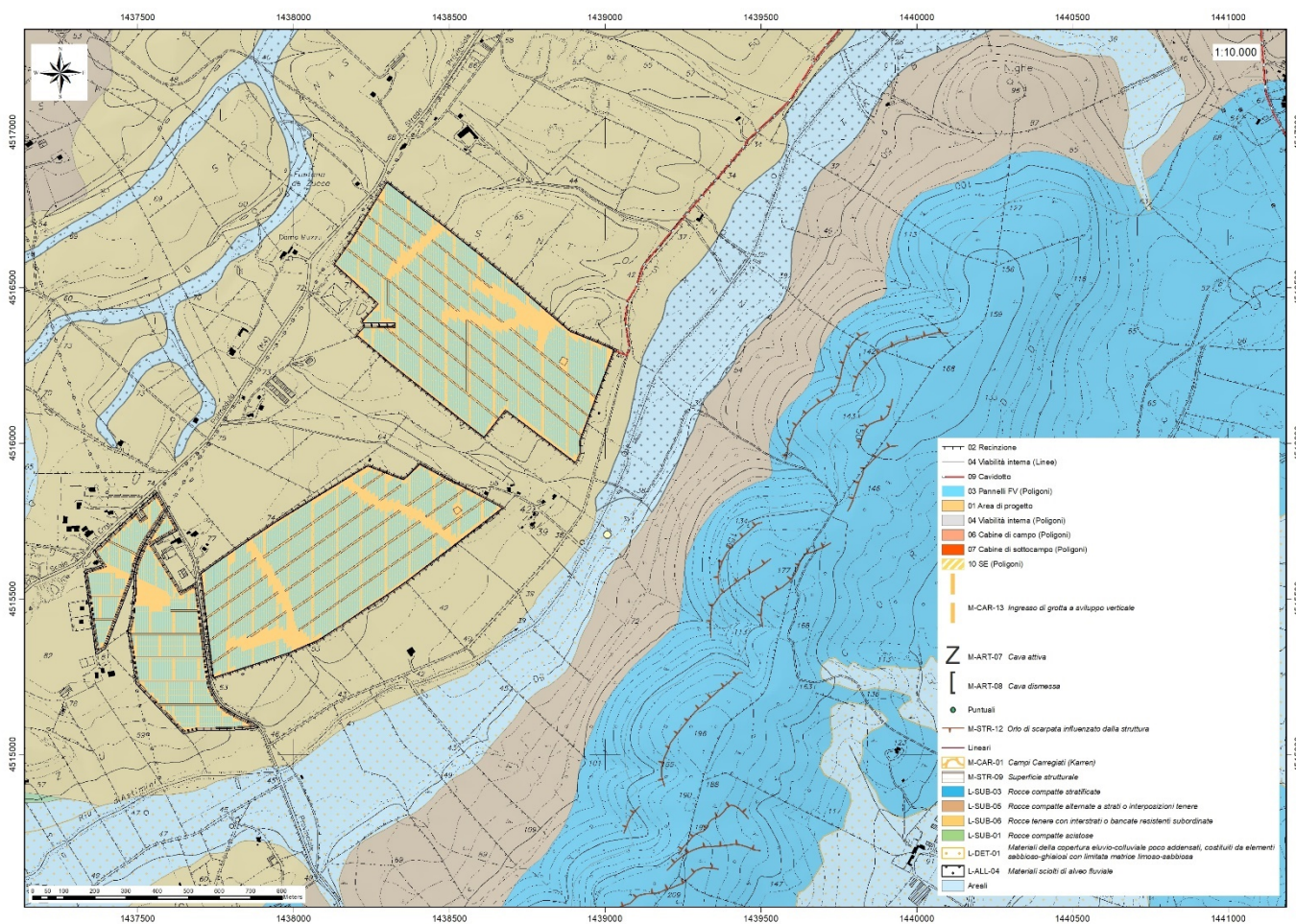
Figura 18 Carta geomorfologica dell'area di progetto
