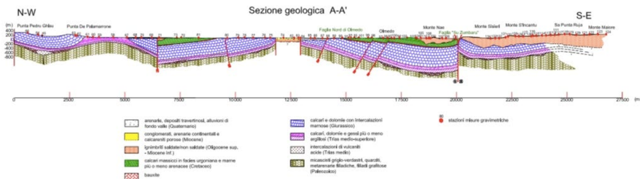
Figura 8 Sezione geologica rappresentativa dell'area vasta (tratto da Ghiglieri et al 2006; 2009a)
