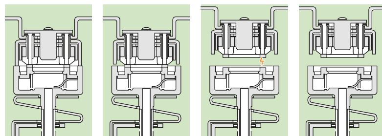
Contatti chiusi
