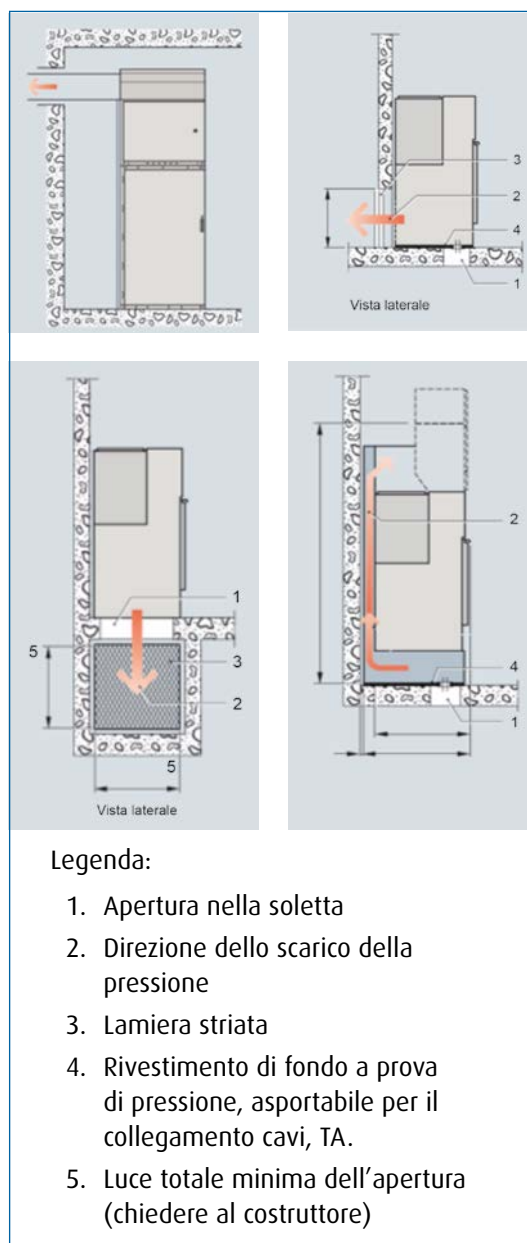
Figura 5.8: Sistema di canalizzazione della pressione verso l'esterno (1° immagine) o verso il retro (2° immagine) o verso il basso (3° immagine) o l'alto (4° immagine)
