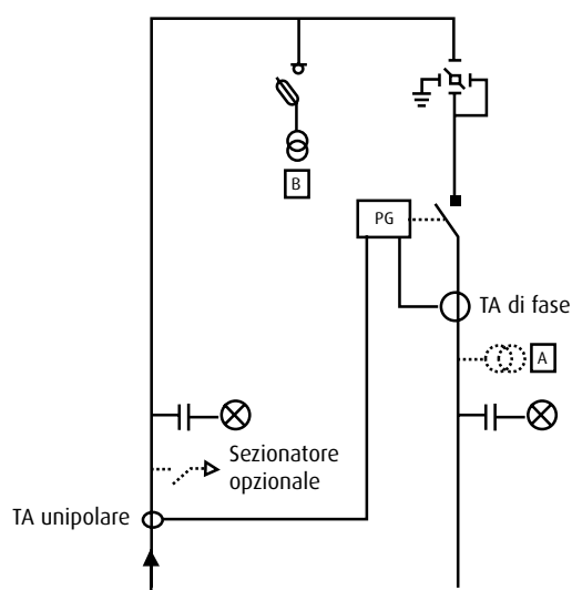
Figura 5.4: Schema di impianto di utenza per la connessione: caso generale
