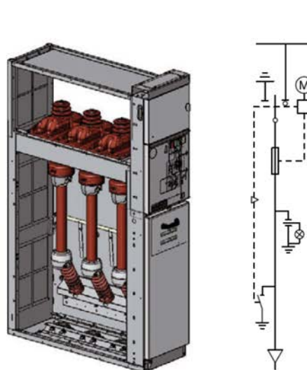
Figura 5.2: UF Interruttore di manovra-sezionatore combinato con fusibile
