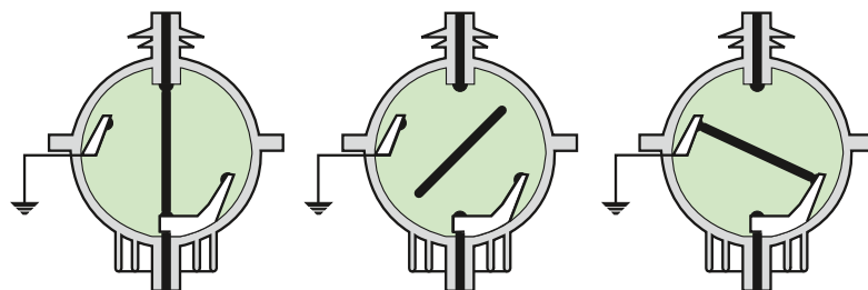
apparecchio chiuso
