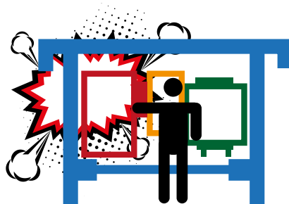
Figura 1.19: Classificazione arco interno IAC-A
