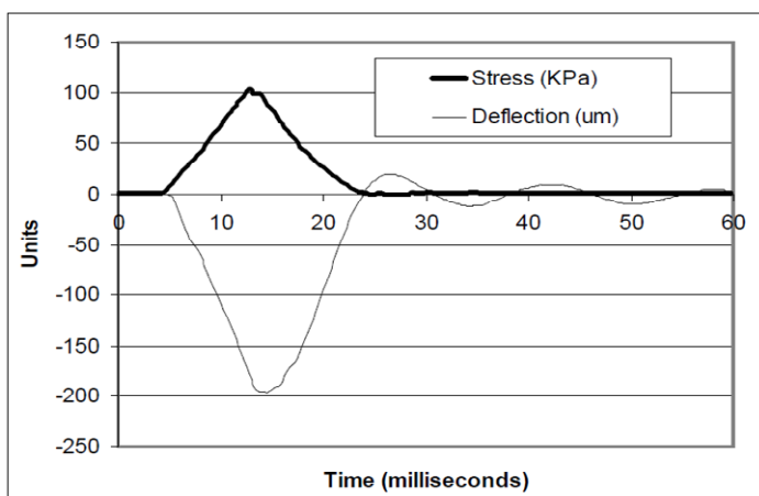
Tipico diagramma risultante da una prova LWD su stabilizzato granulometrico di buone caratteristiche (la pressione è risultata in questo caso superiore a 70 kPa)
