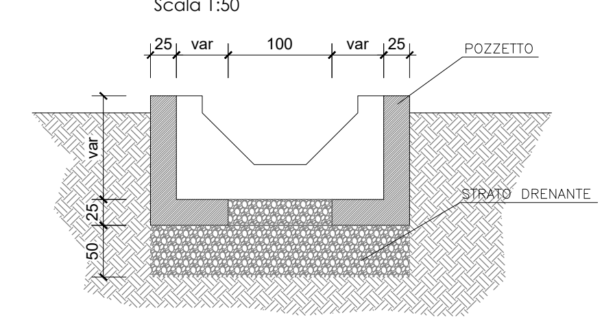
PARTICOLARE POZZETTO DISPERDENTE
