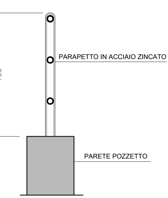
TIPOLOGICO PARAPETTO scala 1:20
