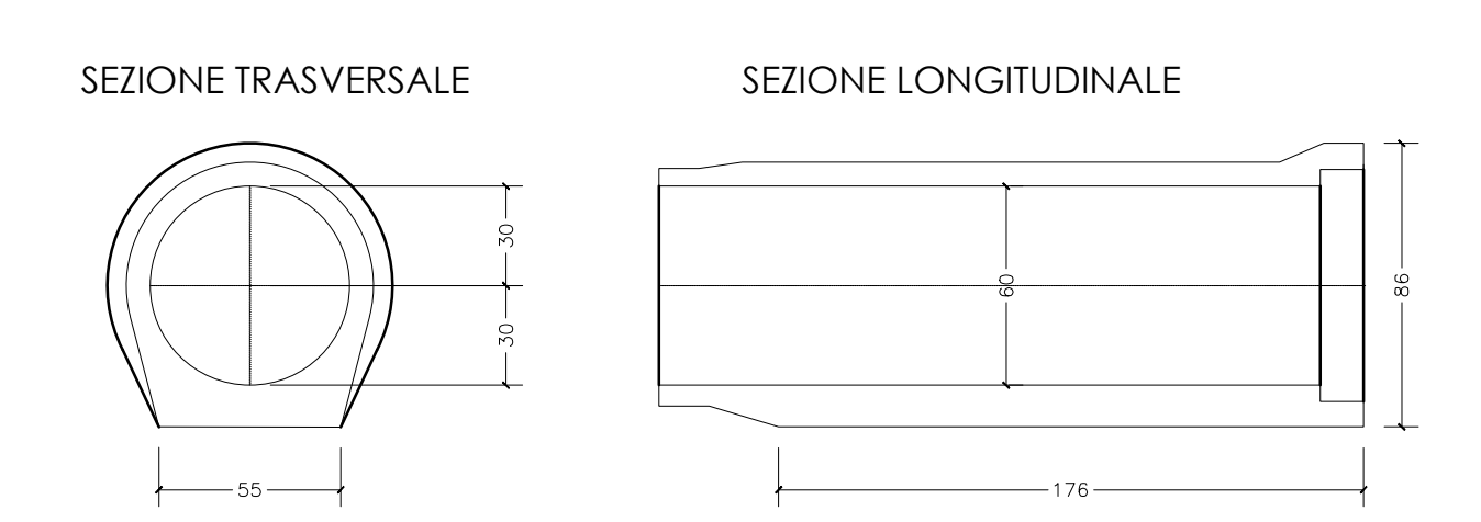
TUBAZIONE ADOTTATA (Ø60): CASSERATURA
