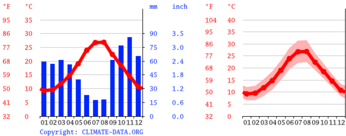
Figure 9 | Grafico della Temperatura e del clima, del Comune di Erchie ( https://it.climate-data.org/europa/italia/puglia/erchie-990985/#climate-graph ).
