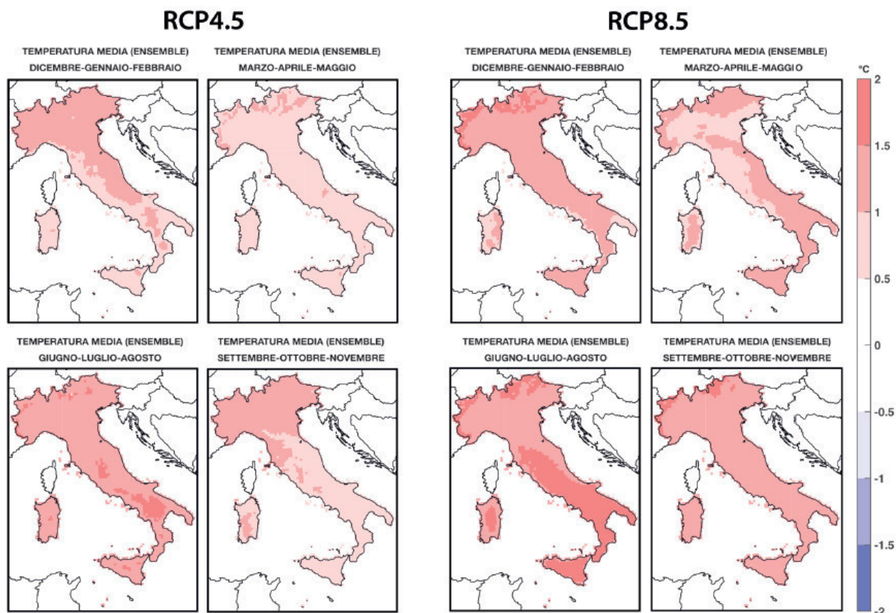
Figure 11 | Mappe di variazione della temperatura a due metri su scala stagionale sull'Italia dall'ensemble EURO-CORDEX secondo gli scenari RCP4.5 e RCP8.5 per il periodo 2021-2050 rispetto al periodo di riferimento 1981-2010 (CMCC, 2019)
