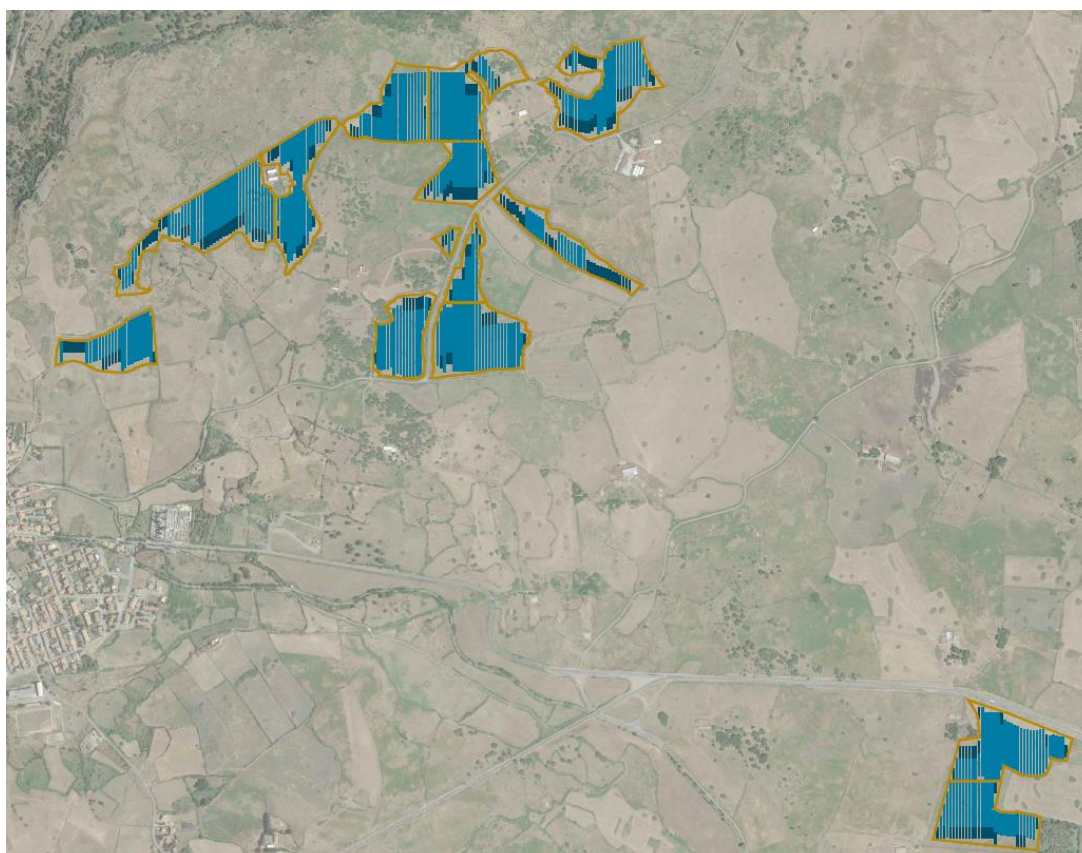
FIGURA 1: LAYOUT D' IMPIANTO
