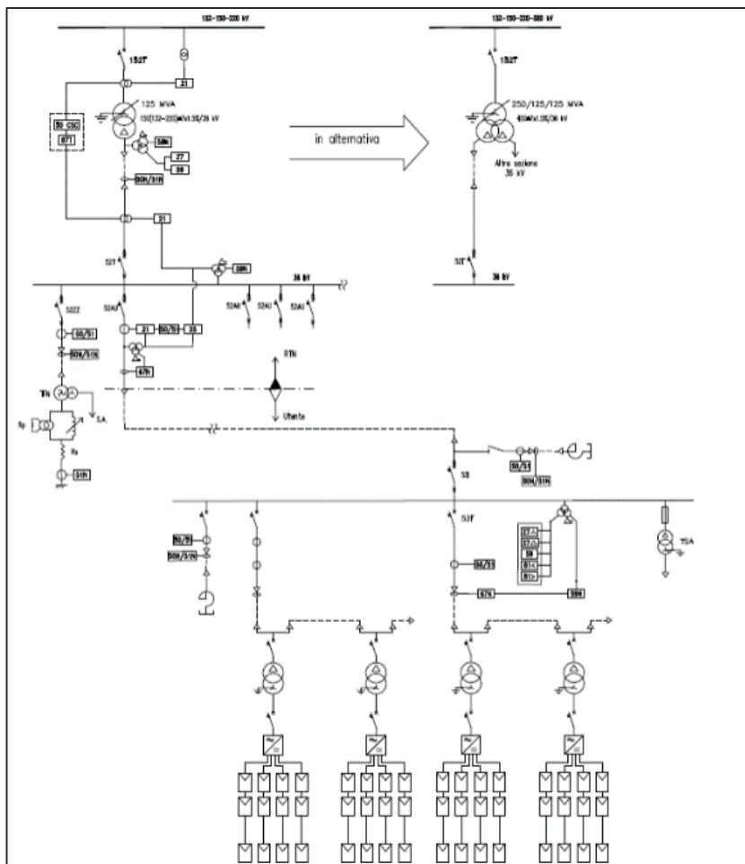
FIGURA 9: ASSETTO DELLE PROTEZIONI CONTRO I GUASTI E LE PERTURBAZIONI NELLA RETE DI UNA CENTRALE FOTOVOLTAICA (ESTRATTO DA ALLEGATO A.68 DEL 19 MAGGIO 2022)
