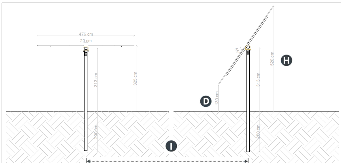
FIGURA 3: DEFINIZIONE DELLE DIMENSIONI DEI TRACKER
