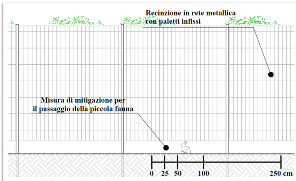
FIGURA 9: RECINZIONE TIPO
