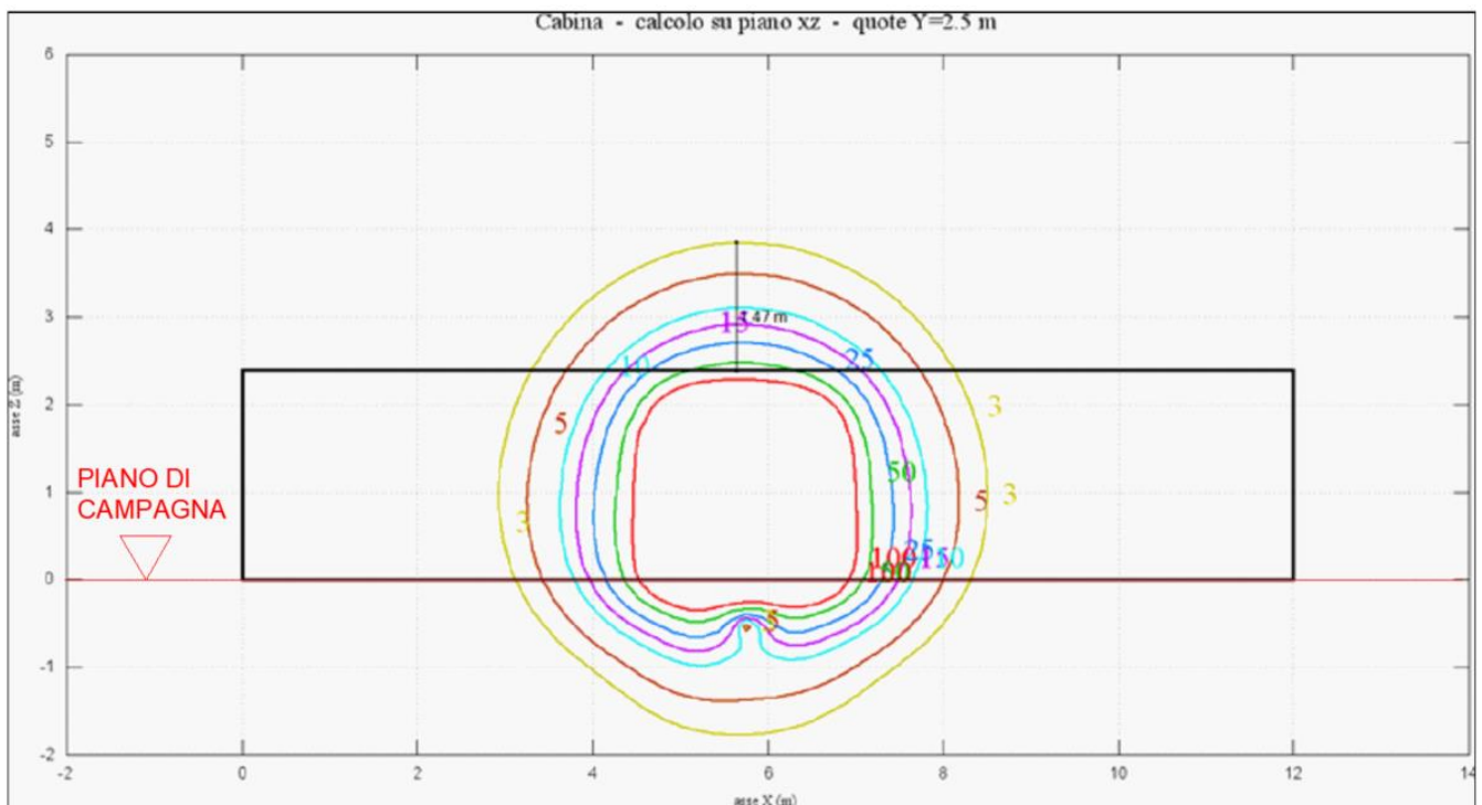
FIGURA 5: CURVE ISOINDUZIONE CABINA AT DI CONSEGNA (PROSPETTO FRONTALE)
