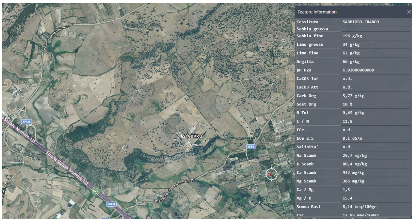
Figura 29: Caratterizzazione ecopedologica
