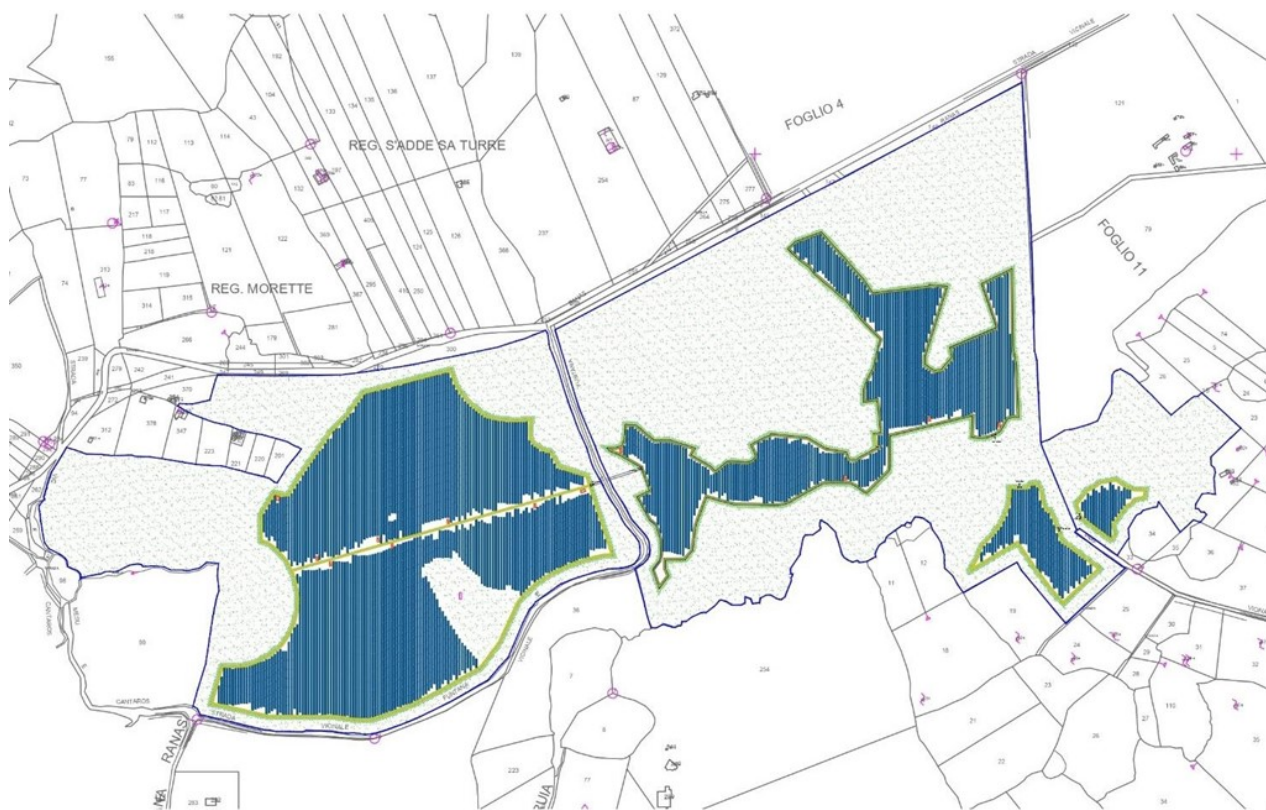
Figura 6: Vista d'insieme del campo agrivoltaico su base catastale
