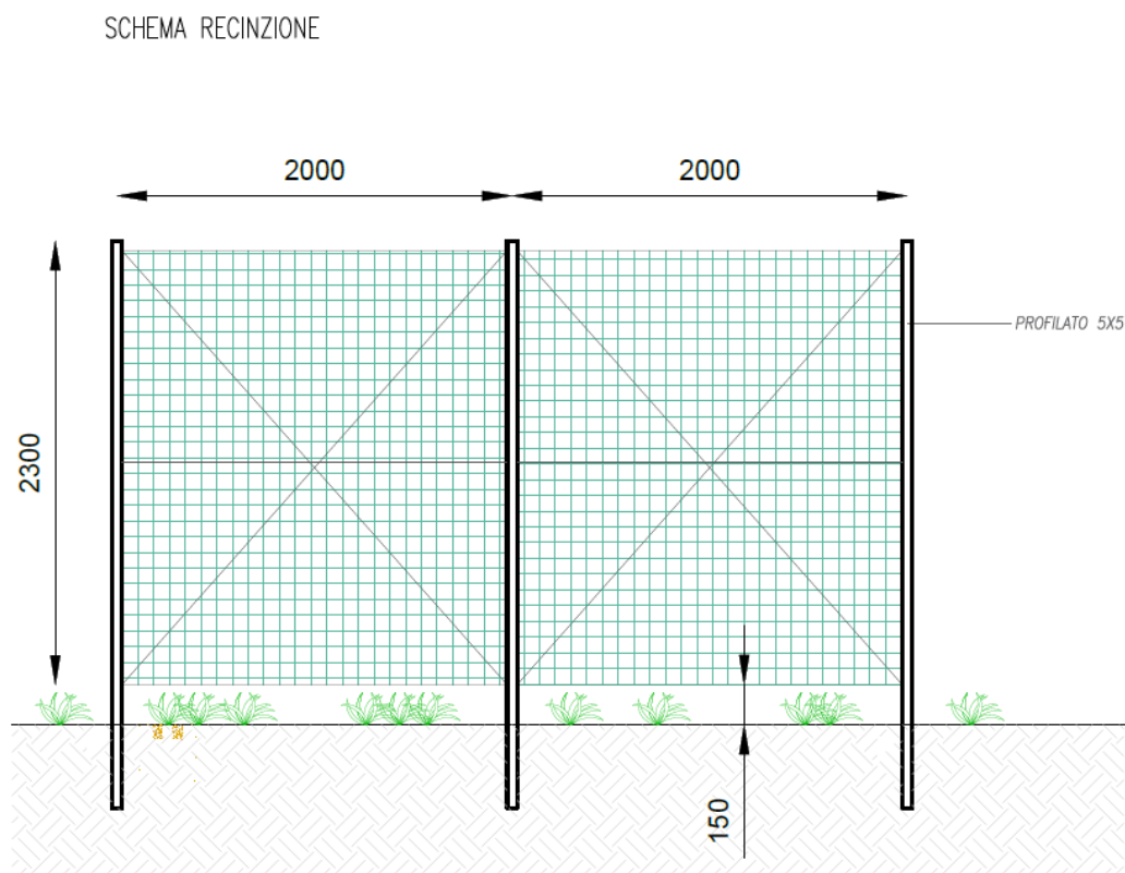
Figura 7: Particolare opera di recinzione
