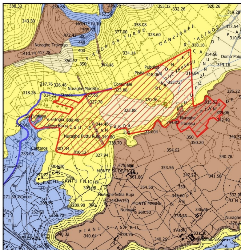
CARTA LITOLOGICA
