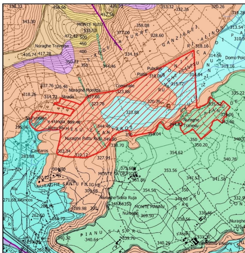
CARTA GEOLOGICA
