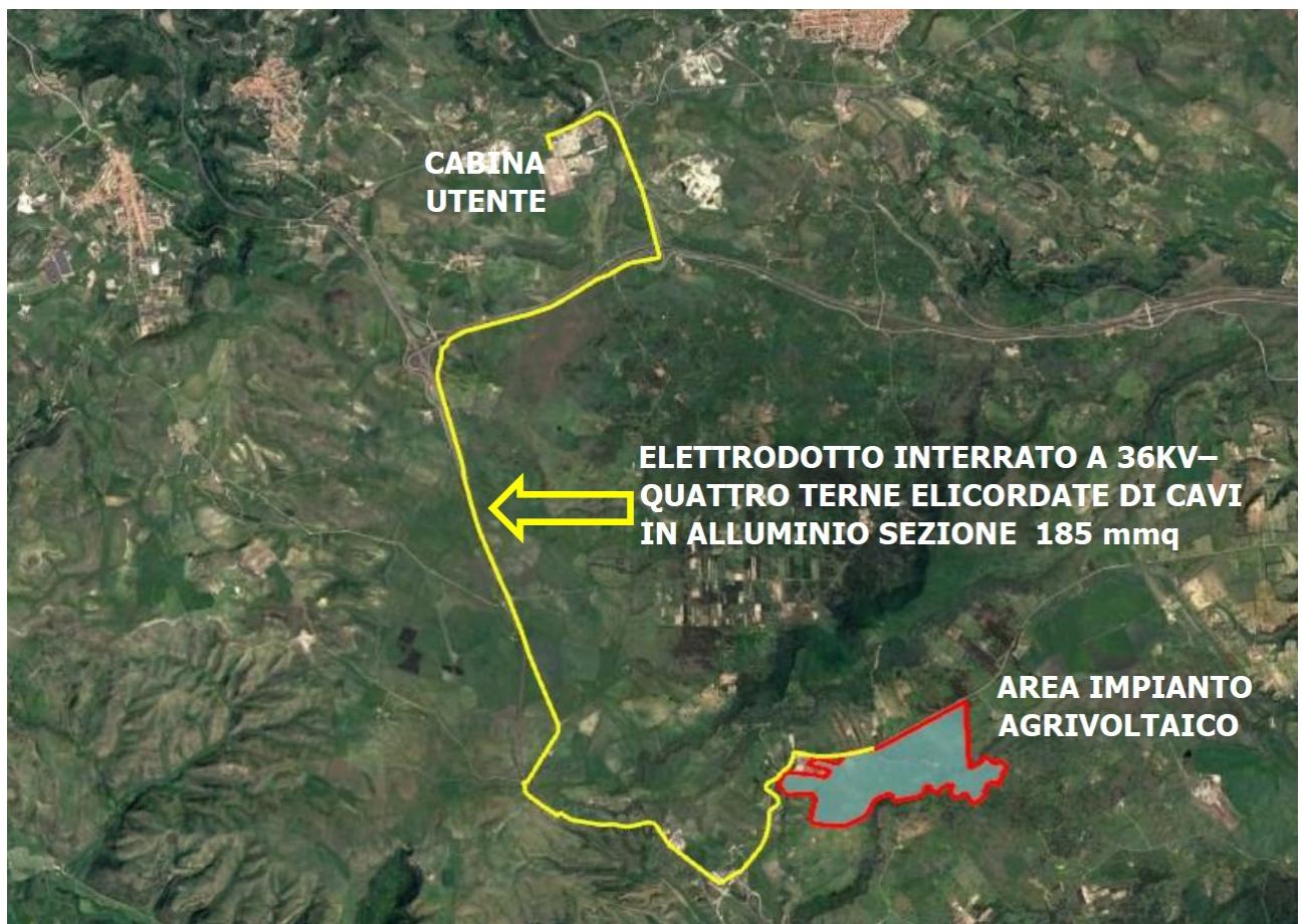
Figura 3. Vista d'insieme dell'impianto e delle opere di connessione su base ortofoto
