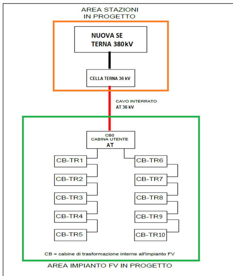
FIGURA 5: SCHEMA A BLOCCHI IMPIANTO
