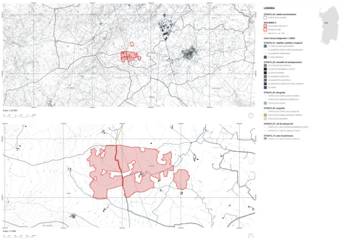
FIGURA 1: INQUADRAMENTO TERRITORIALE SU CTR IN SCALA 1:25000 E 1:5000
