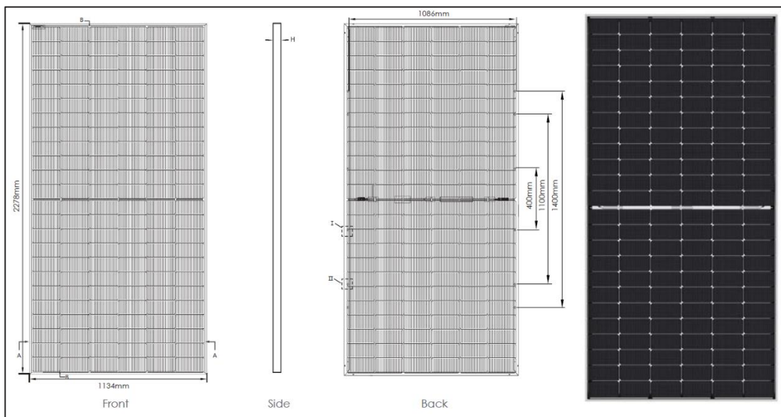
FIGURA 6: PANNELLO FV PARI A 570 WP CON DIMENSIONI 2278 x 1134 x 35 MM
