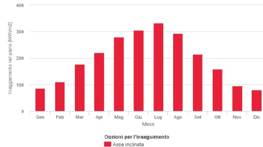
FIGURA 4: SULLA SINISTRA PRODUCIBILITÀ MEDIA MENSILE DEL SITO, SULLA DESTRA IRRAGGIAMENTO AL METRO QUADRO
