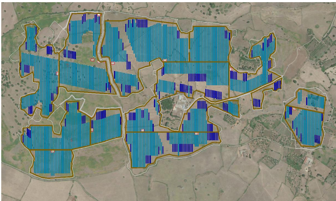
FIGURA 4: LAYOUT D' IMPIANTO
