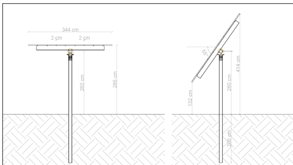
FIGURA 2: TRACKER TIPO AD ASSE VARIABILE
