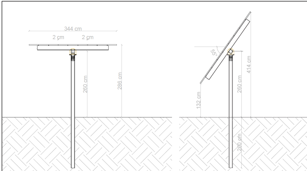
FIGURA 1: TRACKER SOLARE TIPO
