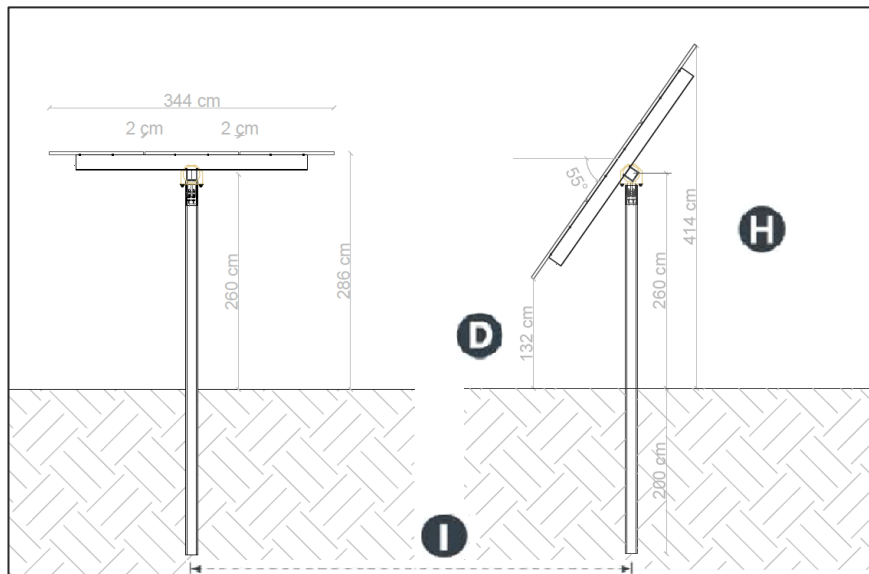
FIGURA 3: DEFINIZIONE DELLE DIMENSIONI DEI TRACKER
