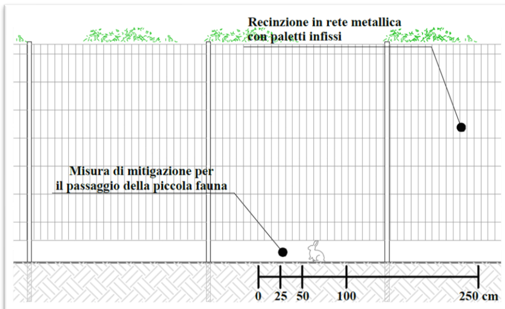
FIGURA 8: RECINZIONE TIPO
