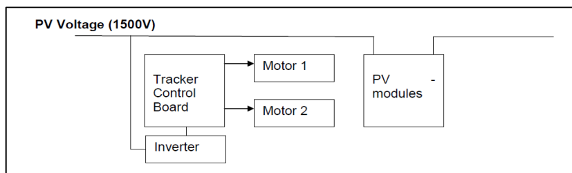
FIGURA 5: ALIMENTAZIONE DEL MOTORE DEI TRACKER DIRETTAMENTE DAL CAMPO FV
