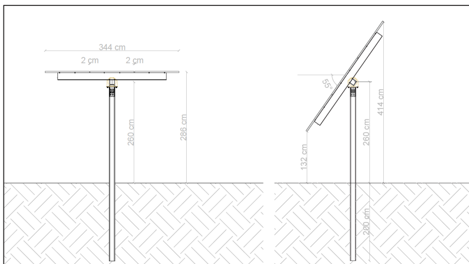
FIGURA 2: SCHEMA TIPO TRACKER AD ASSE VARIABILE
