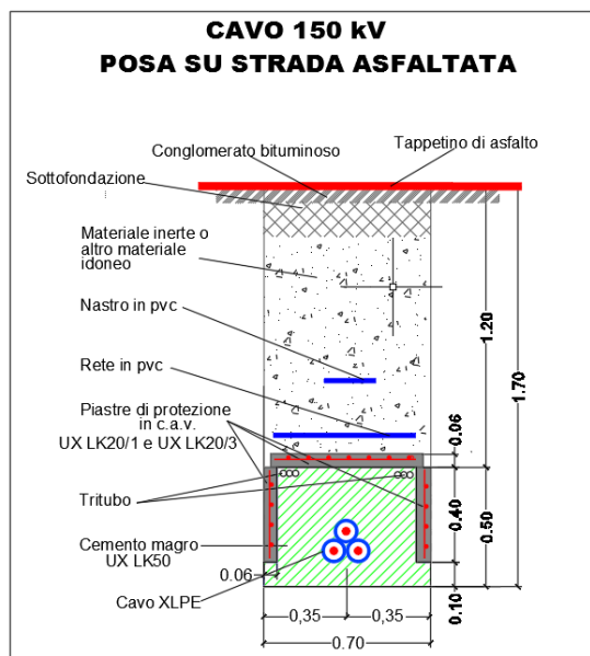
Figura 2: Posa cavo 150 kV "SE 30/150 kV – SE "RTN Ittiri"
