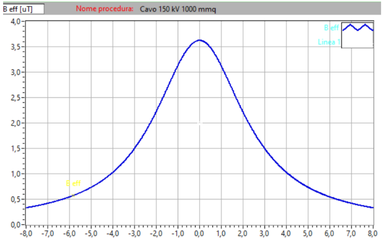
Fig. 3 Profilo laterale induzione magnetica (B) sezione tipo con indicazione della DPA - V=150 kV I = 910 A
