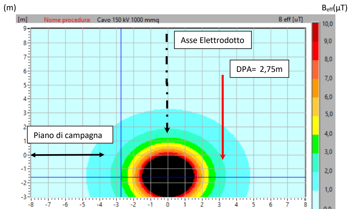
Fig. 4 Mappa verticale induzione magnetica (B) sezione tipo con indicazione della DPA - V=150 kV I = 910 A
