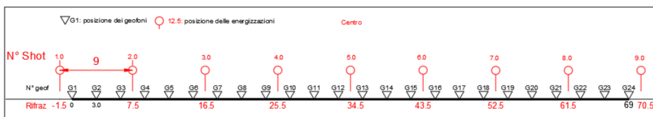
Figura 20 Stendimento di sismica a rifrazione in onde P con 24 geofoni, interdistanza di 3,0 m, lunghezza complessiva 69,0 m
