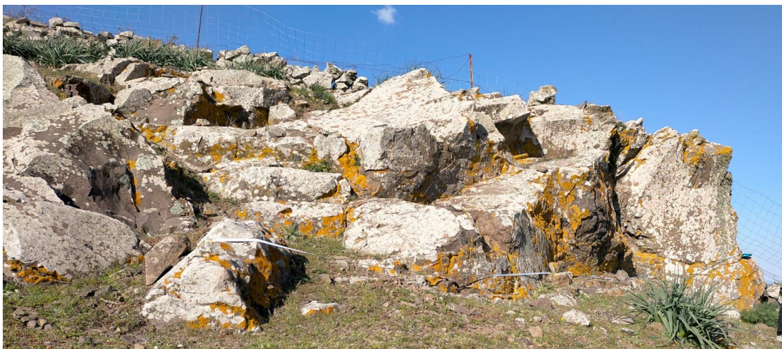
Figura 8 Affioramento dell'Unità di Nuraghe Vittore
