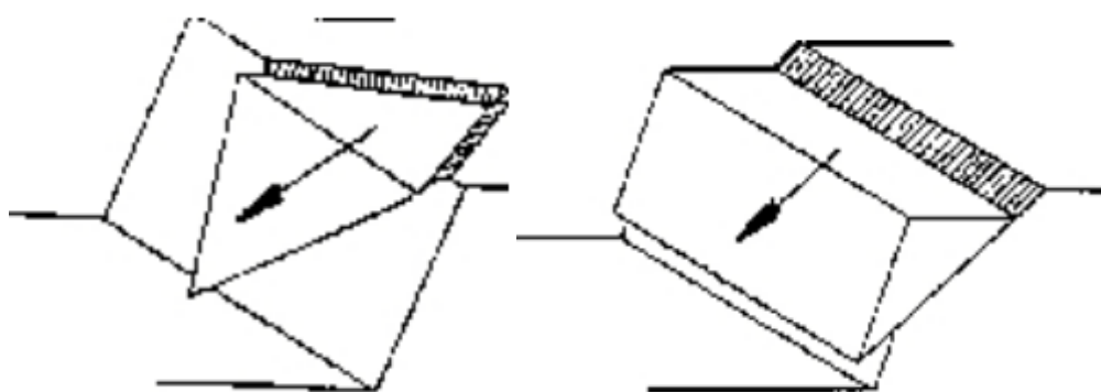
Figura 11 Tipologie di scivolamento di blocchi rocciosi lungo piani di fratturazione
