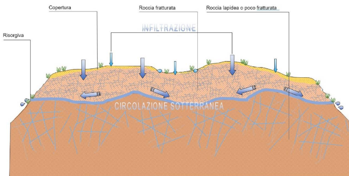
Figura 15 Schema esemplificativo, non in scala, dei processi di infiltrazione e deflusso sotterraneo
