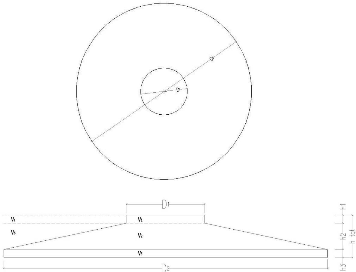
Figure 2 - Caratteristiche geometriche della fondazione
