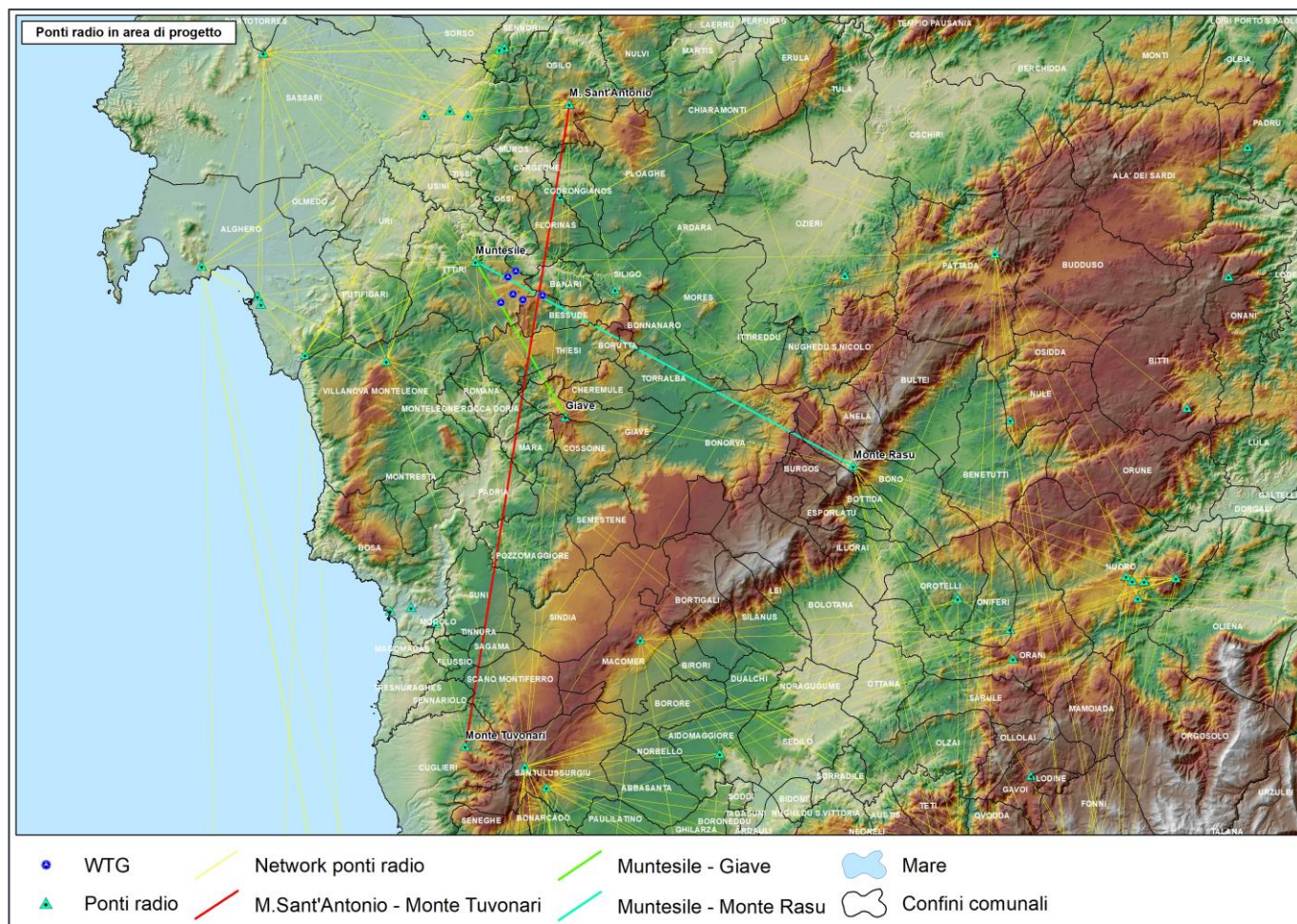
Figura 6 - tratte ponti radio nell'area vasta.
