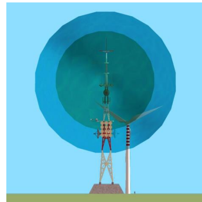
Figura 4 - Interferenza di una WTG con le zone di Fresnel
