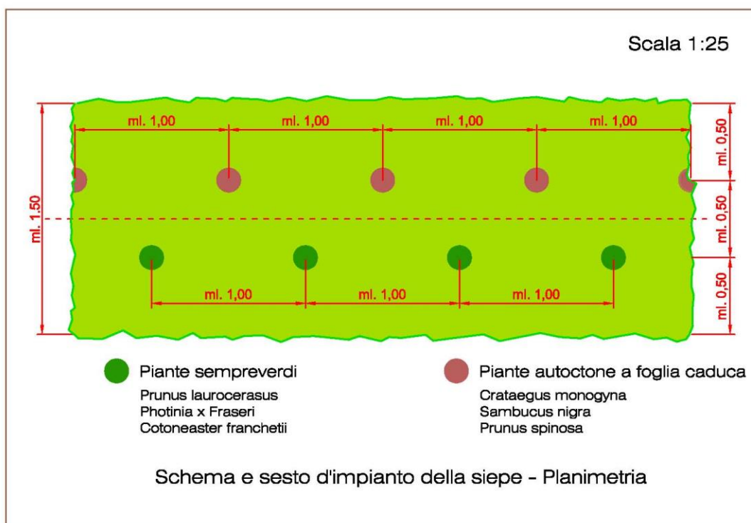
Figura 8: Schema di siepe – Planimetria
