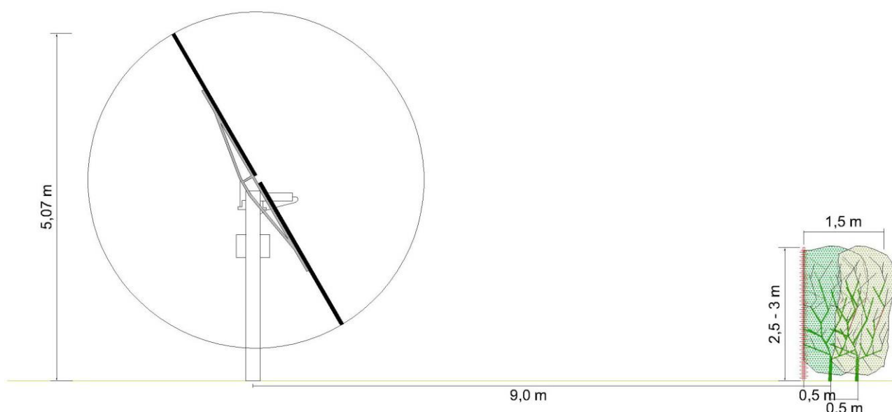
Figura 7: Schema di siepe – Sezione trasversale
