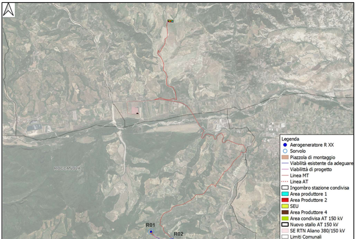
Figura 6.2: Soluzione di connessione alla RTN in corrispondenza della SSE RTN Terna 380/150 kV Aliano
