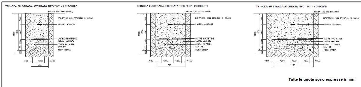
Figura 6.3.3.4: Sezioni tipiche delle trincee cavidotto su strada sterrata
