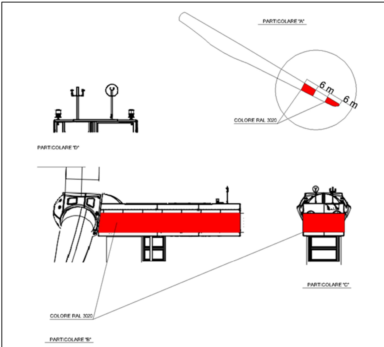
Figura 6.1.2: Particolari aerogeneratore SG170 – 6.2 MW di cui alla Figura 6.1.1
