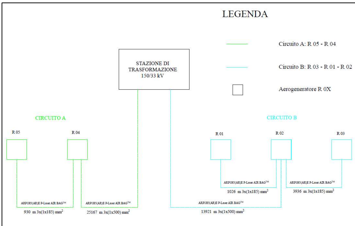
Figura 6.3.3.1: Schema a blocchi del Parco Eolico Roccanova
