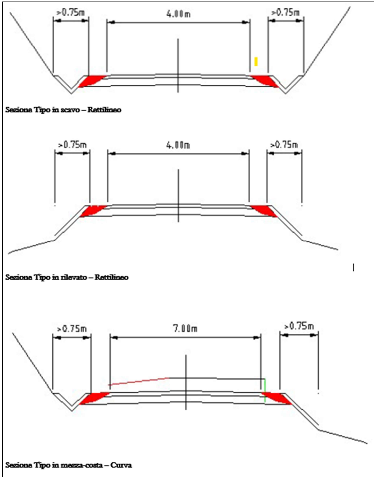
Figura 6.2.1: Sezioni tipo viabilità parco eolico
