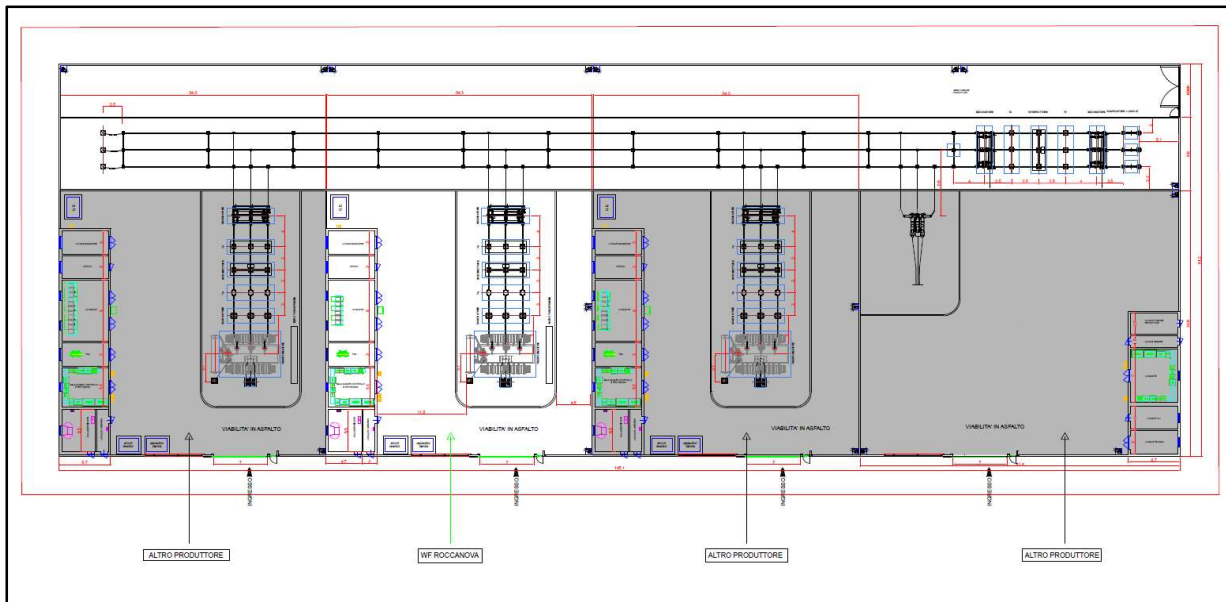
Figura 6.3.2.2: Layout della Stazione Elettrica Utente 150/33 kV (SEU)
