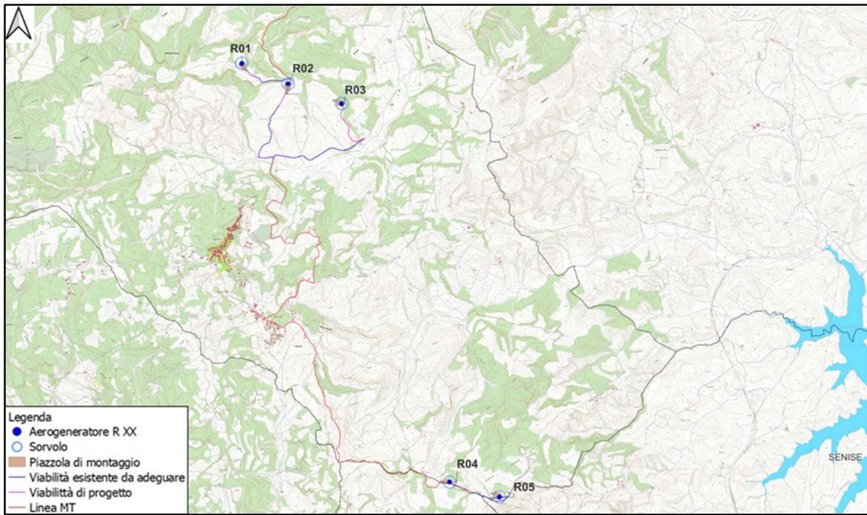
Figura 6.5: Parco Eolico Roccanova su CRT
