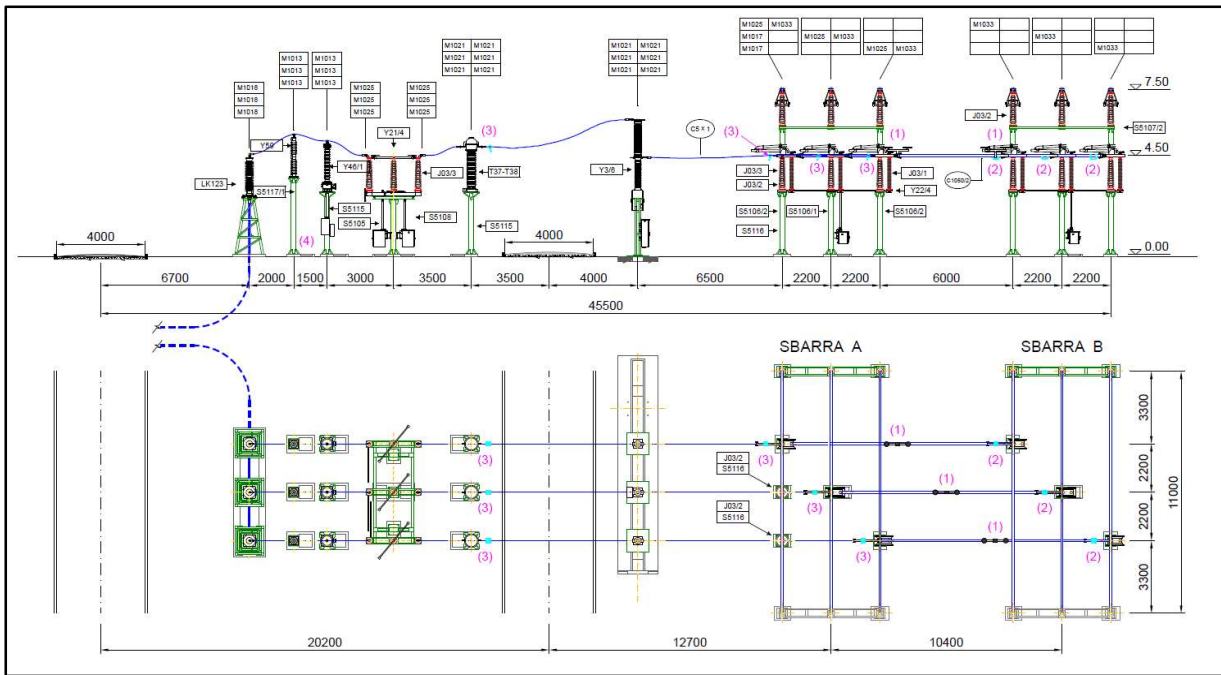
Figura 6.3.6.3: Planimetria e sezione elettromeccanica relativa alle apparecchiature dello stallo 150 kV nella stazione Terna
