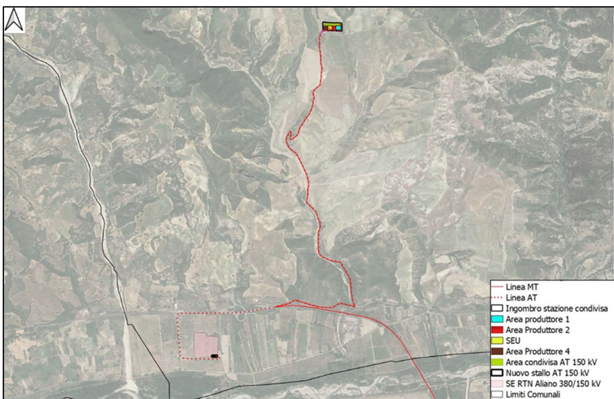
Figura 6.3.2.1: Localizzazione della SEU 150/33 kV e della SE RTN 380/150 kV di Aliano
