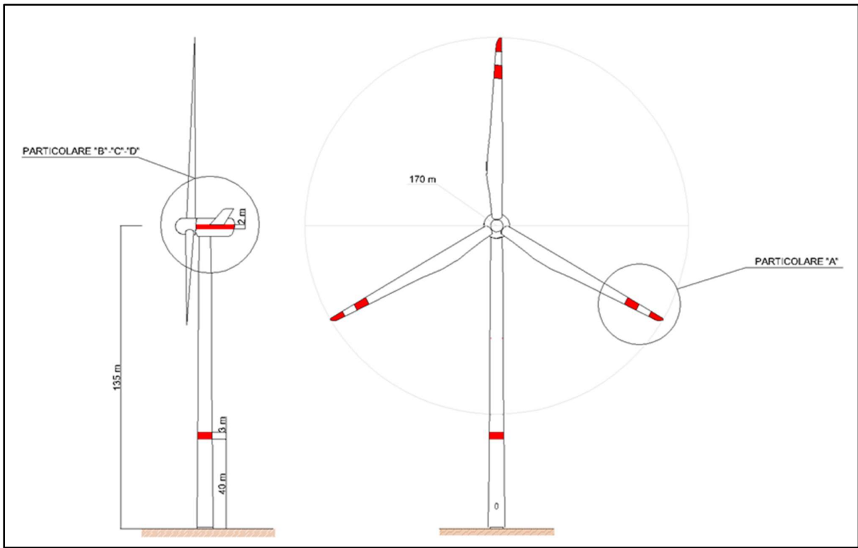
Figura 6.1.1: Profilo aerogeneratore SG170 – 6.2 MW
