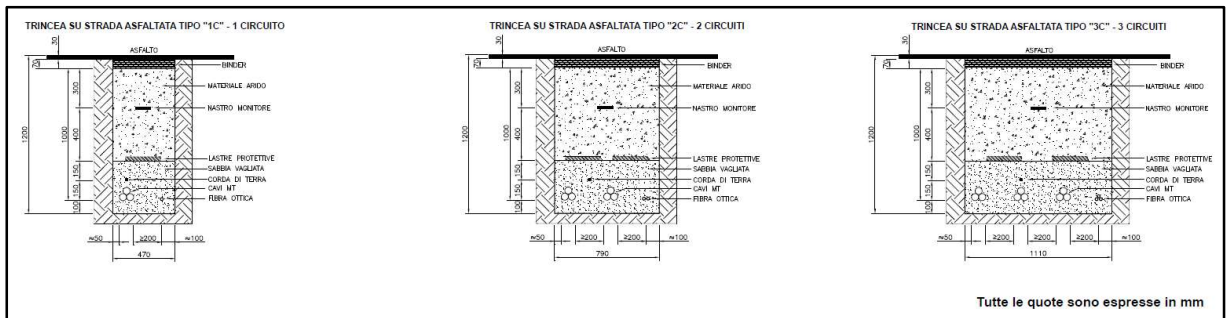
Figura 6.3.3.5: Sezioni tipiche delle trincee cavidotto su strada asfaltata
