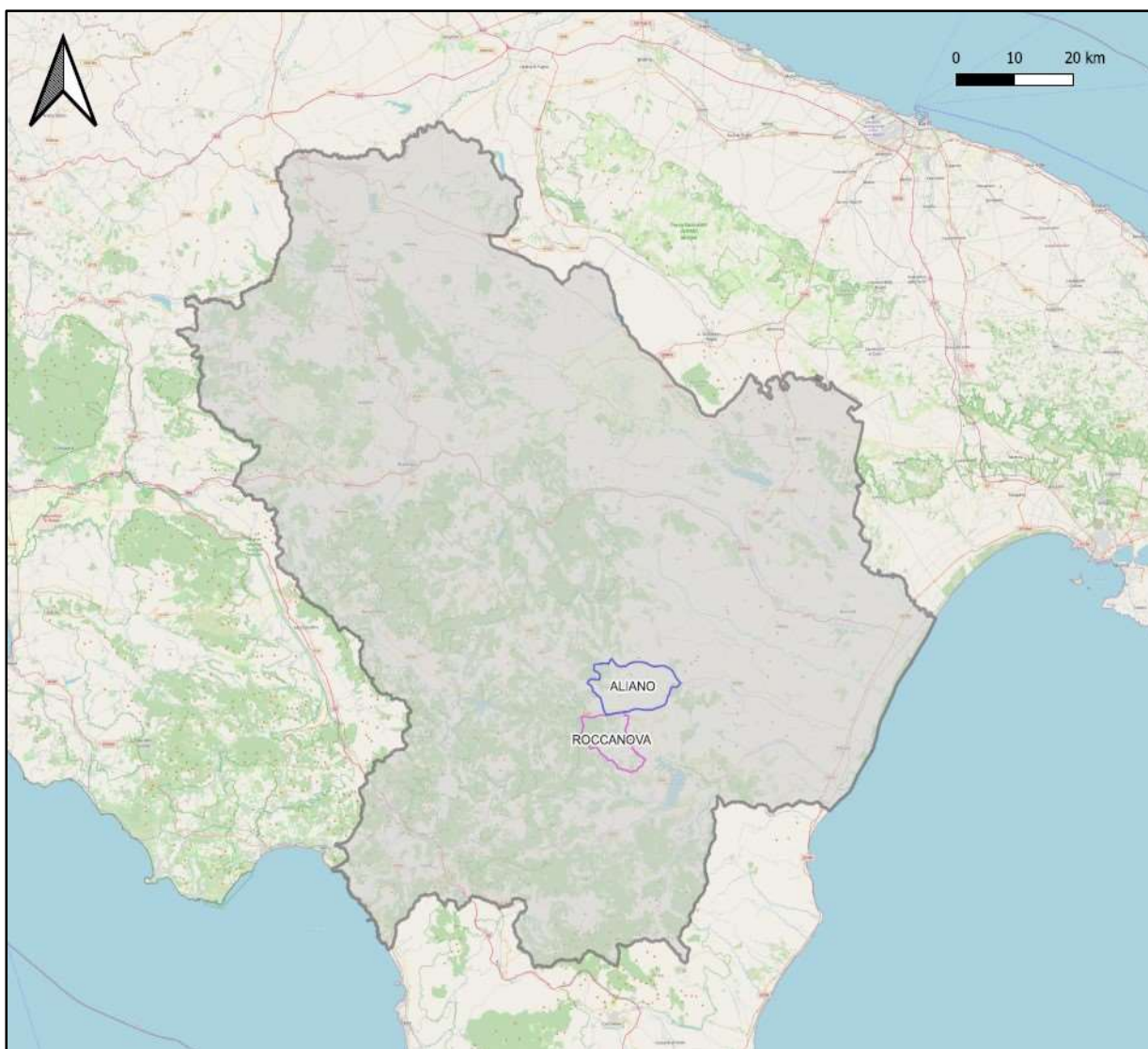
Figura 1.1: Localizzazione Impianto Eolico Roccanova
