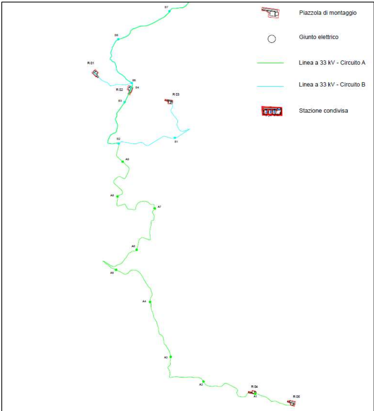
Figura 6.3.3.2: Planimetria di distribuzione linee MT di collegamento tra gli aerogeneratori
