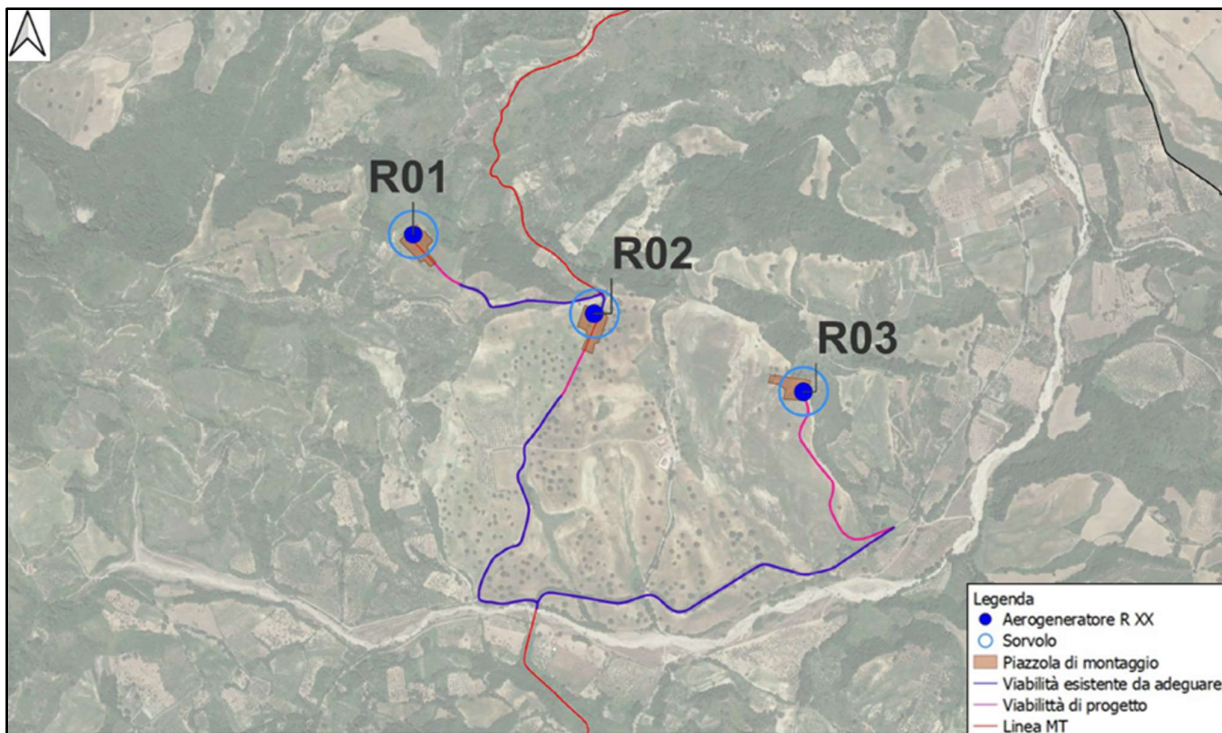
Figura 6.6: Parco Eolico Roccanova – Zona 1 su ortofoto
