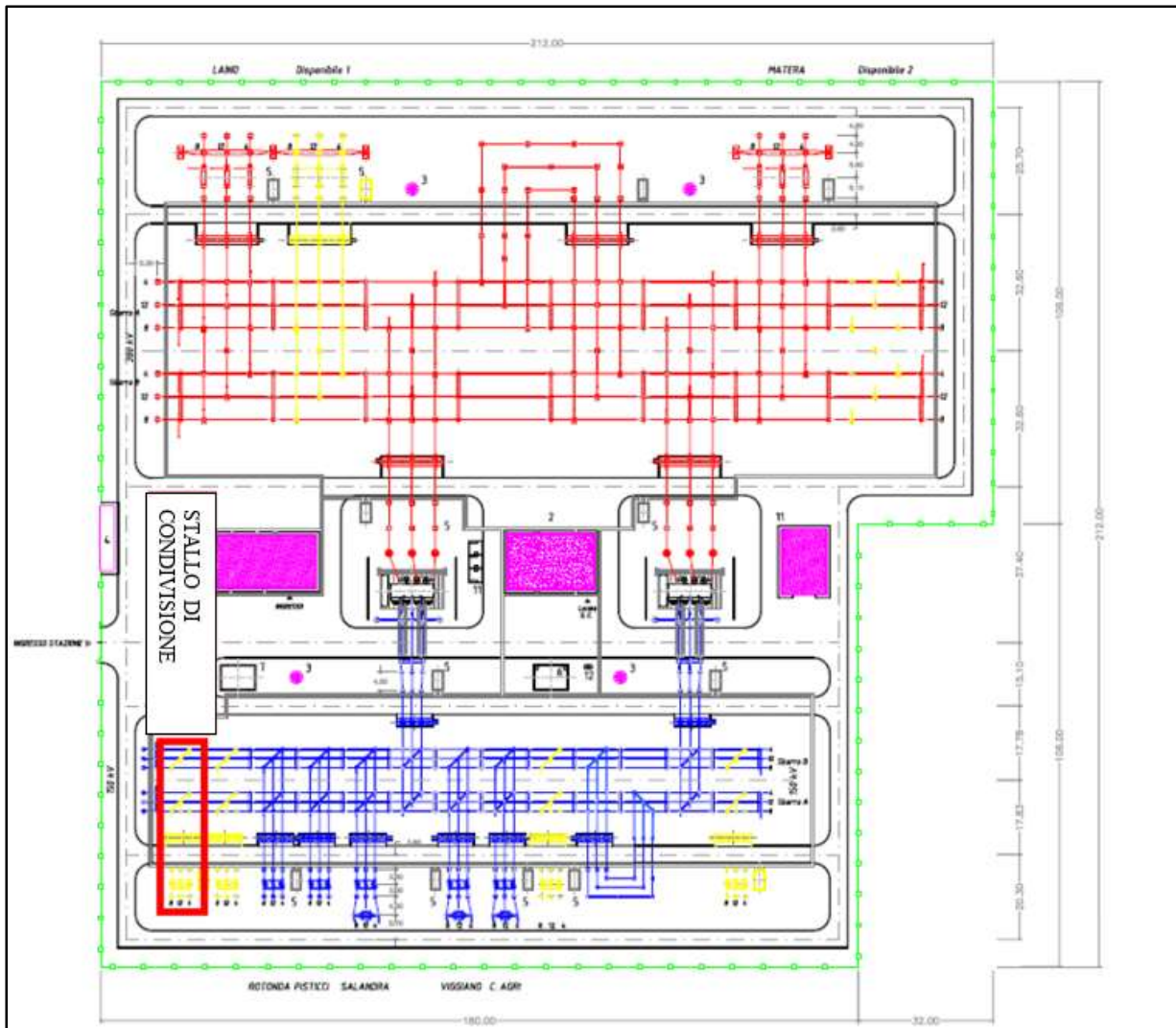
Figura 6.3.6.2: Planimetria della SE RTN a 380/150 kV con l'ubicazione dello stallo condiviso
