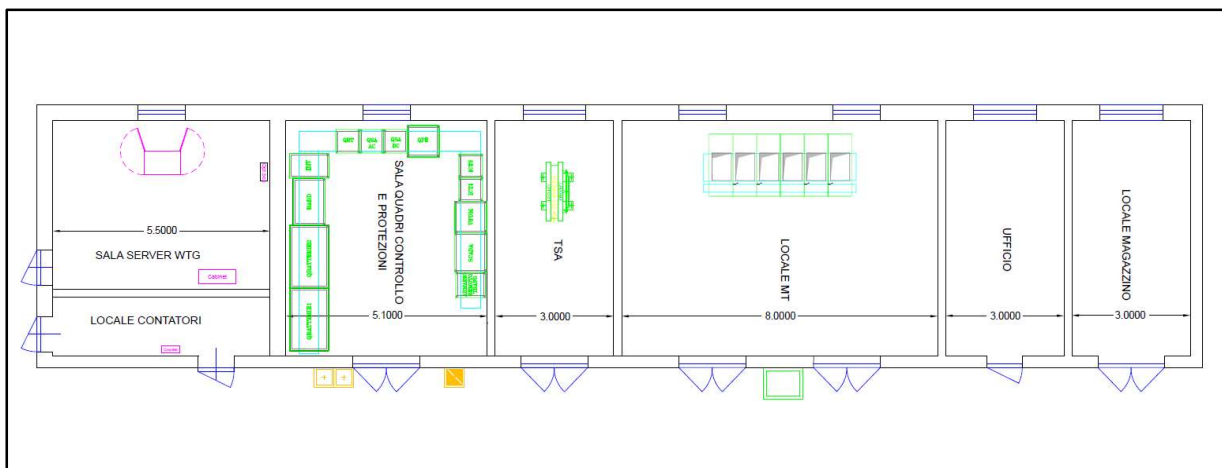
Figura 6.3.2.3: Pianta edificio di controllo SEU
