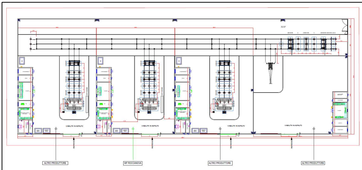
Figura 6.3.4.2: Planimetria elettromeccanica della sottostazione elettrica condivisa
