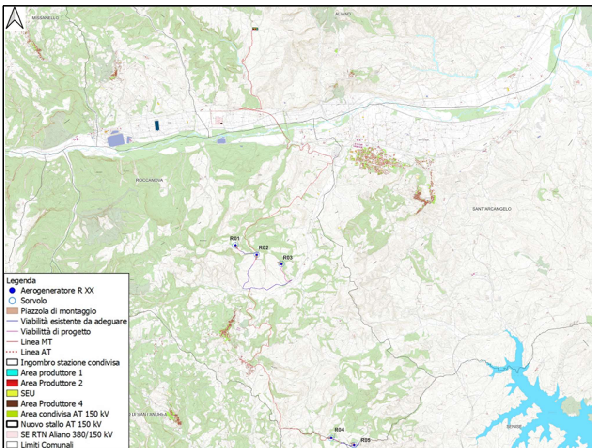
Figura 6.1: Inquadramento territoriale - Limiti amministrativi comuni interessati
