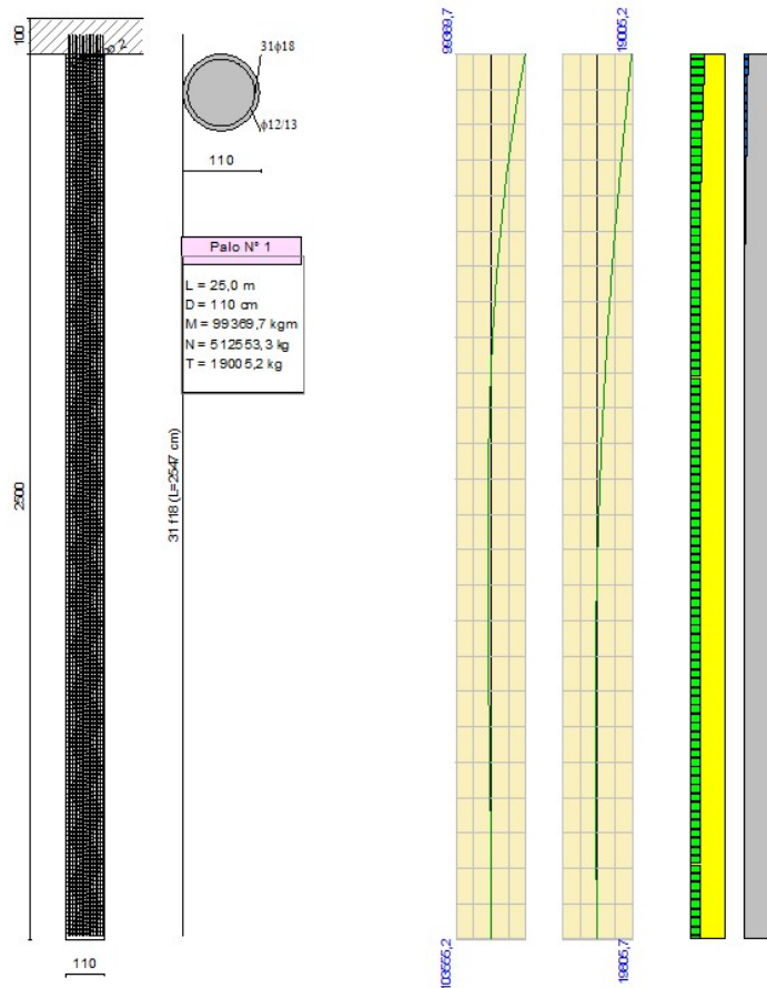
Figura 12.1.1: Diagrammi limite e di esercizio (unità di misura kgm per il momento flettente e kg per il taglio)
