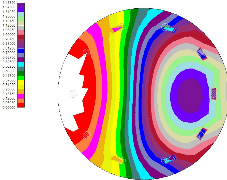
Figura 10.1.2 – Diagramma delle pressioni (unità di misura kg/cmq)
