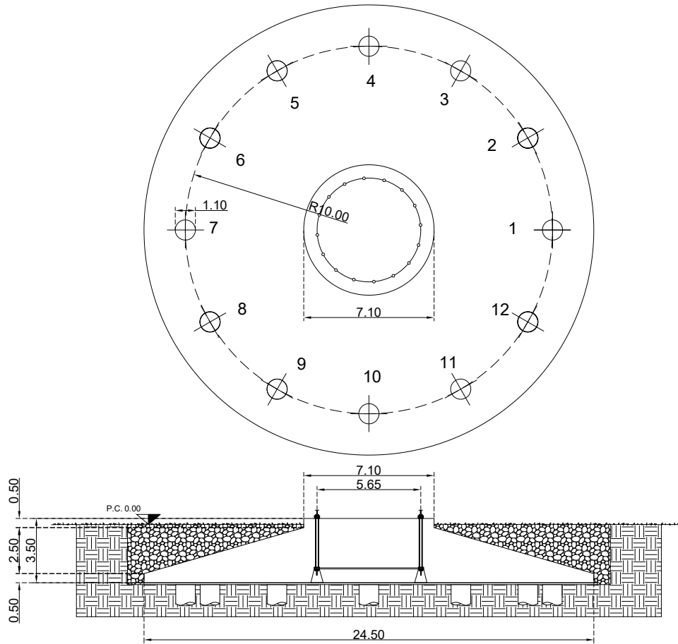
Figura 5.1.1: Dettaglio pianta e sezione fondazione
