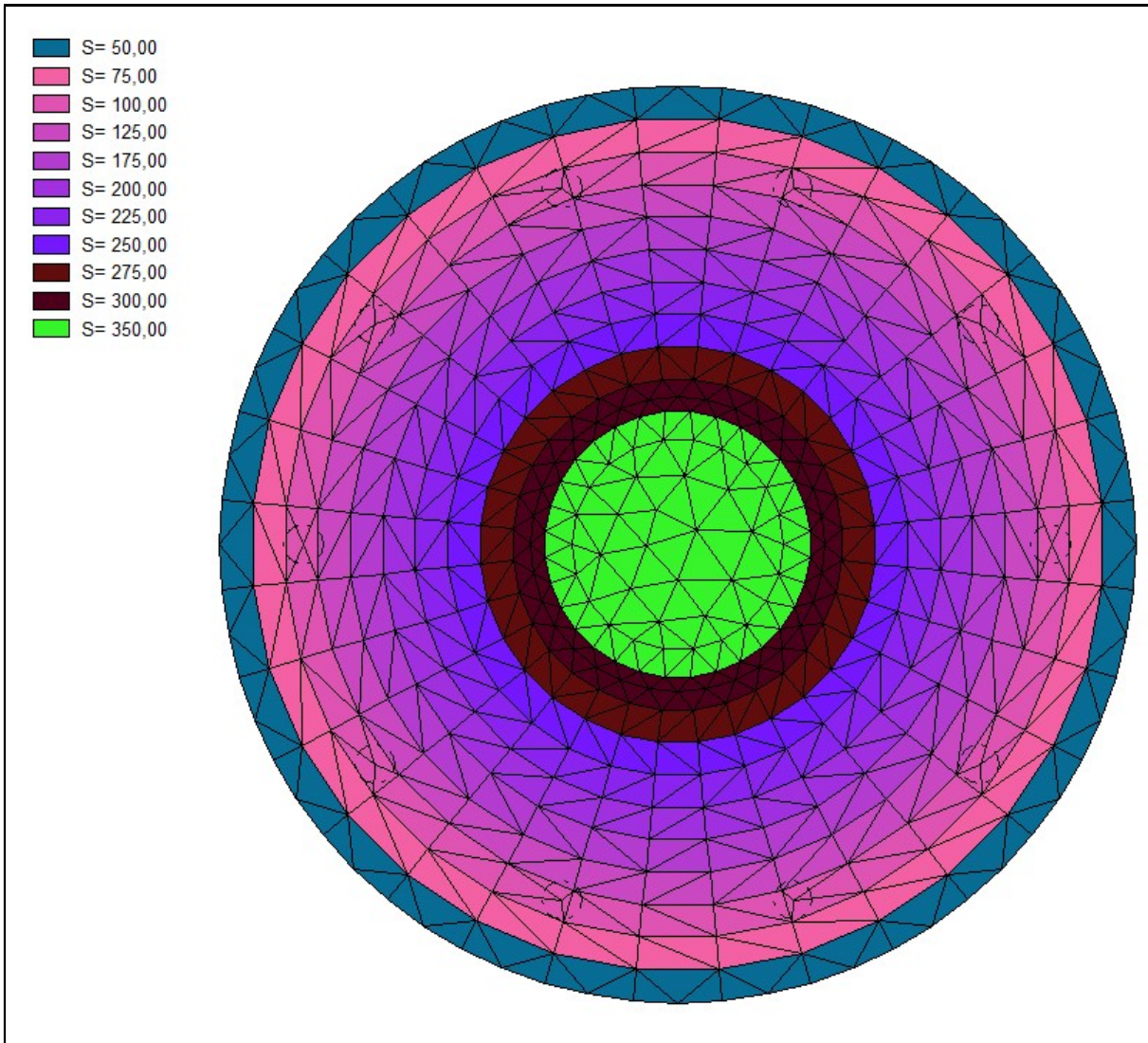
Figura 9.1.1: Spessori modellazione strutturale ( unità di misura cm )
