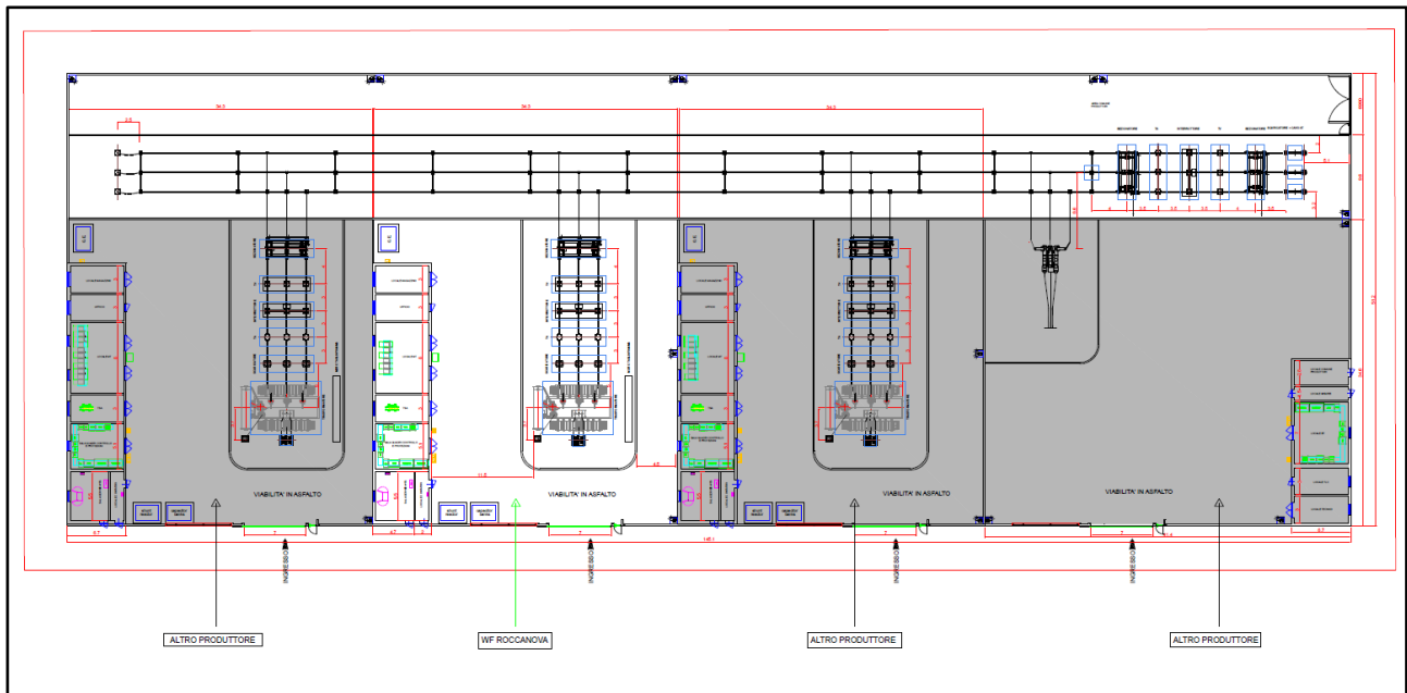
Figura 7.1: Planimetria elettromeccanica della Stazione di trasformazione 150/33 kV
