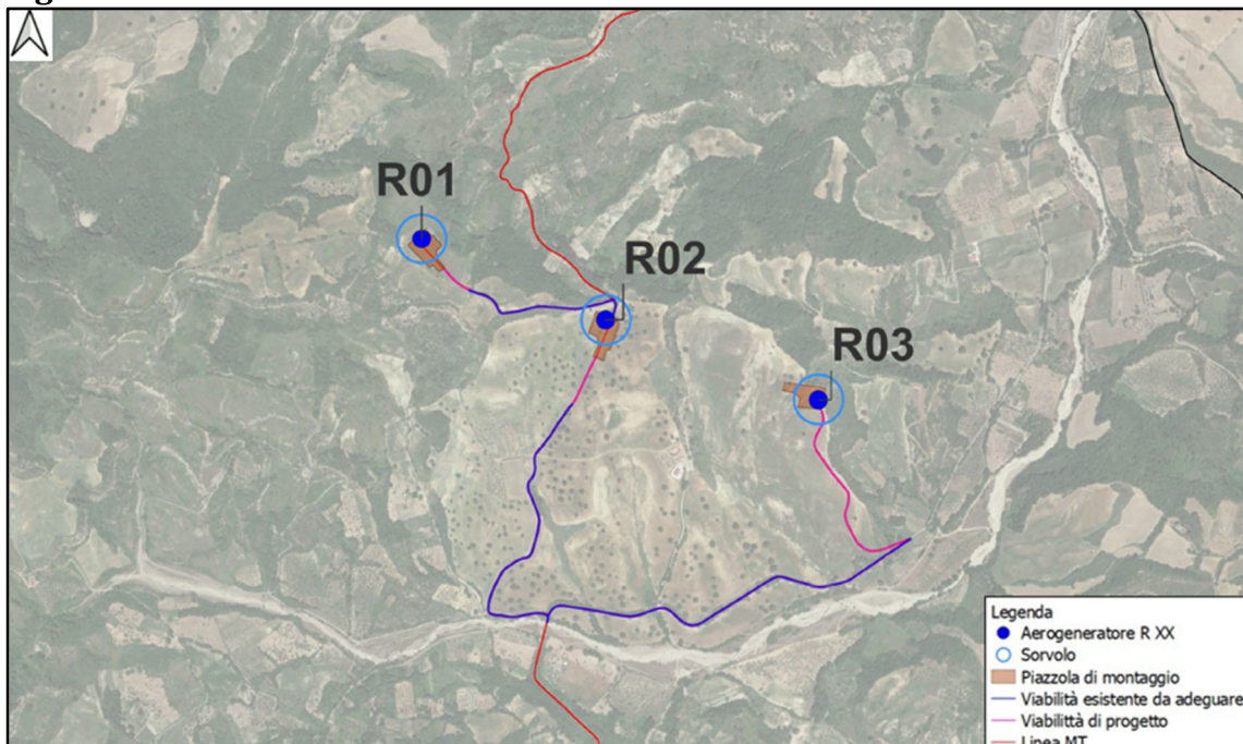
Figura 2.6: Parco Eolico Roccanova – Zona 1 su ortofoto
