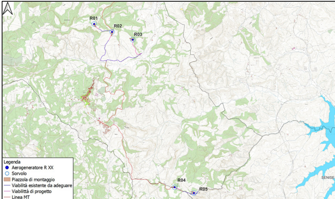
Figura 2.5: Parco Eolico Roccanova su CRT
