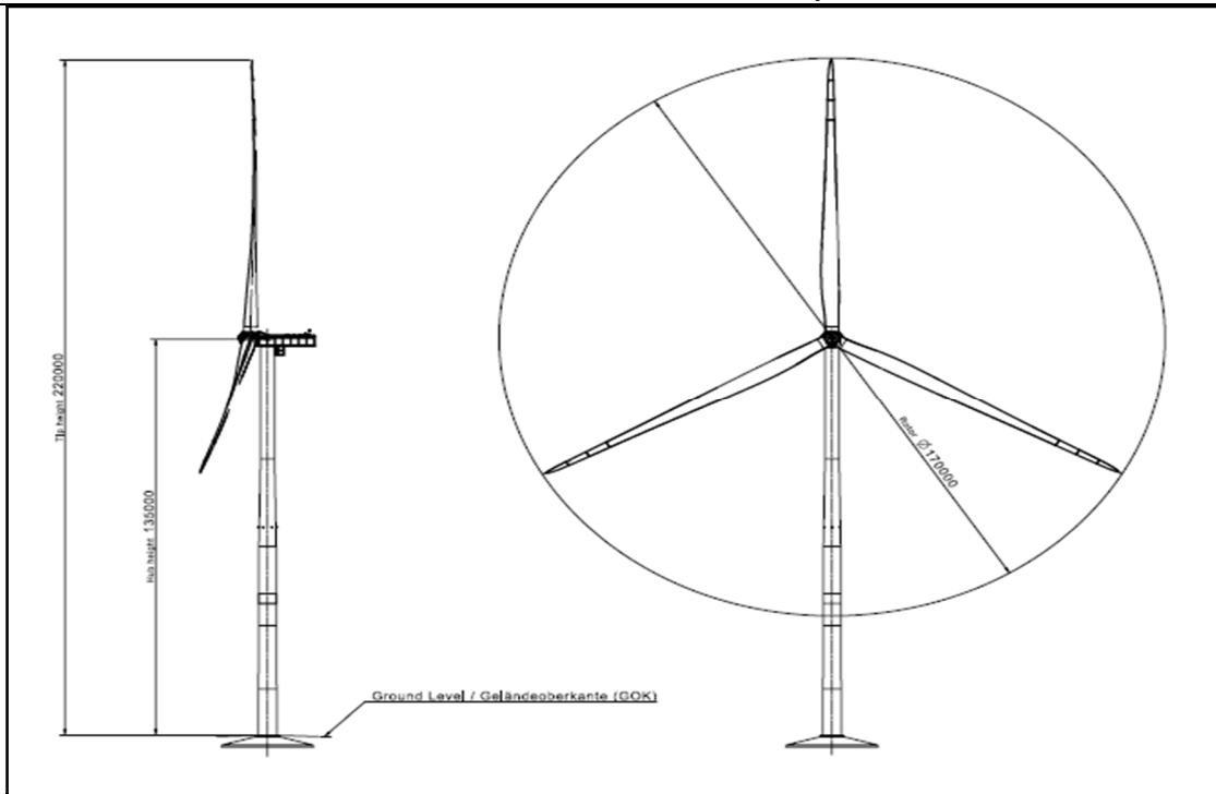
Figura 2.1.1: Profilo aerogeneratore SG170 HH135 – 6.2 MW
