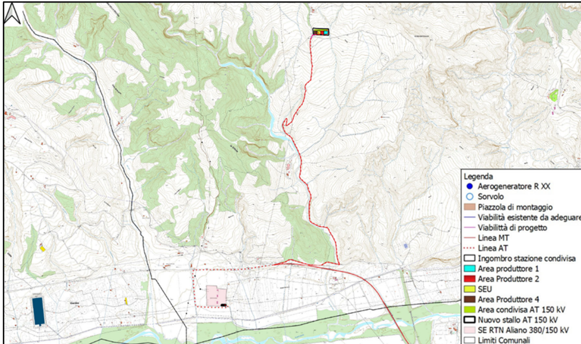
Figura 2.3: Area SEU 150/33 kV
