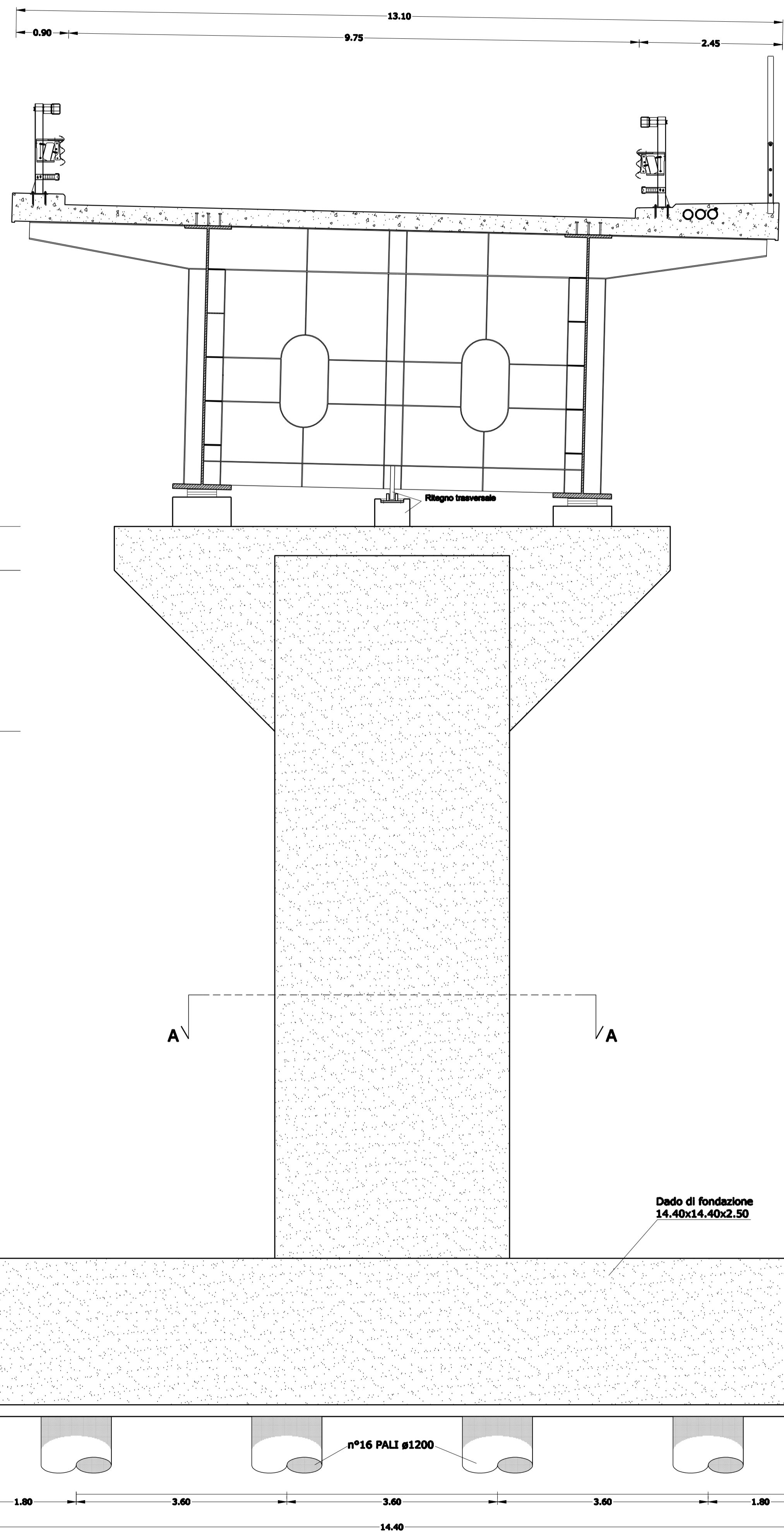
PROSPETTO PILA IN DIREZIONE LONGITUDINALE
