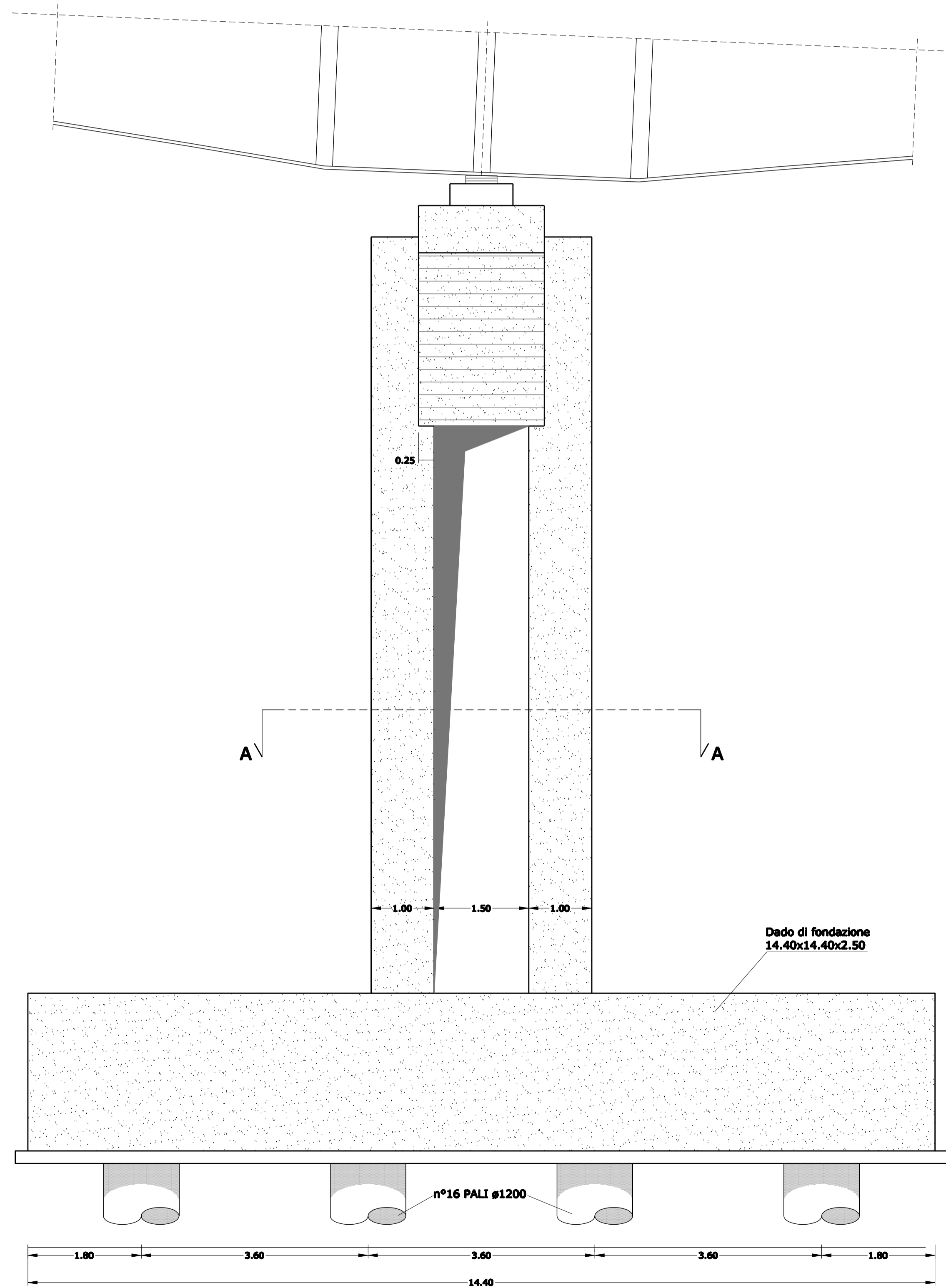
PROSPETTO PILA IN DIREZIONE TRASVERSALE
